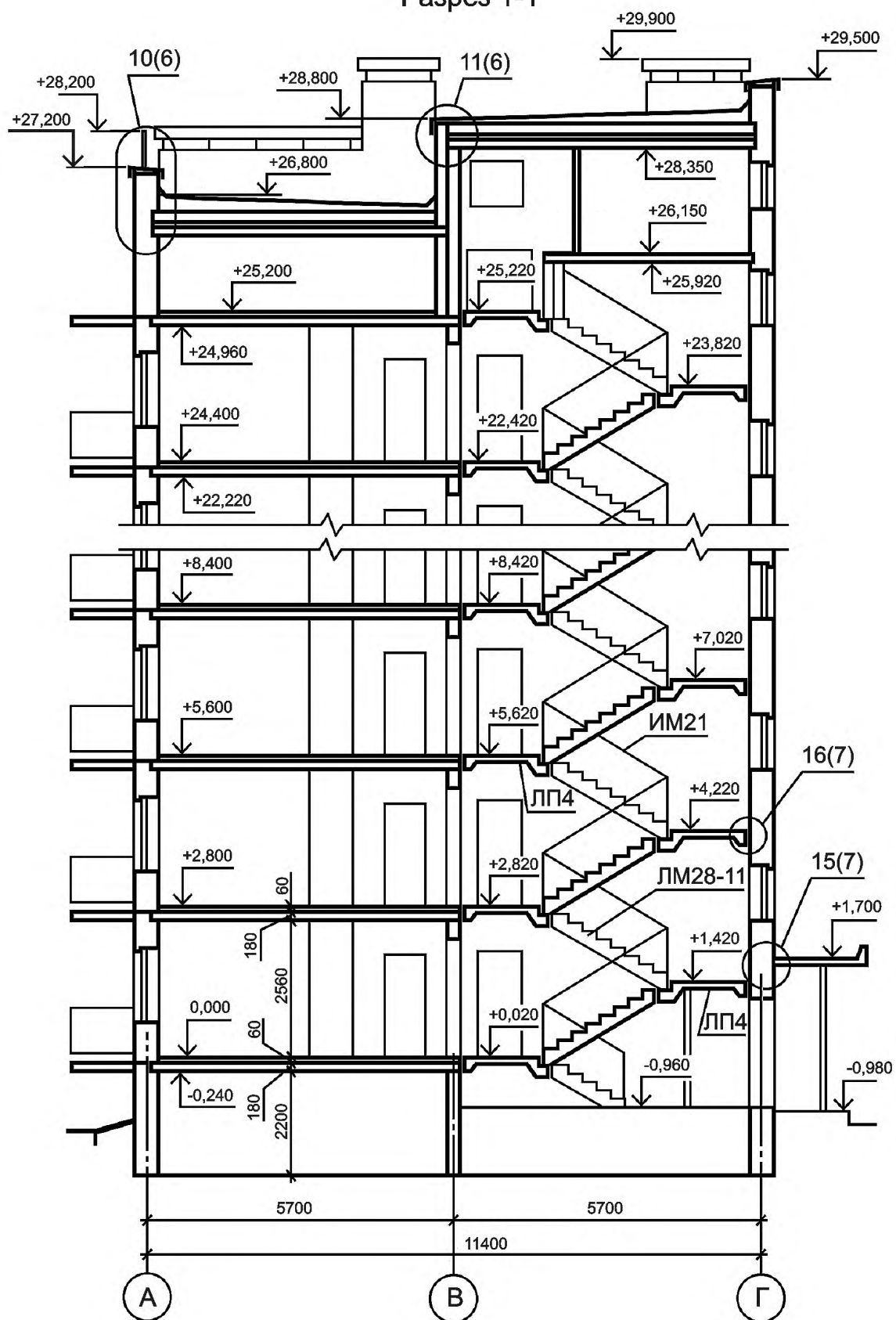
Рисунок Г.3 — Пример выполнения разреза жилого дома
