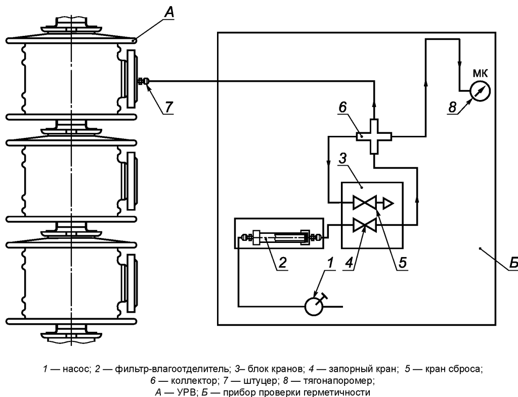
Рисунок 12.2 — Схема проверки герметичности УРВ
