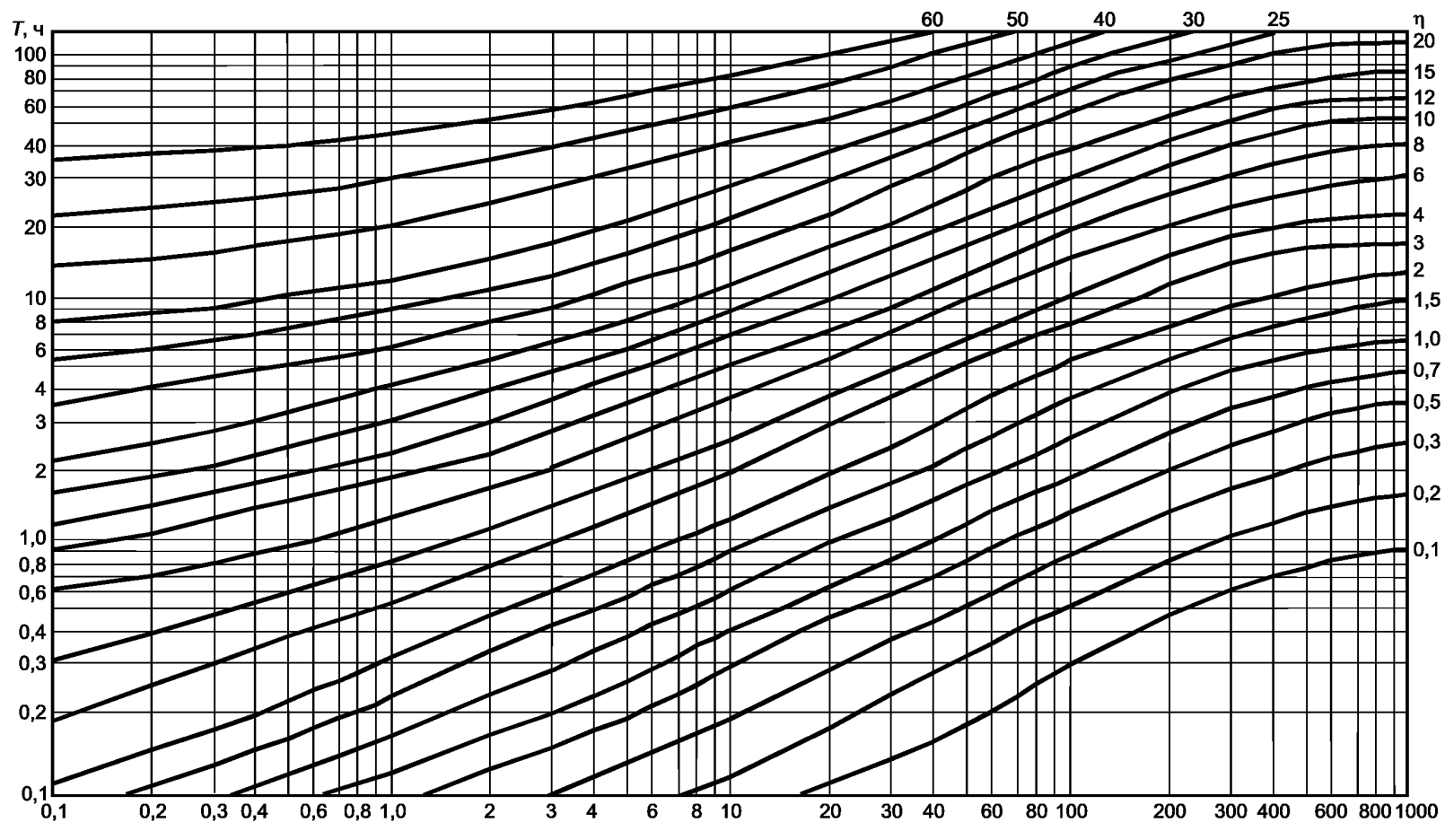
Рисунок 3 — Зависимость допустимого времени пребывания на загрязненной территории T , ч, от времени начала облучения t_n , ч, при различных значениях коэффициента \eta = \frac{D_d \cdot K_0}{P_{24}} ( D_d , сГр; P_{24} , сГр/ч). Вклад внутреннего облучения и \beta -облучения кожных покровов не учитывают
