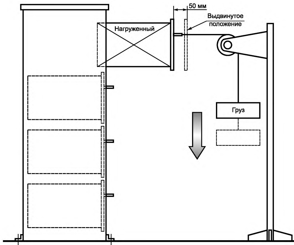
Рисунок 6 — Испытание на прочность крепления ящика картотеки
