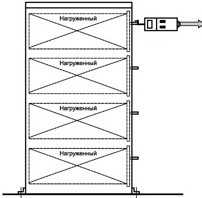
Рисунок 7 — Испытание картотек на прочность
