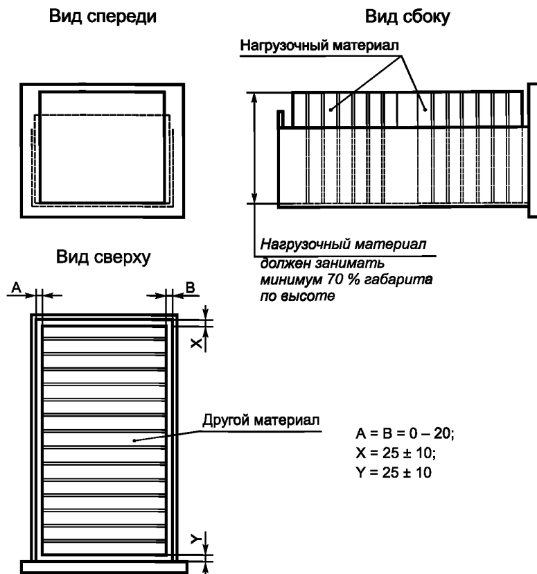
Рисунок 1 — Схема укладки выдвижных элементов
