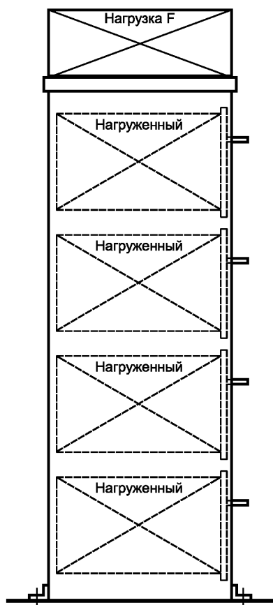
Рисунок 3 — Испытание картотек на прочность под нагрузкой
