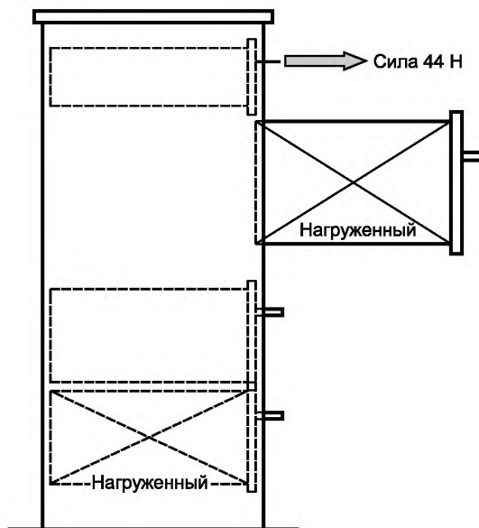
Рисунок 2 — Испытание картотек на устойчивость
