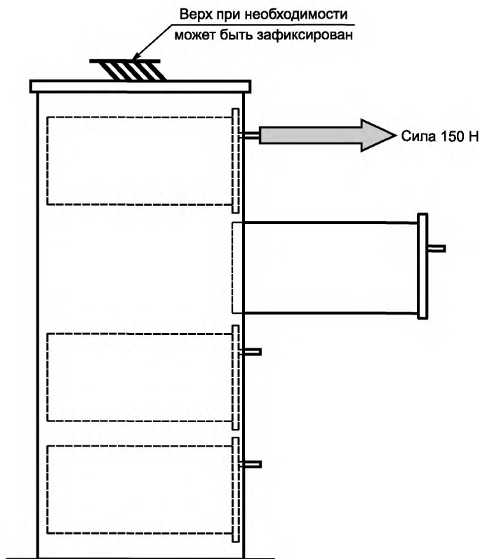
Рисунок 5 — Испытание на прочность блокирующего устройства
