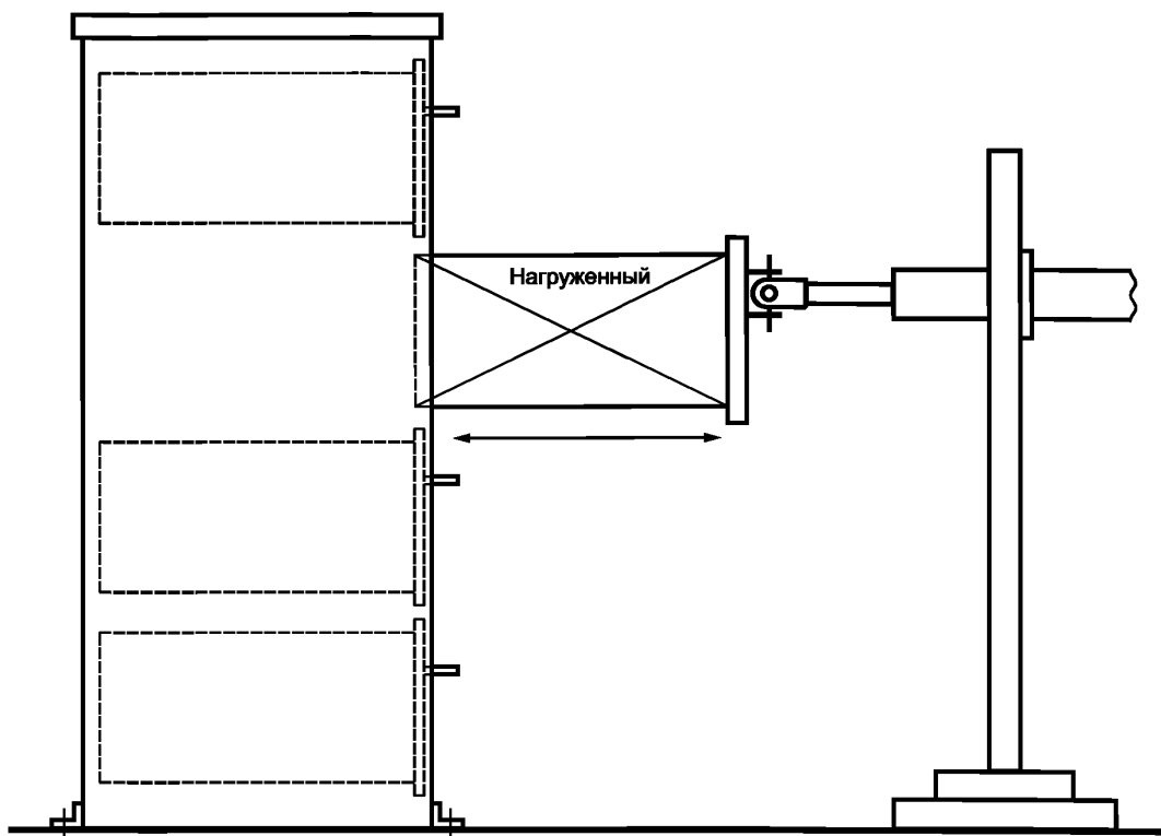
Рисунок 4 — Циклическое испытание раздвижного элемента
