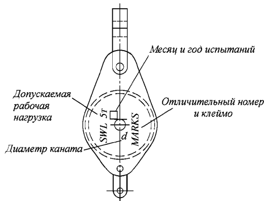
Рис. 11.2.1-5 Маркировка блока
