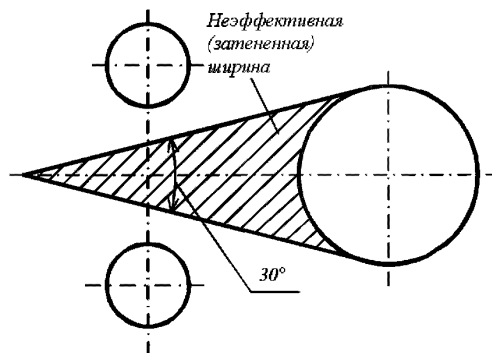
Рис. 1.4.8.3 Расчетное сечение
