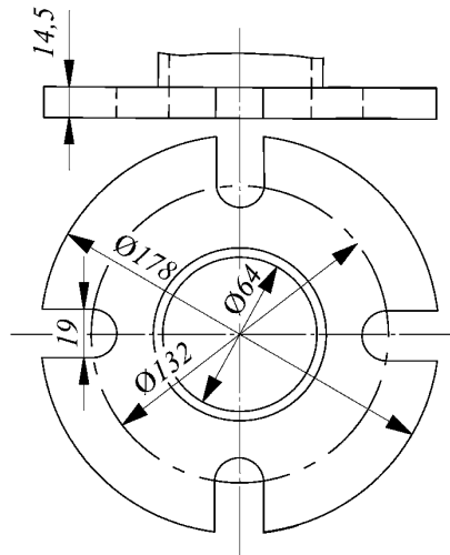
Рис. 5.1.18 Международное береговое соединение (судно)
