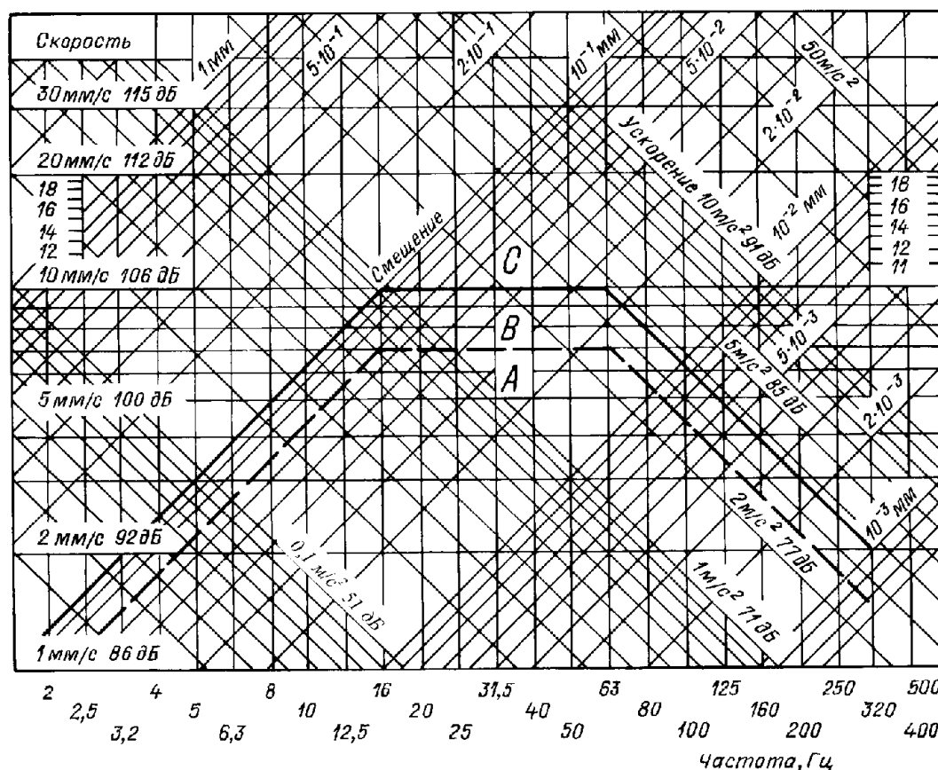
Рис. 9.7.1 Нормы вибрации котлов, вспомогательных механизмов и оборудования:
