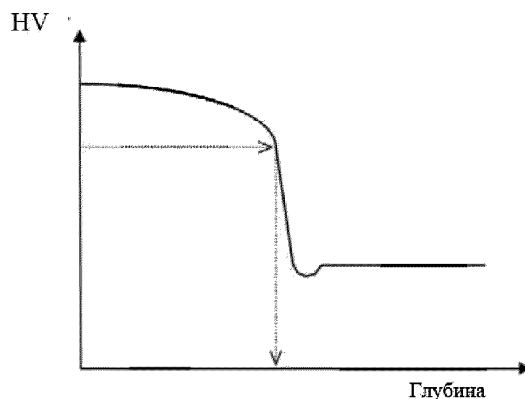
Рис. 4-1. Типовой график зависимости твердости от глубины. Стрелки указывают на глубину заковки
