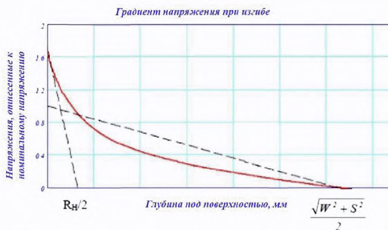
Рис. 3.1-1. ККН при изгибе в галтели шатунной шейки в зависимости от глубины. Соответствующий ККН для галтели рамовой шейки может быть определен путем замены R_H на R_G
