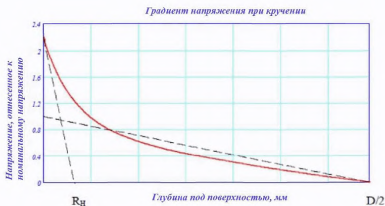
Рис. 3.1-2. ККН при кручении в галтели шатунной шейки в зависимости от глубины. Соответствующий ККН для галтели рамовой шейки может быть определен путем замены R_H на R_G и D на D_G
