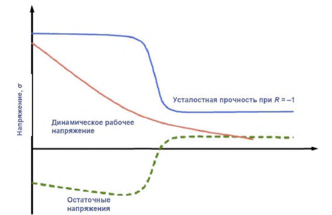
Рис. 3. Общие принципы зависимости напряжений от глубины
