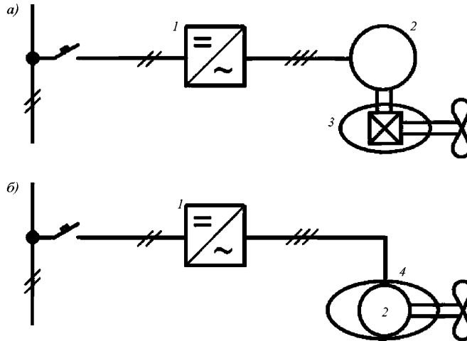
Рис. 3.2-4 Структурные схемы ГЭУ с винторулевыми колонками:
