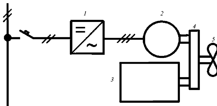
Рис. 3.2-3 Структурная схема вспомогательной ГЭУ с комбинированным пропульсивным комплексом:
