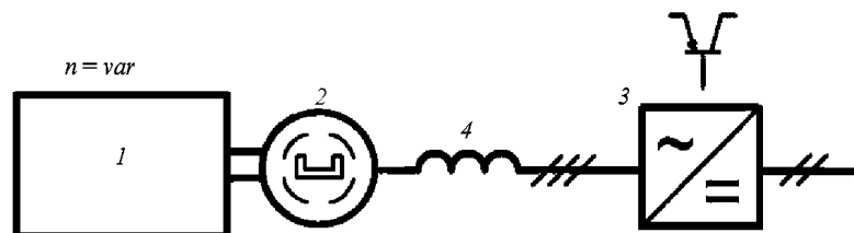
Рис. 3.1-4. Структурная схема вентильного генератора на базе активного выпрямителя
