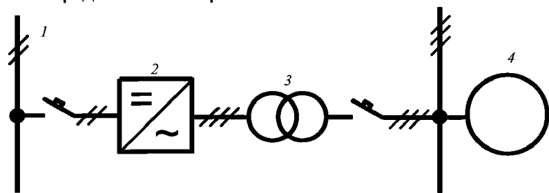
Рис. 3.3.1-4 Схема подключения эквивалентного электродвигателя в ЭЭС с полным распределением электроэнергии на постоянном токе:
