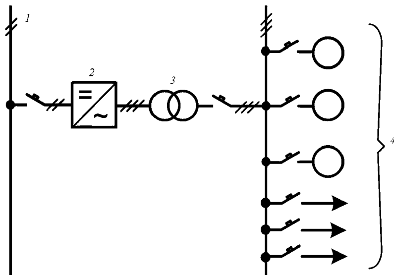
Рис. 3.3.1-3 Схема подключения общесудовой нагрузки переменного тока в ЭЭС с полным распределением электроэнергии на постоянном токе:
