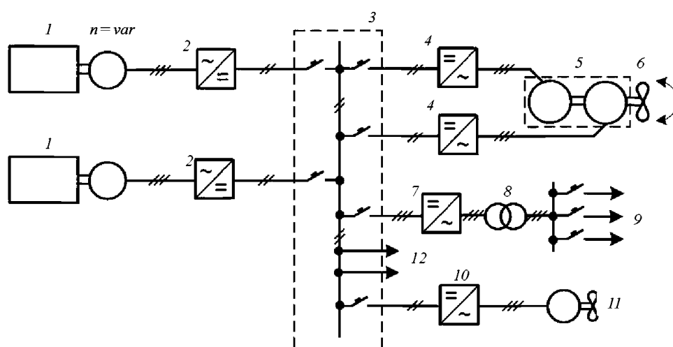
Рис. 2.2-2 Структурная схема ЭЭС с полным распределением вырабатываемой электроэнергии на постоянном токе с одновальной системой электродвижения и прямой передачей вращающего момента на винт:
