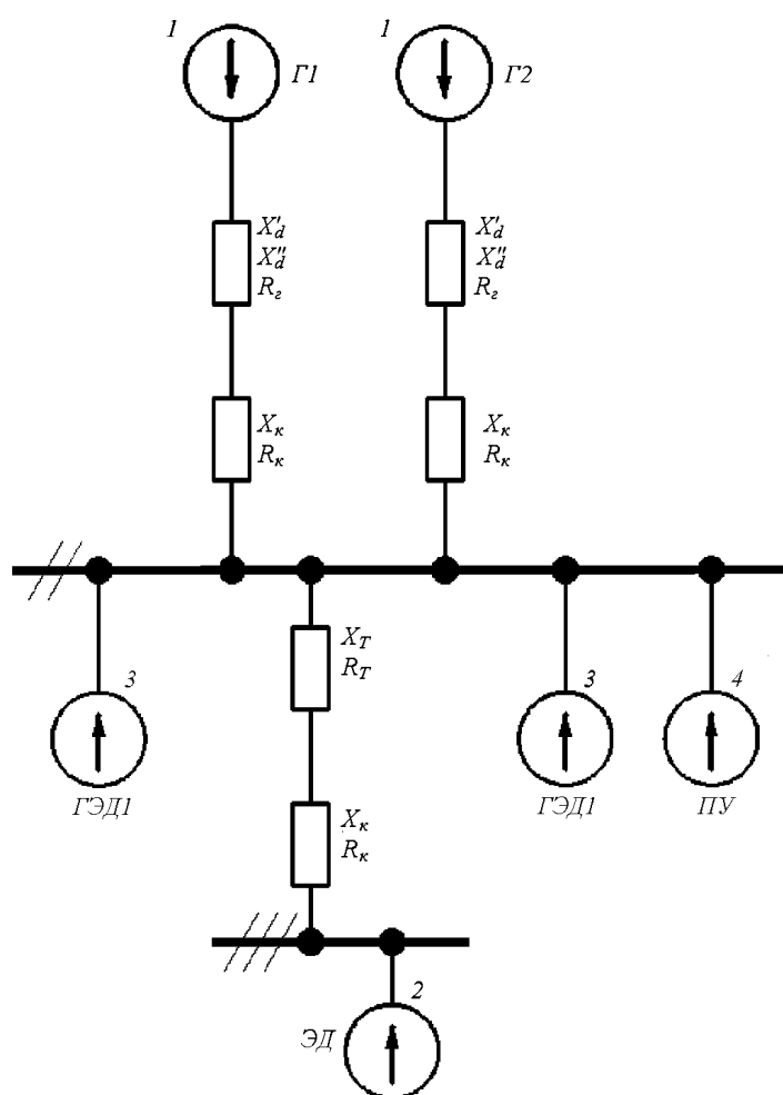
Рис. 7.2-1 Расчетная схема замещения ЭЭС с полным распределением вырабатываемой электроэнергии на постоянном токе с асинхронными гребными двигателями:
