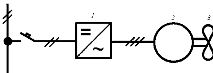
Рис. 3.2-2 Структурная схема ГЭУ с прямой передачей вращающего момента на винт:
