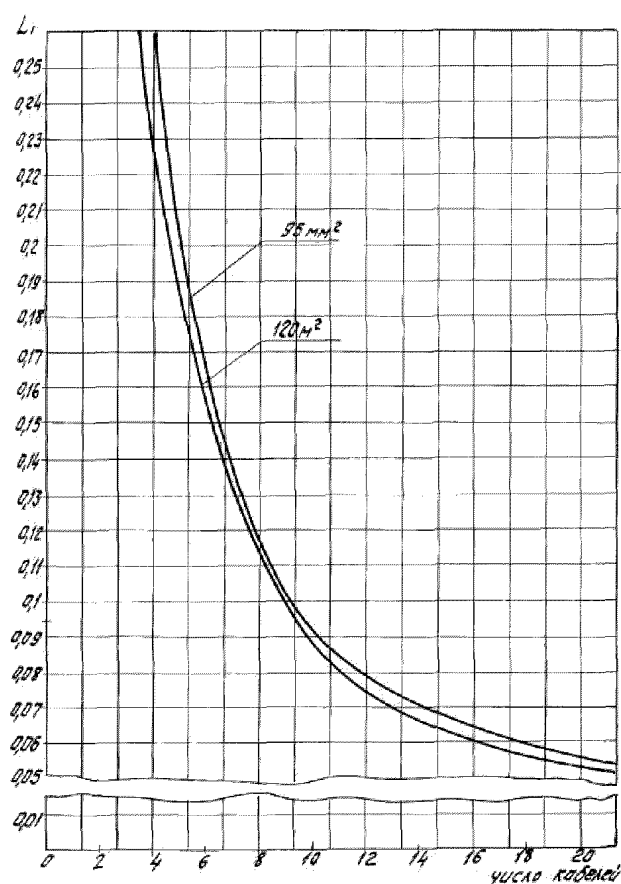
Рис. 8.6-4 Кривые для определения удельной индуктивности кабельной трассы в зависимости от числа кабелей и сечения токопроводящей жилы кабеля марок КВД-60, КВД-100 и КРНГ-60, \text{Г/м} \cdot 10^{-6}
