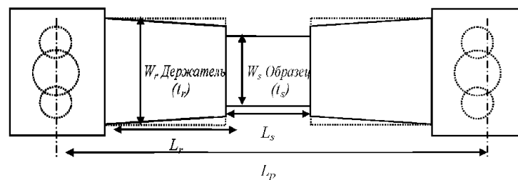
Рис. 3.20.6.2 Схема расположения испытываемого образца, держателя и оснастки
