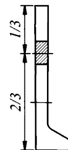
Рис. 3.2.5-4 Полособульб
