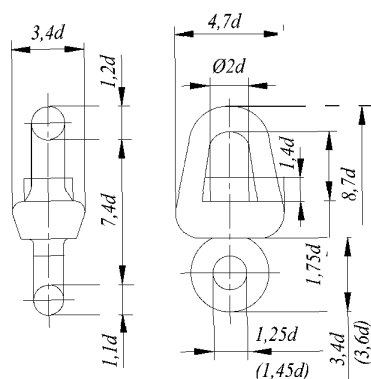
Рис. 7.1.3-7 Вертлюг
