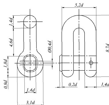
Рис. 7.1.3-6 Концевая скоба
