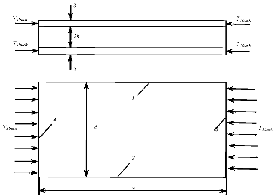
Рис. 30 Вид нагружения прямоугольной трехслойной пластины
