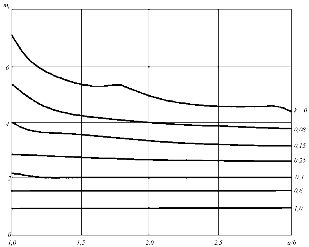
Рис. 35 График зависимости коэффициента m_l от соотношения сторон пластины a/b , если кромки 1, 2 — шарнирно оперты; кромки 3, 4 — защемлены
