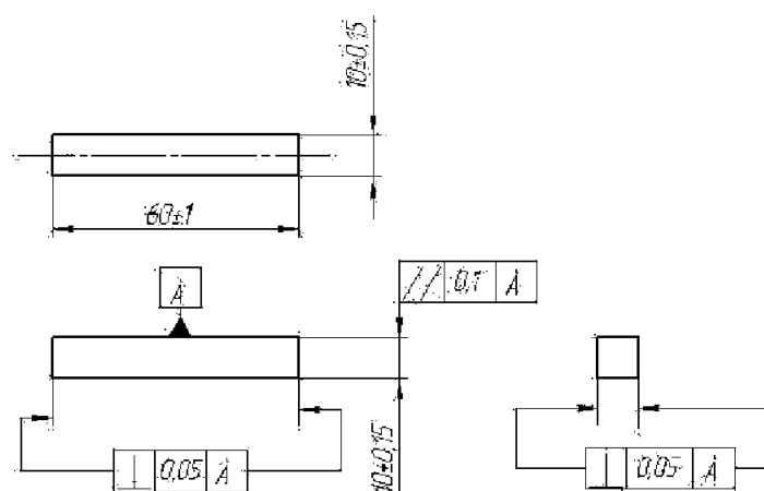
Испытания на межслойный сдвиг Призма 60 \times 10 \times 10 мм
