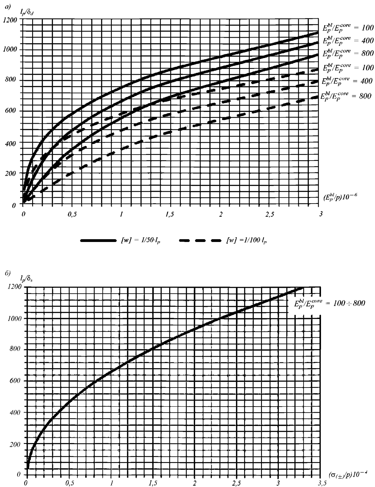
Рис. 3.9 Графики зависимости отношения максимальной длины l_p , м, опорного контура трехслойной пластины к толщине ее несущих слоев \delta_d , ( \delta_s ), м, от отношения свойств материала несущих слоев E_p^{bl} , \sigma_{(\pm)}^{bl} , МПа, пластины к расчетному давлению p (при 2h=10\delta ):
