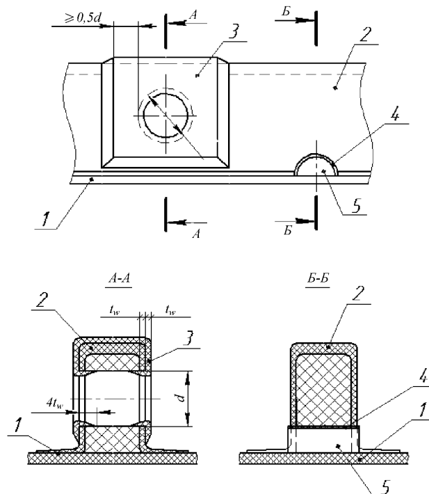
Рис. 3.27 Подкрепление вырезов в балках набора П-образного профиля: 1 — обшивка (настил палубы, платформы); 2 — балка; 3 — накладка; 4 — оформитель выреза; 5 — водопроток (шпигат)
