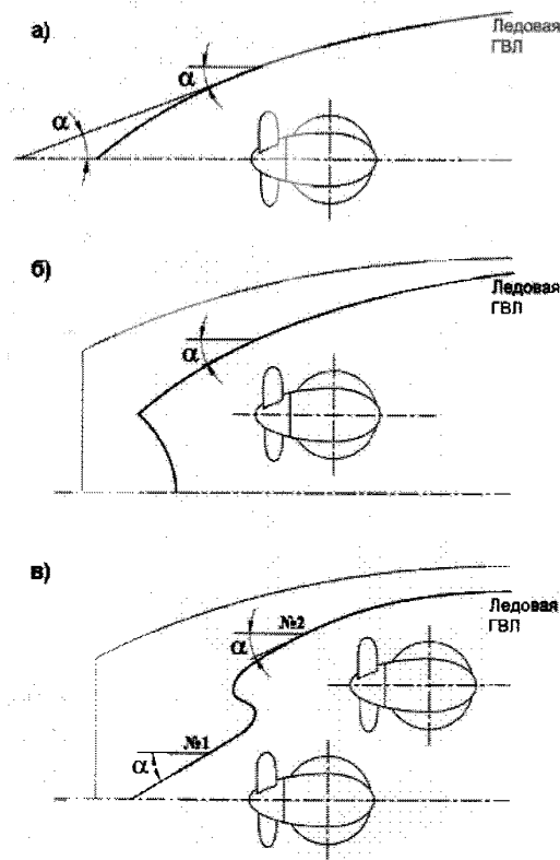
Рис. 19.2.4.1 Определение углов наклона ватерлинии в кормовой оконечности:
