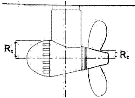
Рис. 10.7.6.5.2 Определение R_c
