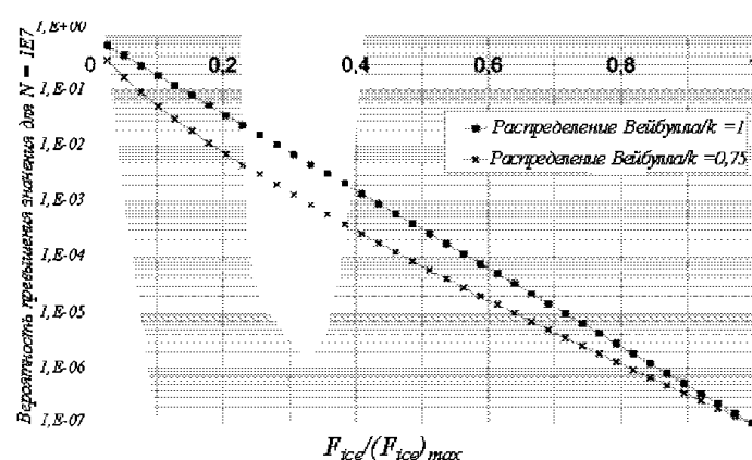
Рис. 10.7.5.1.8 Распределение Вейбулла
