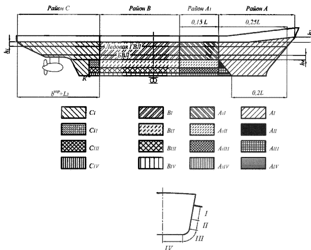
Рис. 19.2.2.3 Районы ледовых усиления арктических судов двойного действия, имеющих в символе класса знак ледового класса Icebreaker6 или Icebreaker7 при движении кормой вперед:
