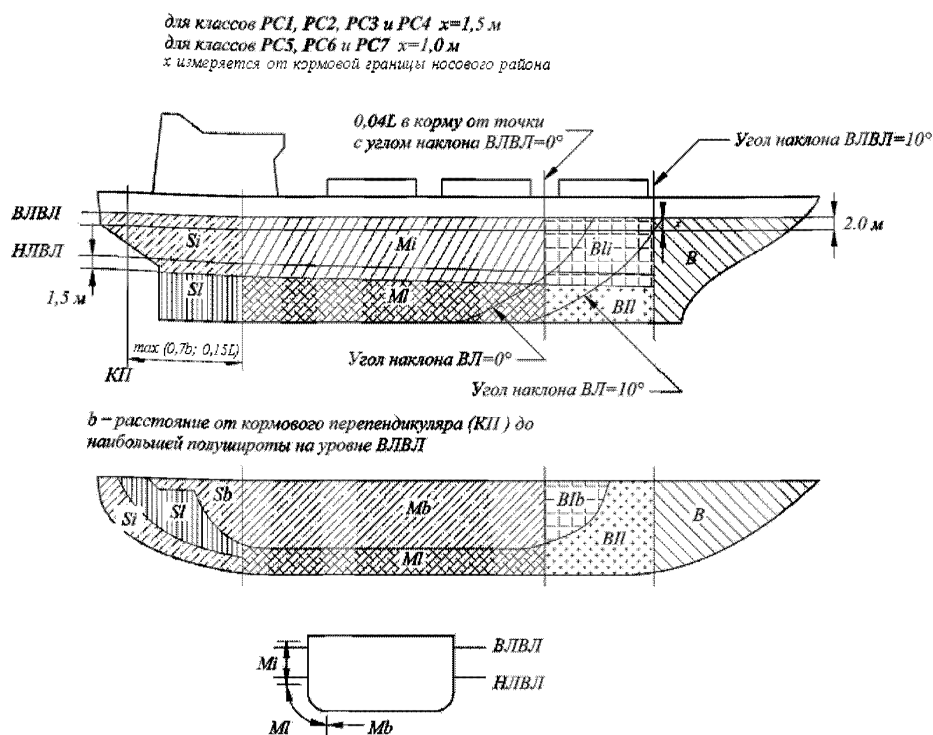
Рис. 1.2.2.1 Границы районов корпуса судна
