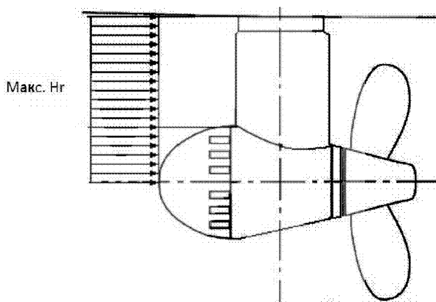
Рис. 10.7.6.5.3 Определение зоны контакта при преодолении тороса
