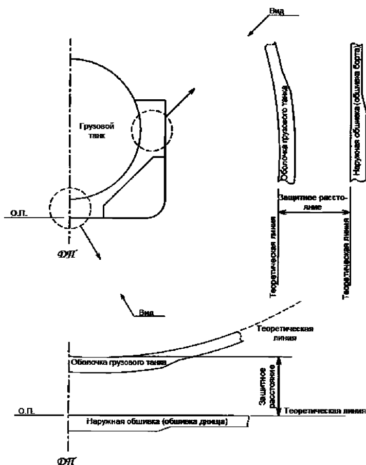
Рис. 2.5-5 Защитное расстояние для напорной грузовой емкости
