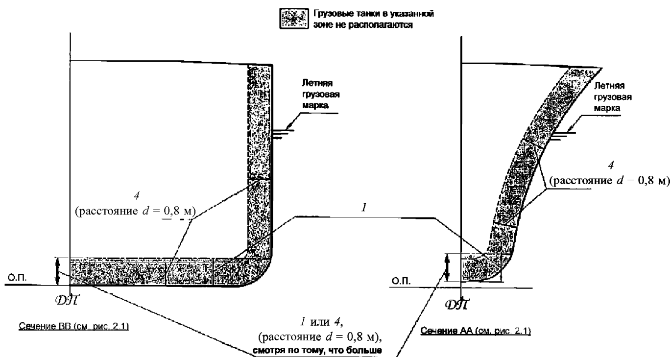
Поперечные сечения – суда типа 3G
