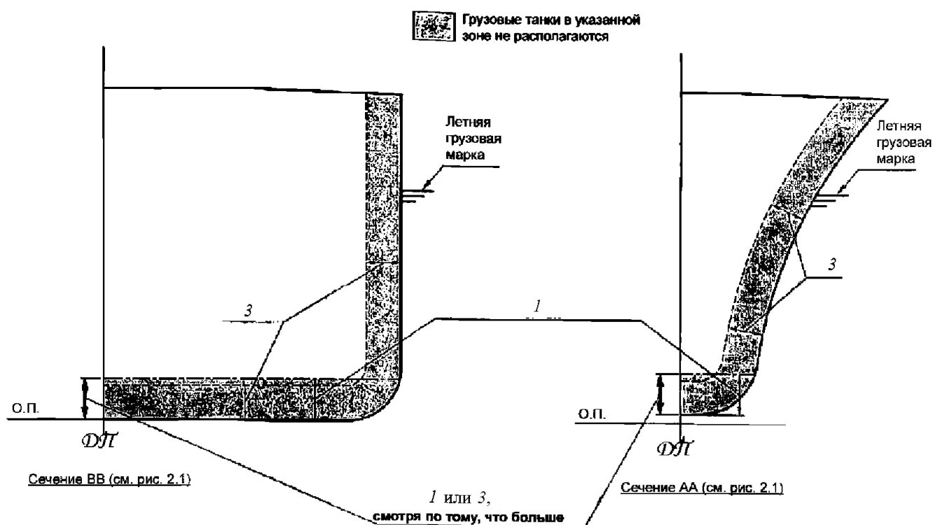
Поперечные сечения – суда типов 2G и 2PG
