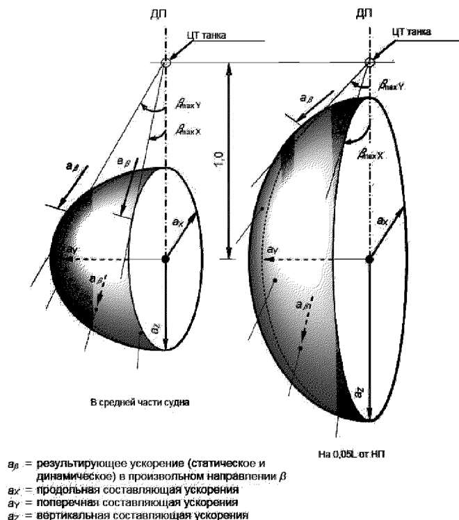
Рис. 28.1.2-1 Эллипсоид ускорений
