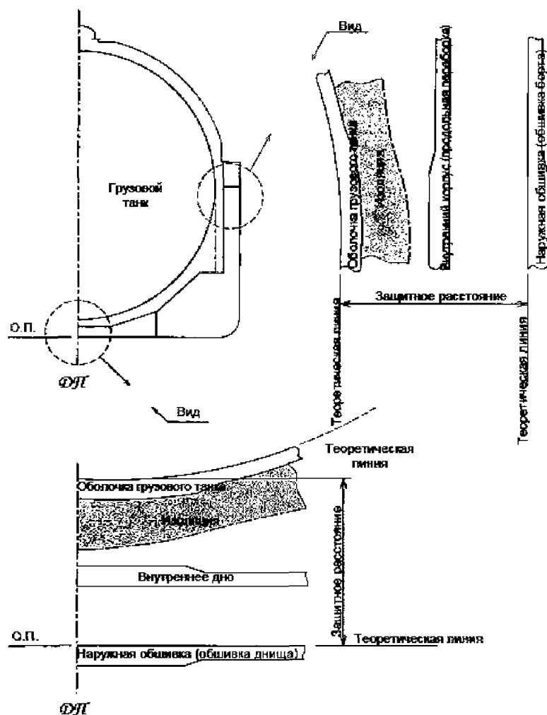
Рис. 2.5-4 Защитное расстояние для сферической грузовой емкости
