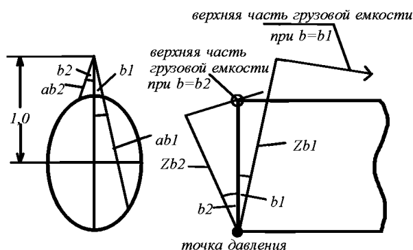
Рис. 23.1.4 Схема для определения разницы динамического давления
