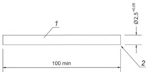
1 — испытательный стержень (металлический); 2 — прямоугольные острые края
