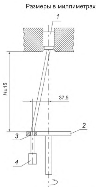
1 — зажим; 2 — плита; 3 — втулка 1) ; 4 — груз
