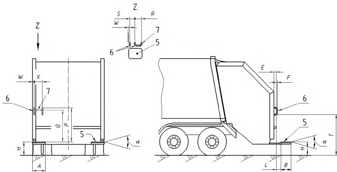
Рисунок В.4-1а — Езда на подножках. Подножка (и) и поручни. Ситуация I
