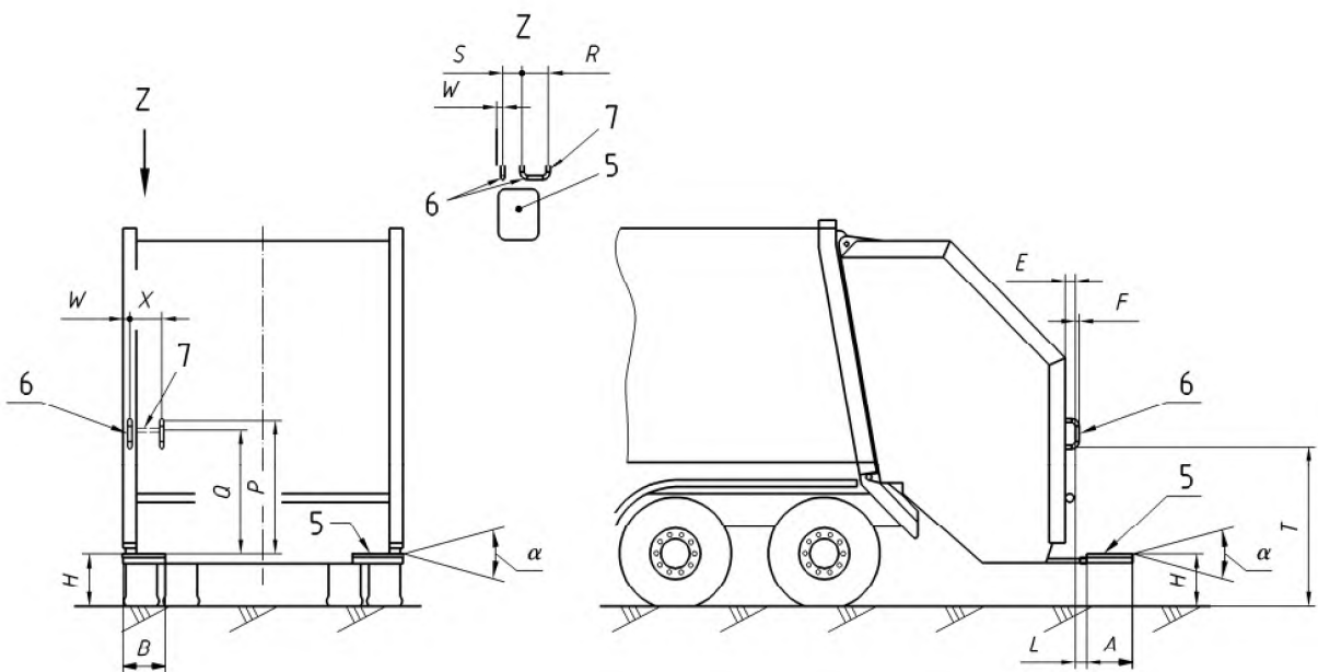
Рисунок В.4-1b — Езда на подножках. Подножка (и) и поручни. Ситуация II
