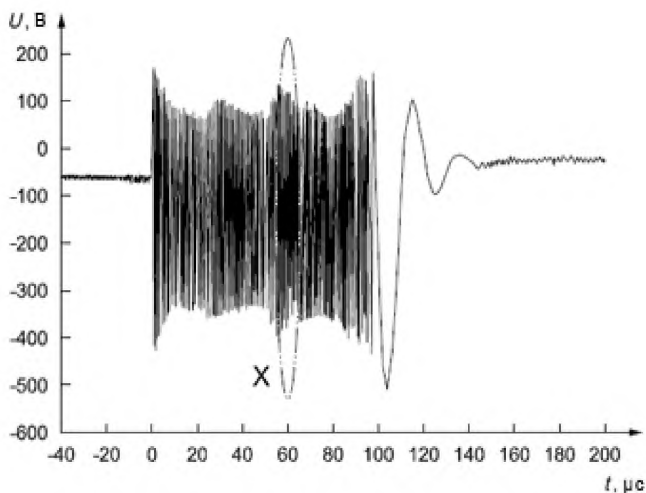
а) Пример сложной формы сигнала A2
