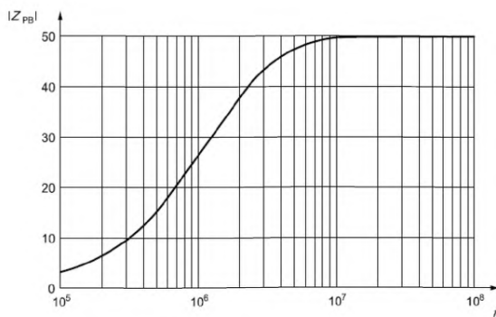
Рисунок 4 – Полное сопротивление |Z_{PB}| как функция частоты от 100 кГц до 100 МГц (АВ замкнуты накоротко)
