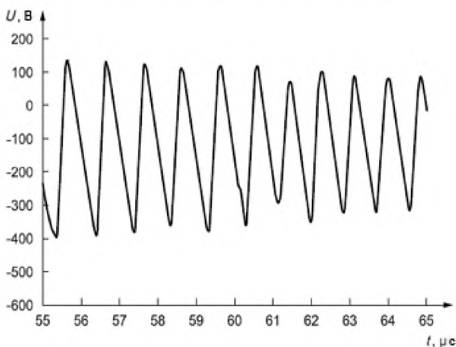
б) Пример формы сигнала A2 (подробный)
