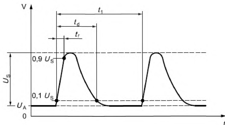
Рисунок 6 – Испытательный импульс 2а
