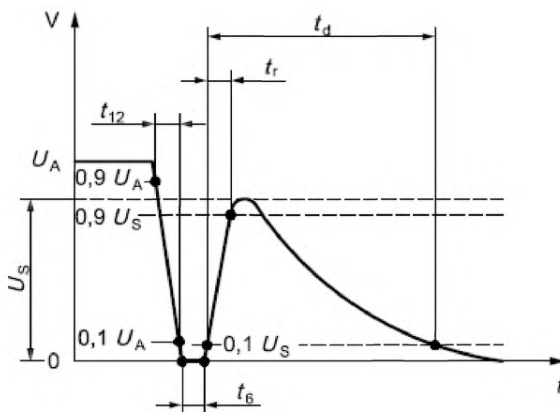
Рисунок 7 – Испытательный импульс 2b
