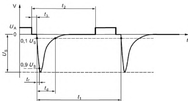
Рисунок 5 – Испытательный импульс 1
