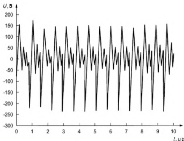
Рисунок F.8 – Пример характеристик формы сигнала С
