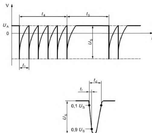
Рисунок 8 – Испытательный импульс 3а
