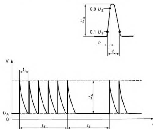
Рисунок 9 – Испытательный импульс 3б
