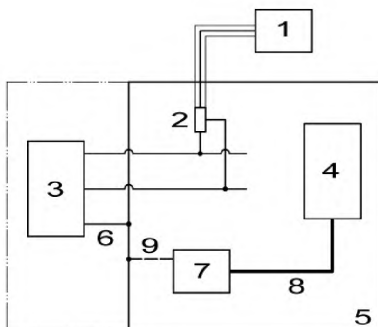
а) Коррекция импульсов
