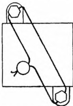
Рисунок 8 – Принципиальная схема пломбирования промежуточного штеккерного разъема электромеханического спидометра
