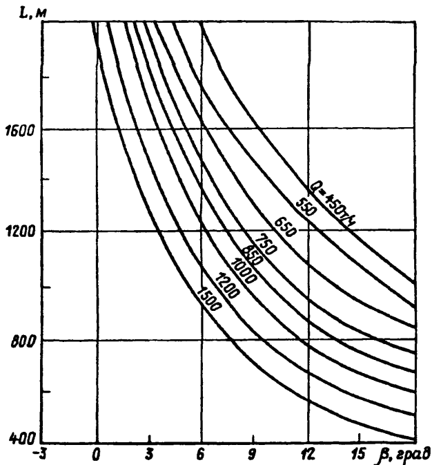
Рис. П246. Зависимость длины L конвейеров 2ЛУ120А и 2ЛУ120В от активационной нагрузки Q и угла установки \beta при мощности привода N_{\text{сум}} = 1000 кВт и скорости ленты 3,15 м/с
