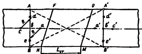
Рис. П.9.1. Схема разметки и центрирования концов ленты
