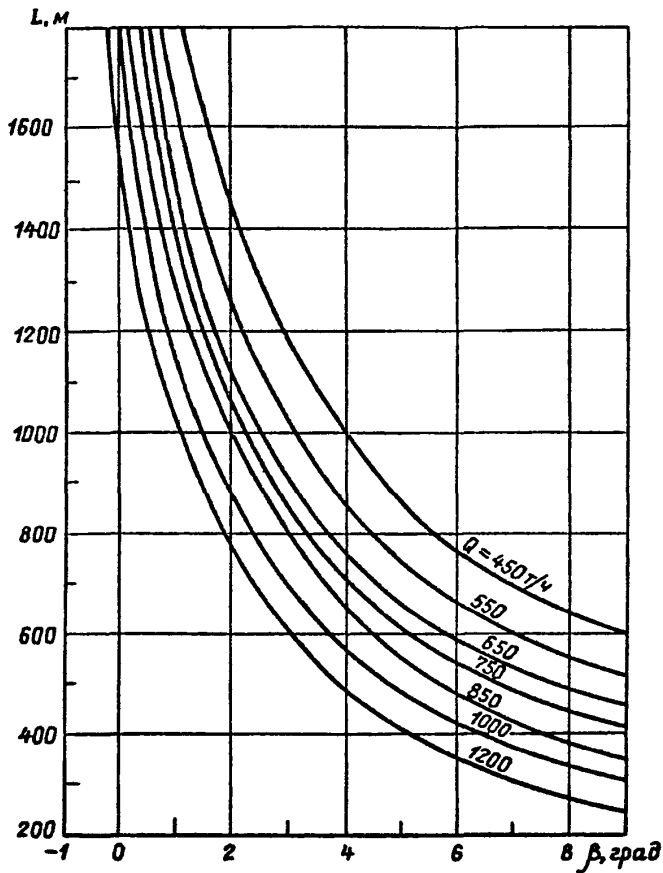
Рис. П2.40. Зависимость длины L конвейера ЛГУ120 от эксплуатационной нагрузки Q и угла установки \beta при мощности привода N = 500 кВт и скорости ленты 2,5 м/с
