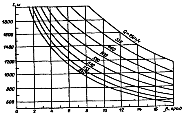
Рис. П.2.34. Зависимость длины L конвейера 3Л11000А-01 от эксплуатационной нагрузки Q и угла установки \beta при мощности привода N = 750 кВт и скорости ленты 2,5 м/с (лента резиновая ЗРЛГТВ(П)-2500)
