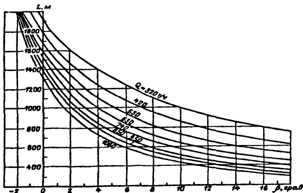
Рис. П.2.33. Зависимость длины L конвейера 3Л11000А от эксплуатационной нагрузки Q и угла установки \beta при мощности привода N = 500 кВт и скорости ленты - 3,15 м/с (лента резиновая ЗРЛГТВ(П)-2500)
