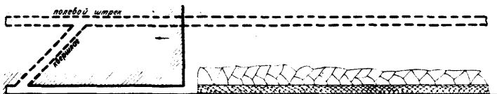
Рис.37. Схемы полевой подготовки защитных пластов (первого слоя)
