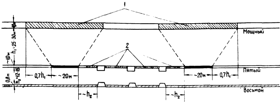
Рис.38. Схема возможного расположения уклонов по пластам Пятому и Восьмому для условий шахт № 30 и 32: 1-районы повышенных напряжений на пласте Мощном; 2-бутовые полосы
