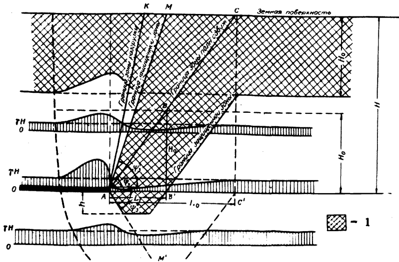
Рис. 3. Схема построения защищенной зоны на разрезе по простираанию пласта 1 - защищенная зона
