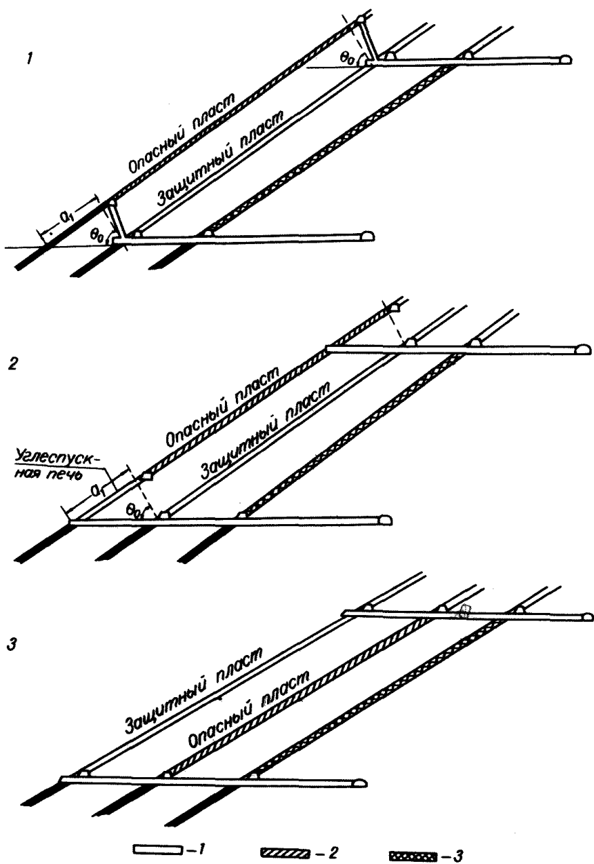
Рис. 19. Схемы подготовки и порядка обработки свиты пластов пологого и наклонного падения 1,2,3- порядок обработки пластов
