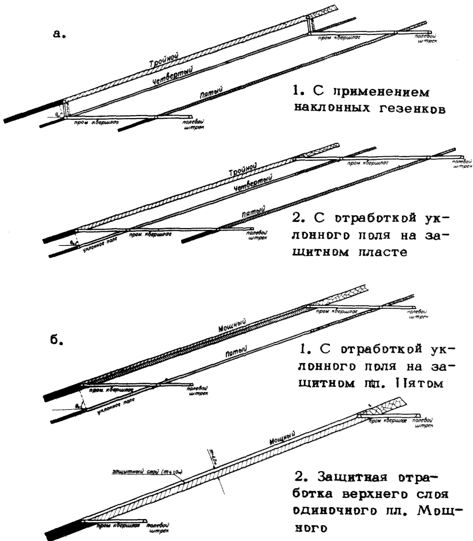
Рис. 33. Порядок отработки и схема подготовки по шахтам Воркутского месторождения
