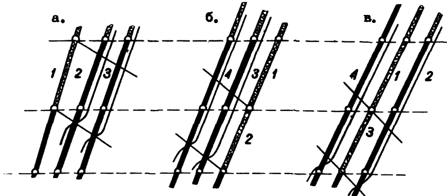
Рис.8. Рекомендуемый порядок отработки пластов: а-нисходящий порядок отработки на одном горизонте; б-восходящий порядок отработки на двух горизонтах; в-смешанный порядок отработки на двух горизонтах; 1,2,3,4 - порядок отработки пластов
