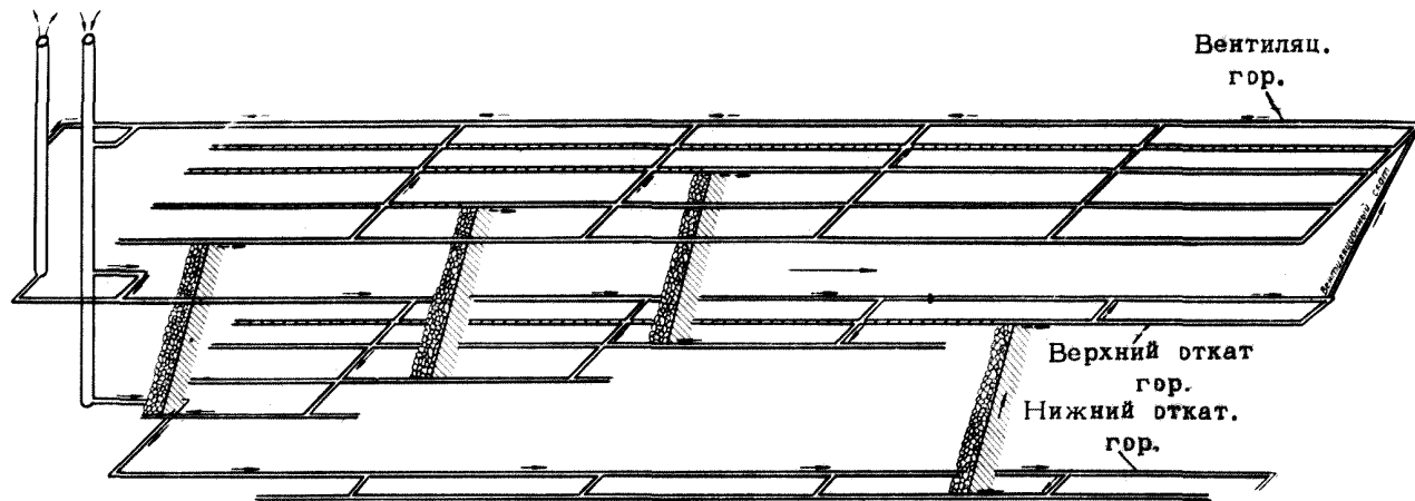
Рис. 14. Схема отработки пластов в пределах двух этажей
