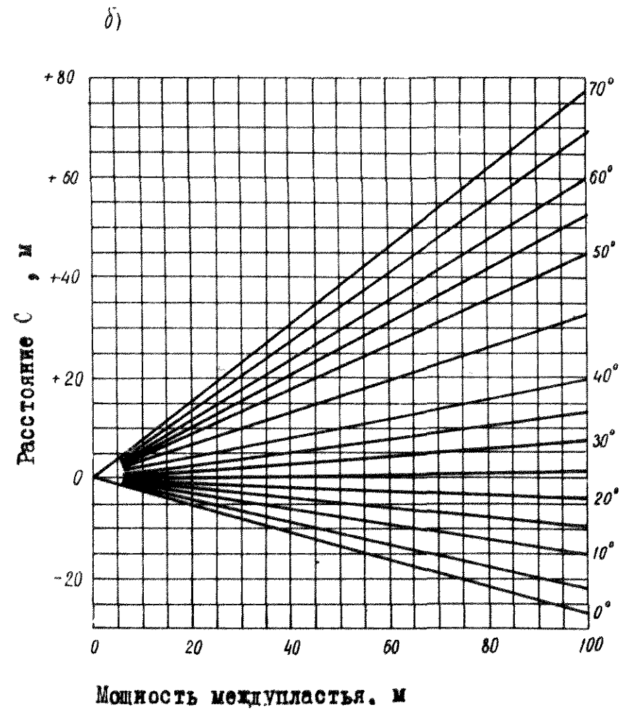
Рис. 2. Расстояние от границ очистных работ на защитном пласте до границ защищенной зоны на опасном пласте на совмещенном плане горных работ
