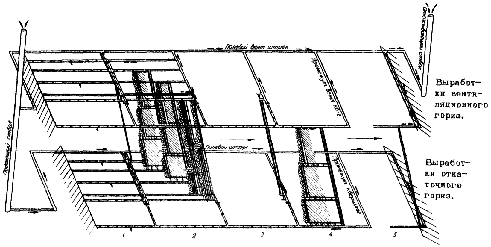
Рис. 28. Последовательная разработка выемочных участков от ствола к границам шахтного поля
