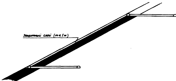
Рис.22. Схема подготовки и отработки мощных пластов пологого и наклонного падения, опасных и угрожаемых по горным ударам, с опережающей надработкой защитным слоем
