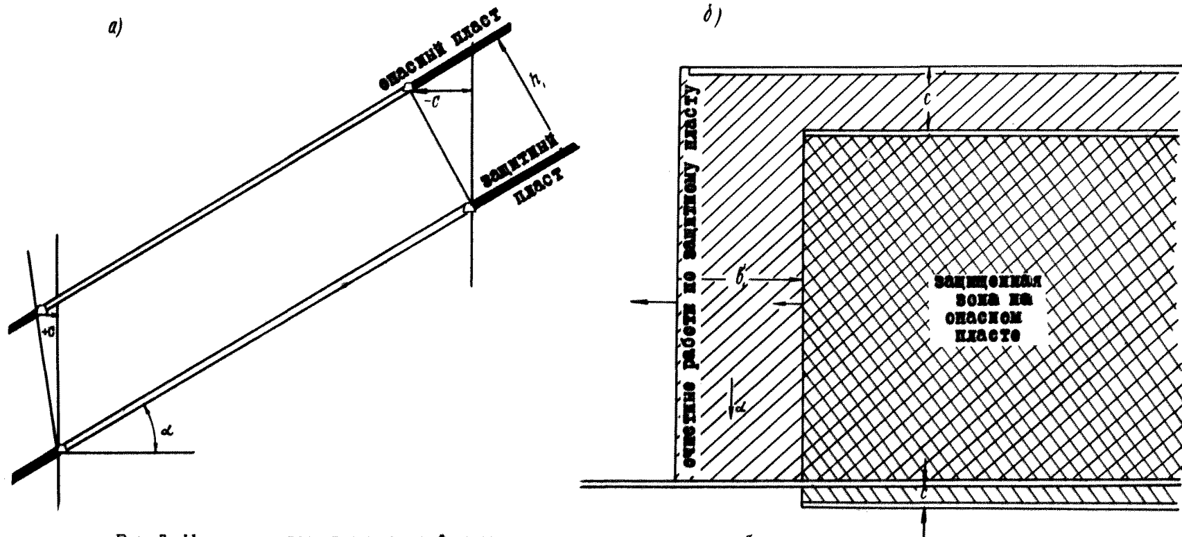
Рис. 5. Пример построения защищенной зоны на опасном пласте при подработке при \alpha = 30^\circ и мощности междупластья 60 м.
