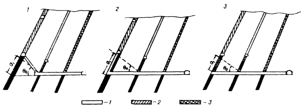
Рис.18. Схемы подготовки к выемке свиты крутых пластов: 1,2,3 - порядок отработки пластов
