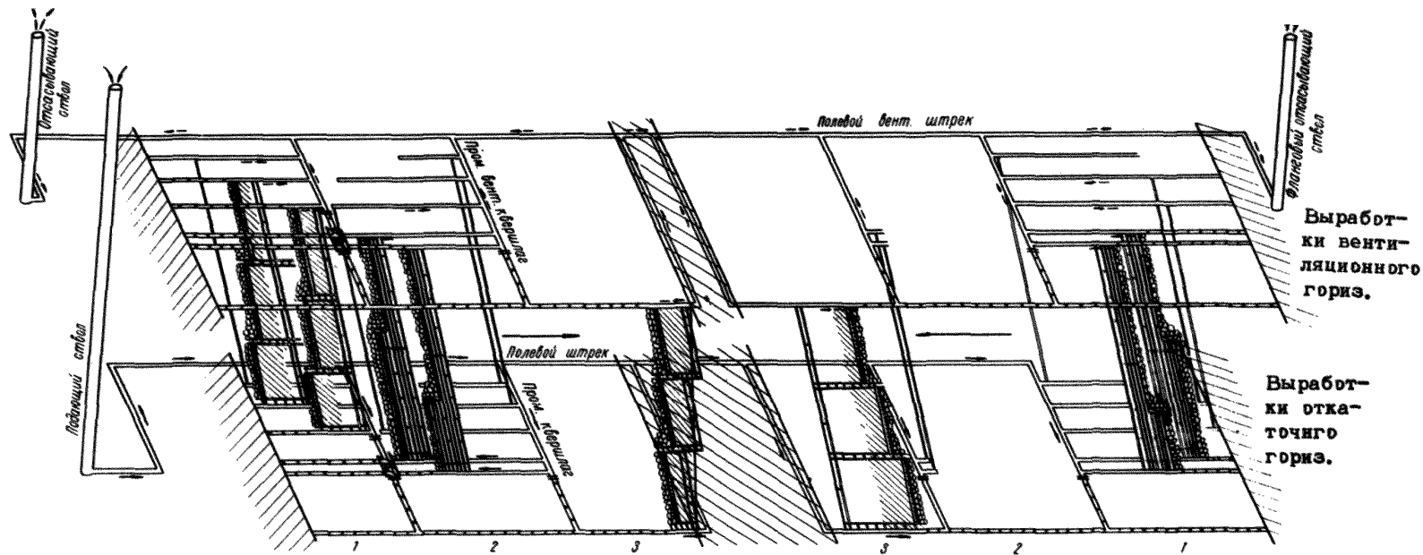
Рис. 29. Последовательная разработка выемочных участков от середины к границам шахтного поля
