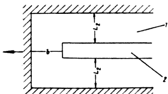
Рис.6. Появление опасных нагрузок в середине выработанного пространства по защитному пласти при ведении работ с щелками у вентиляционного горизонта: 1-защищенная зона; 2-зона восстановления опасных нагрузок
