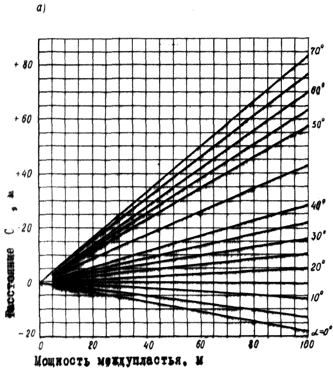
Рис. 1. Расстояние от грани очистных работ на защитном пласте до грани защищенной зоны на опасном пласте на совмещенном плане горных работ при н о д р а б о т к е: а) со стороны падения, б) со стороны восстания. "+" - в сторону массива, "-" - в сторону выработанного пространства.
