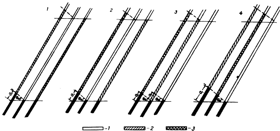
Рис.17. Схемы порядка отработки свиты пластов крутого падения: 1,2,3 - порядок отработки пластов
