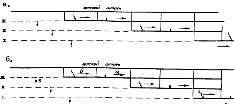
Рис.12. Схема развития работ на передний (а) и задний квершлагах (б)
