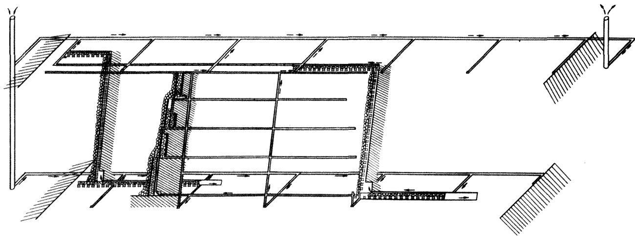
Рис. 20. Соотношение горных работ при обработке свиты пластов крутого падения с опережающим прохождением полевого штрека и работой лав на передовые участковые квершлагги
