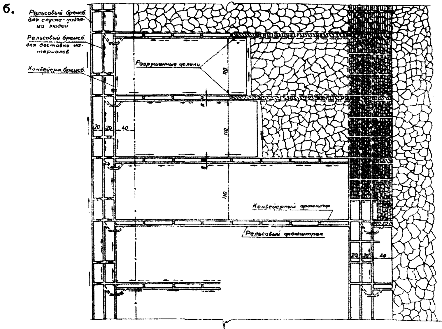
Рис. 35. Односторонняя отработка бремсбергового поля с проходкой выработок узким ходом
