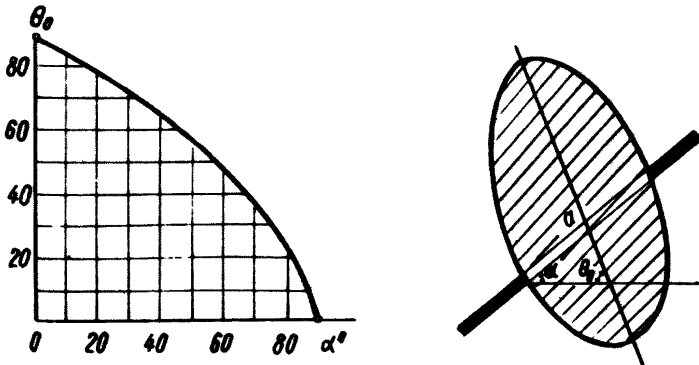
Рис.2. Зависимость положения зоны разгрузки от угла падения пласта
