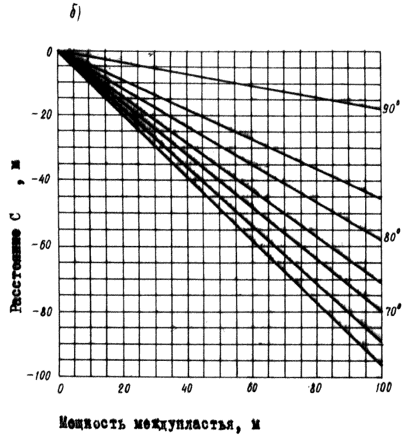
Рис. 4. Расстояние от грани очистных работ на защитном пласте до грани защищенной зоны на опасном пласте в проекции на вертикальную плоскость
