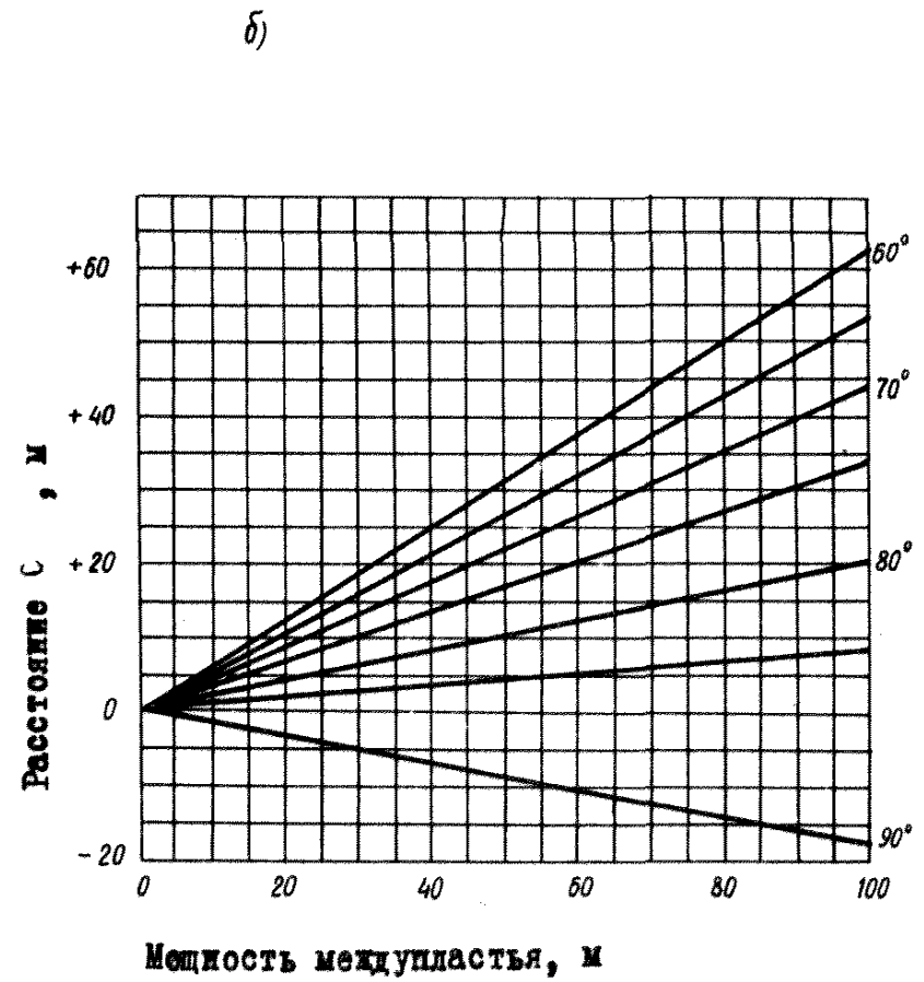
Рис. 3. Расстояние от границ очистных работ на защитном пласте до границ защищенной зоны на опасном пласте в проекции на вертикальную плоскость
