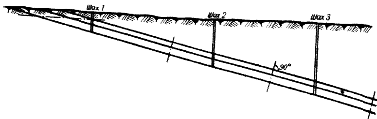
Рис.15. Рекомендуемые границы шахтных полей для свит пластов пологого падения
