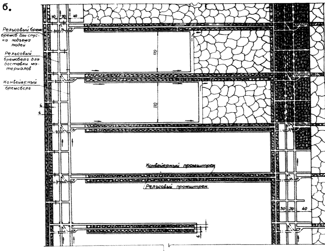
Рис. 34. Односторонняя отработка тормозного поля с проходкой выработок широким ходом
