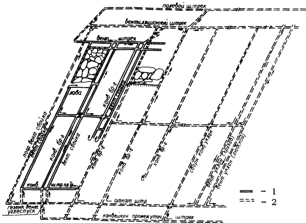
Рис. 36. Схема отработки защитного пласта полосами по падению
