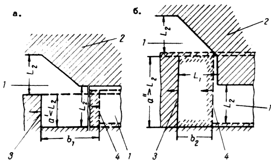
Рис.7. Соотношение работ по защитному и подзащитному пластиам при ведении работ без щелков у вентиляционного горизонта: а-при отставании работ по опасному пласти не более 5 лет; б-при отставании работ по опасному пласти на 0,6(H_0 th) (табл. 2).
