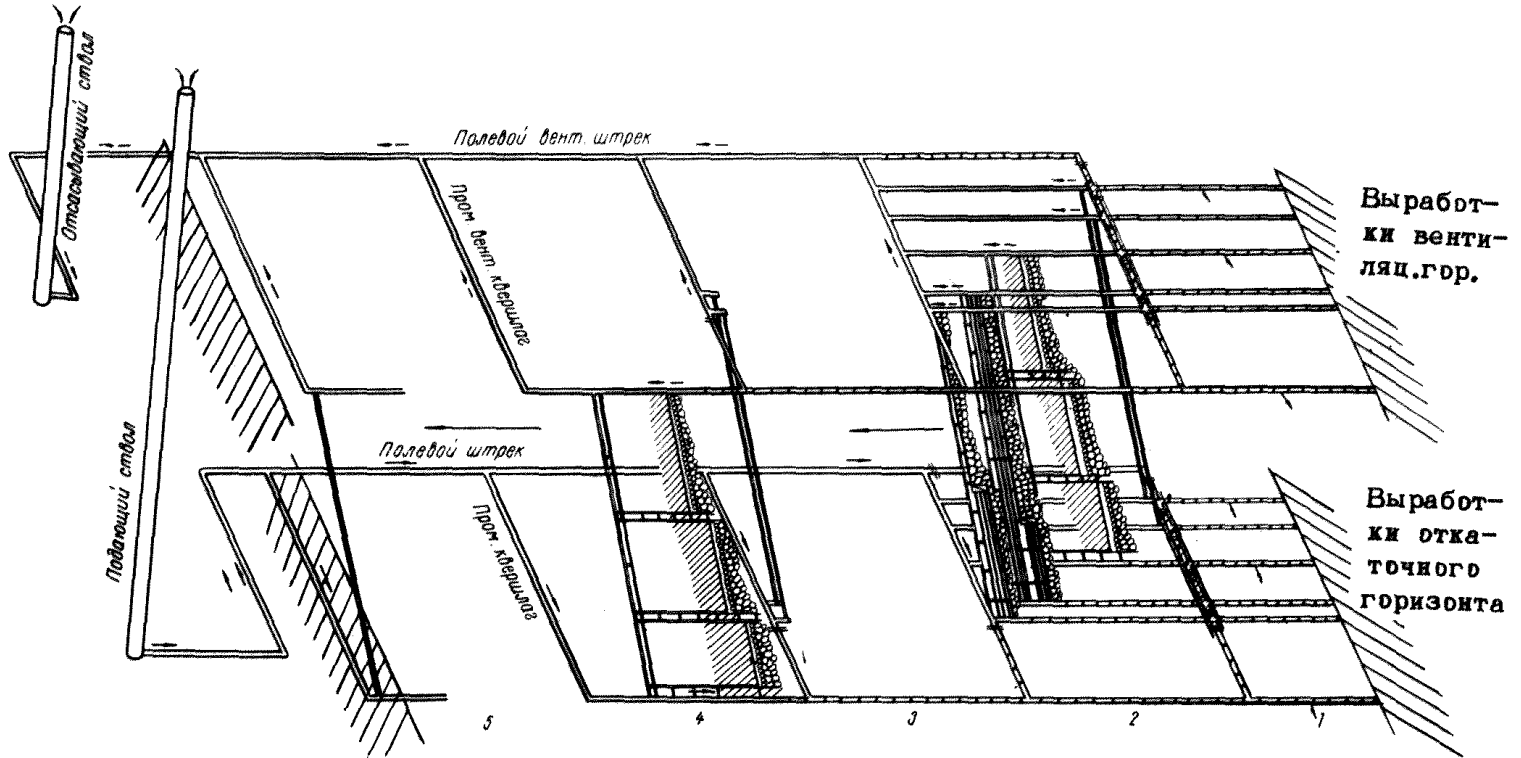
Рис. 27. Последовательная разработка выемочных участков от границ шахтного поля к стволу
