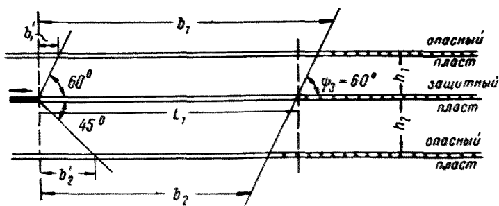
Рис.4. Схема к определению отставания работ по опасному пласту от очистных работ по защитному пласту
