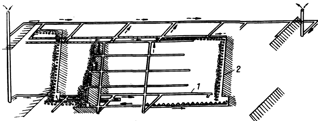
Рис.21. Соотношение горных работ при отработке свиты пластов крутого падения с прохождением полевого штрека в надработанной зоне вслед за очистным забоем защитного пласта и работой лавы защитного пласта на задний квершлаг: 1-полевой штрек; 2-очистной забой по защитному пласту
