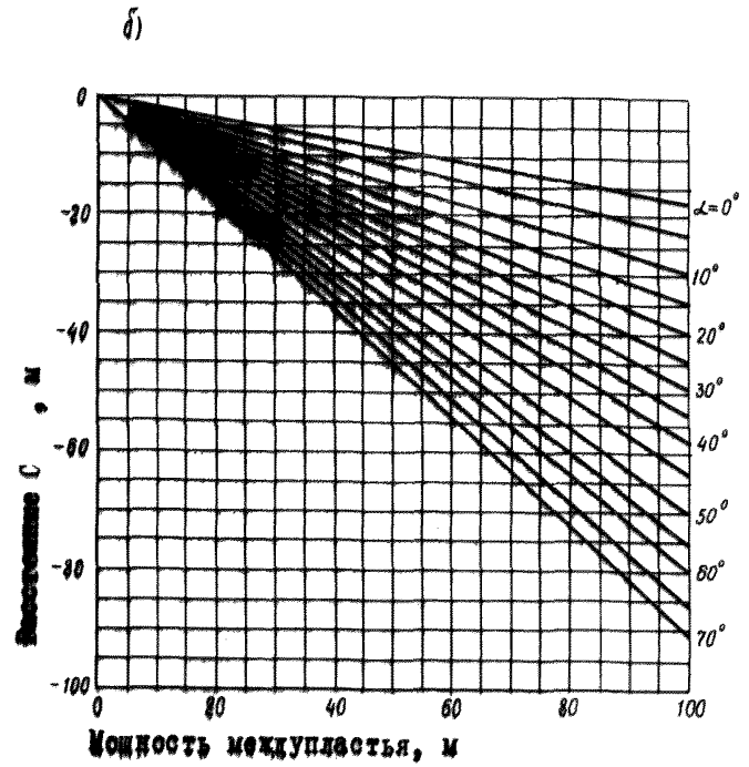
Рис. 1. Расстояние от грани очистных работ на защитном пласте до грани защищенной зоны на опасном пласте на совмещенном плане горных работ при н о д р а б о т к е: а) со стороны падения, б) со стороны восстания. "+" - в сторону массива, "-" - в сторону выработанного пространства.
