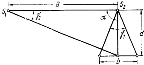
Рис. 15. Схема измерения съемочного базиса с использованием вспомогательного базиса
