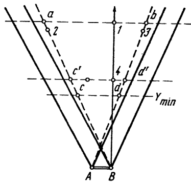
Рис. 11. Расположение корректурных точек в пределах стереопары
