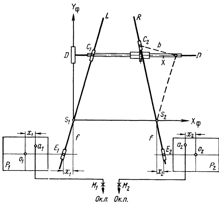
Рис. 5.3. Схема механизма для решения прямой фотограмметрической засечки на стереоаэрофотограмметре
