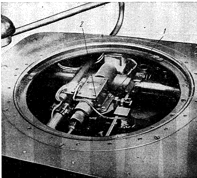
Рис. 3.6. Юстировочные винты для установки измерительных марок
