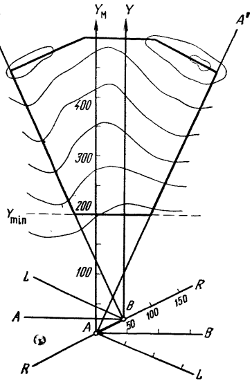
Рис. 8. Палетки для нанесения сектора съемки
