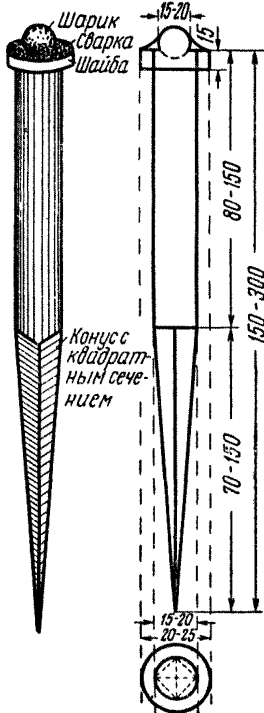
Рис. 52. Металлический костыль.
