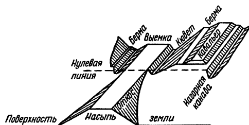
Рис. 81 Элементы земляного полотна.
