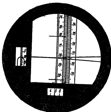
Рис. 30. Поле зрения нивелира Н2.
