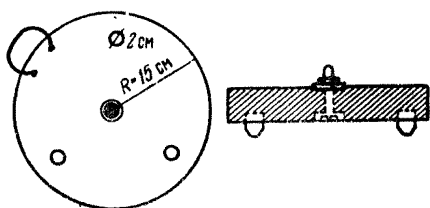
Рис. 53. Деревянный башмак.
