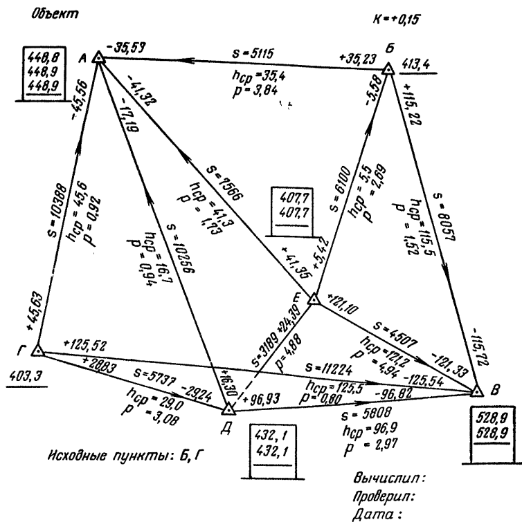
Рис. 92. Схема уравнивания высот пунктов триангуляции.
