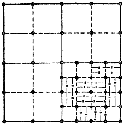
Условные обозначения: — линия нивелирования II класса —●— " " III " основная - - - " " III " заполняющая —·— " " IV " Масштаб 1:100 000
