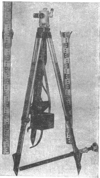
Рис. 44. Комплект нивелира ТН-6.
