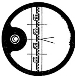
Рис. 36. Поле зрения нивелира NiB-5.
