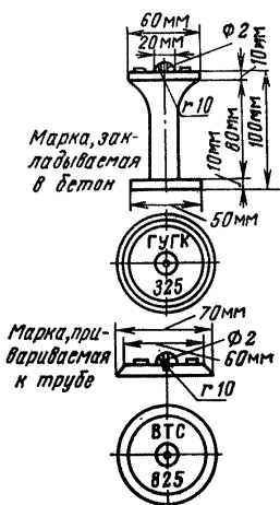
Рис. 10. Марки для грунтовых реперов.
