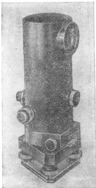
Рис. 32. Нивелир Ni007.
