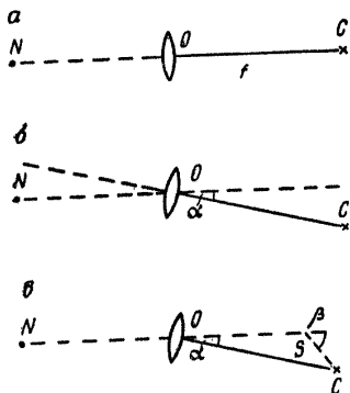
Рис. 31. Принцип работы нивелира с компенсатором.
