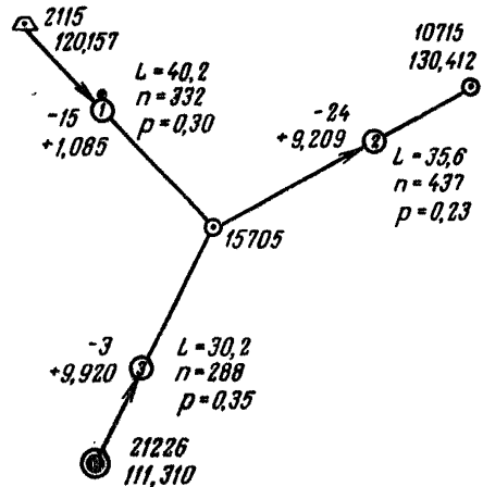
Рис. 91. Уравнивание системы нивелирных линий с одной узловой точкой.
