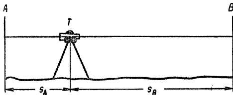
Рис. 79. Определение погрешности за эксцентриситет лимба.
