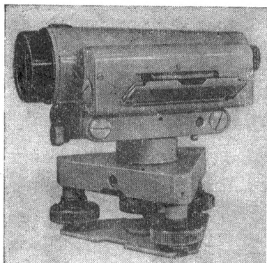
Рис. 22. Нивелир НЗ.
