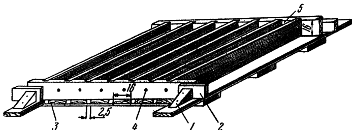
Рис. 21. Многоячейковая опалубка.
