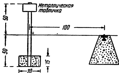
Рис. 19. Трубчатый опознавательный знак для реперов технического нивелирования.
