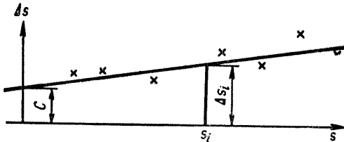
Рис. 84. Определение постоянной дальномера графическим способом.
