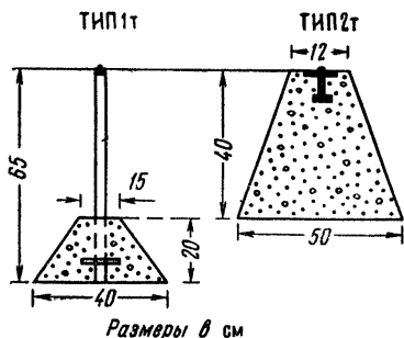
Рис. 16. Реперы для закрепления линий технического нивелирования.
