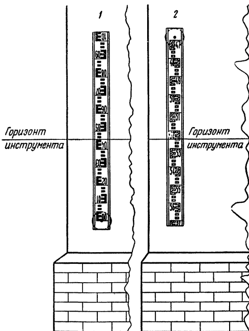
Рис. 64. Привязка к стенным маркам.
