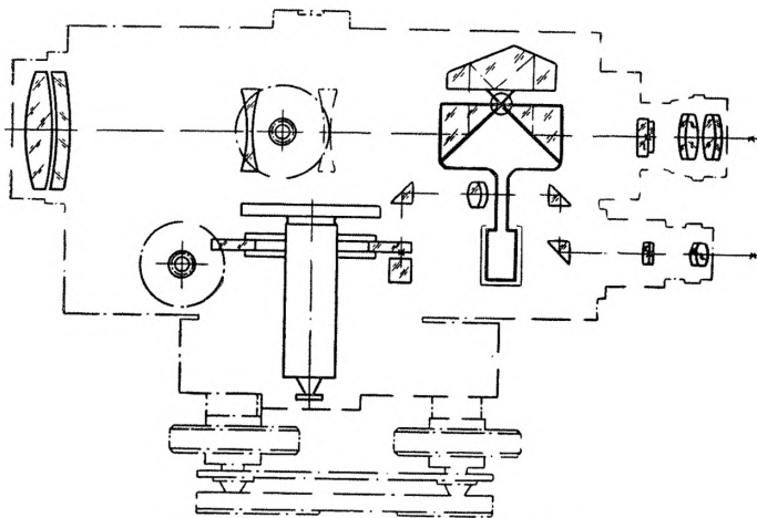
Рис. 41. Оптическая схема нивелира Ni025.
