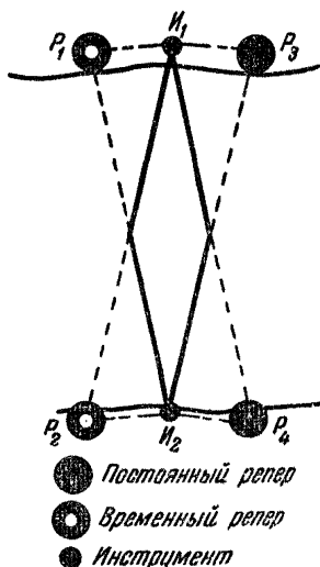
Рис. 69. Передача через препятствия шириной более 200 м.
