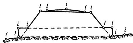
Рис. 82. Места установок рейки при нивелировании труб.
