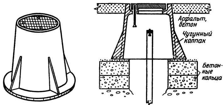
Рис. 15. Чугунный колпак (ковер).
