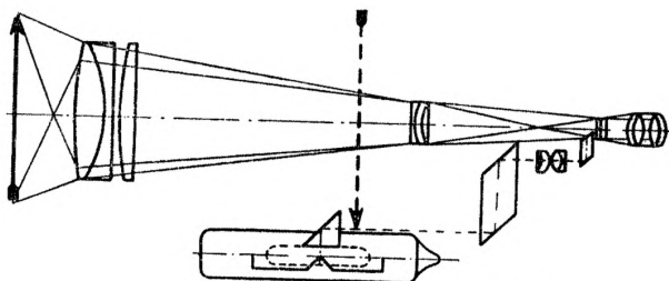
Рис. 43. Оптическая схема нивелира НТ.
