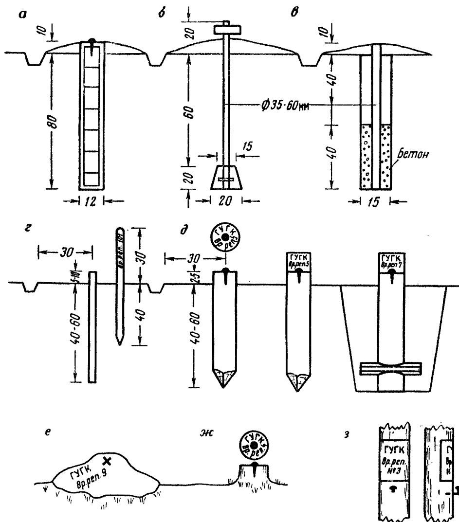
Рис. 20. Временные реперы для зоны сезонного промерзания:
