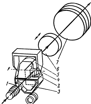
Рис. 37. Оптическая схема нивелира NiB. 1 — сетка нитей; 2, 3 и 4 — призмы компенсатора; 5, 6 и 7 — линзы объектива.
