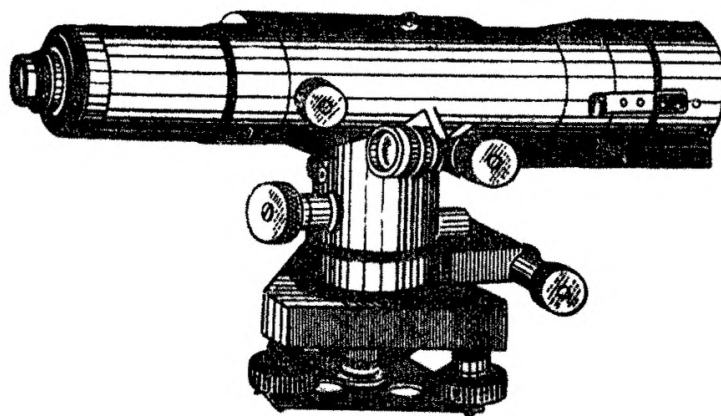
Рис. 29. Нивелир НА-1.
