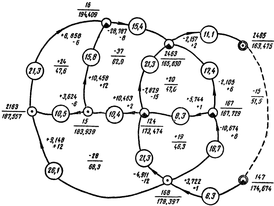
Рис. 89. Уравнивание нивелирной сети методом полигонов.
