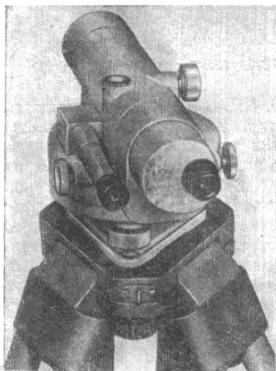
Рис. 35. Нивелир NiB-5.
