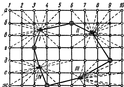
Рис. 76. Способ нивелирования по квадратам.
