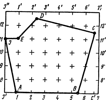
Рис. 75. Разбивка квадратов.
