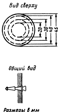
Рис. 7. Стенной репер.
