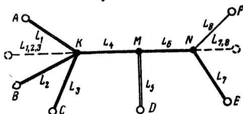
Рис. 93. Уравнивание сети нивелирных линий методом эквивалентной замены.
