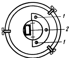
Рис. 55. Крепление сетки нитей нивелира НВ-1.
