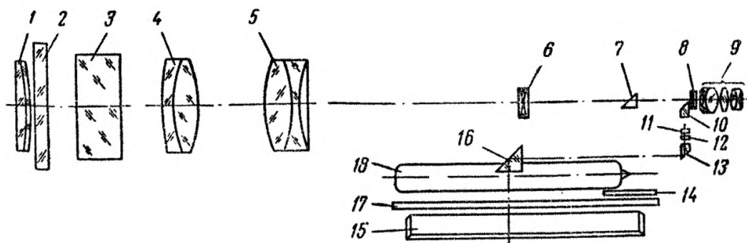
Рис. 28. Оптическая схема нивелира Н2.
