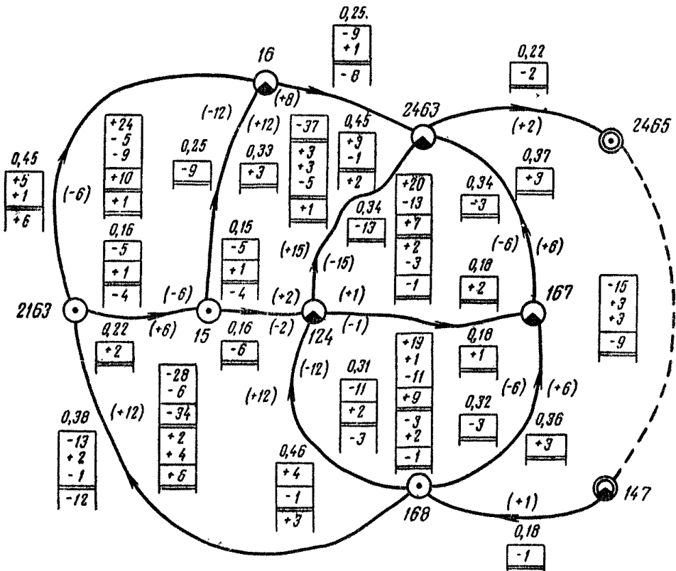
Рис. 90. Уравнивание нивелирной сети методом полигонов.
