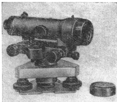
Рис. 23. Нивелир HB-1.
