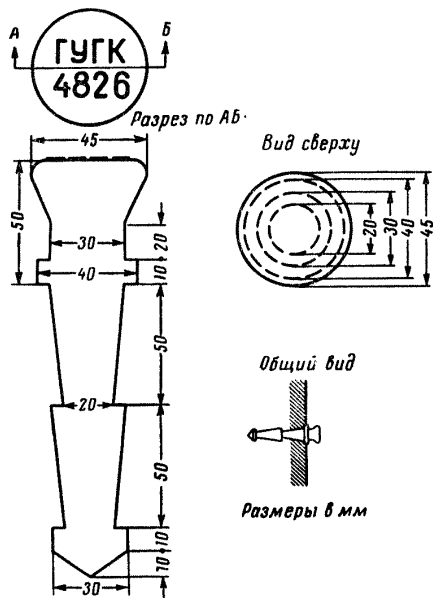
Рис. 7. Стенной репер.
