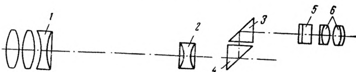
Рис. 39. Оптическая схема нивелира NS4.
