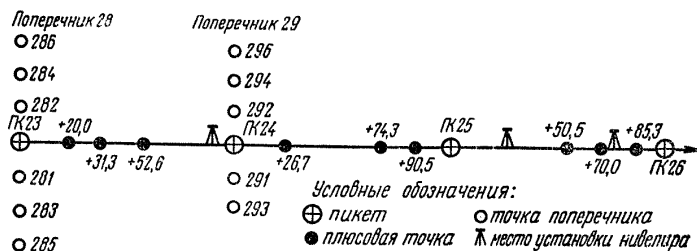
Рис. 71. Участок линии технического нивелирования.
