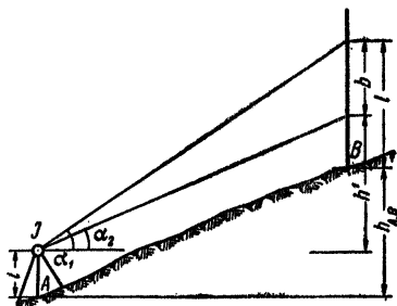
Рис. 86. Измерение превышения методом на две высоты.
