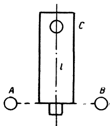
Рис. 54. Определение цены деления круглого уровня.
