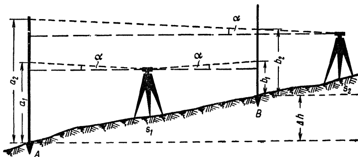
Рис. 58. Определение угла i нивелира вторым способом.
