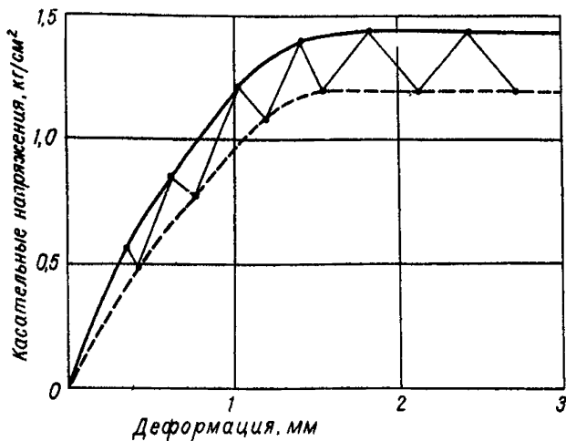
Рис. 20. Зависимость деформации от сдвигающего напряжения на контакте при испытании на длительную прочность
