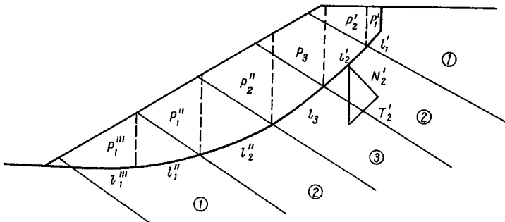
Рис. 22. К расчету устойчивости откосов при совместной работе слоев
