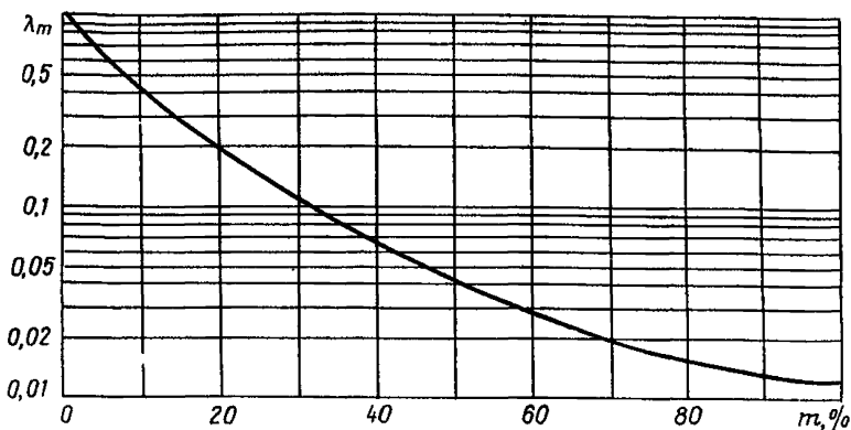
Рис. 16. График зависимости коэффициента \lambda_m от числа наклонных в сторону выемки прерывистых трещин m (%)
