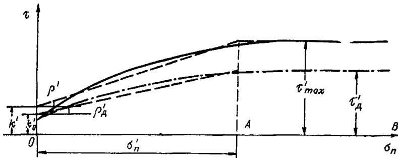
Рис. 1. График зависимости между нормальными и касательными напряжениями при сдвиге по контакту пород:
