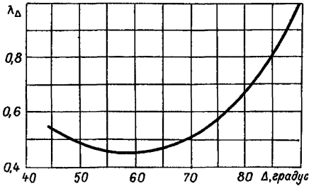
Рис. 13. График зависимости \lambda_{\Delta} от \Delta
