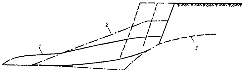
Рис. 9. Пригрузка фильтрующего откоса призмой из скальных пород:
