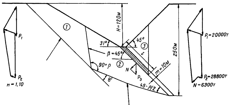
Рис. 24. К расчету устойчивости борта с охранном целиком
