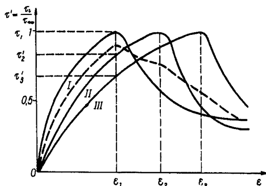
Рис. 21. График кривых бесконечно медленного нагружения при сдвиге слоев с различными деформационными характеристиками
