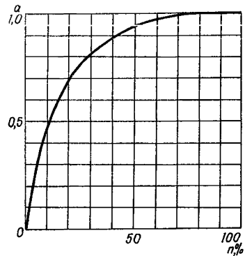
Рис. 12. График зависимости коэффициента разнопрочности a структурных блоков от процентного содержания в массиве блоков малой прочности n
