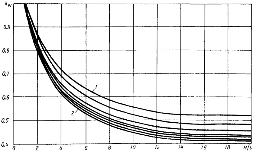
Рис. 11. График зависимости коэффициента структурного ослабления от H/l и \sigma :
