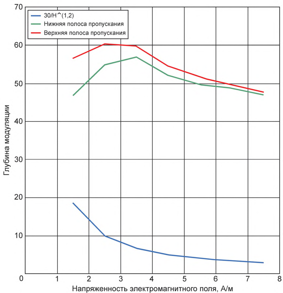
Рисунок ДА.3 — Пример лог-файла с зависимостью глубины модуляции от напряженности электромагнитного поля
