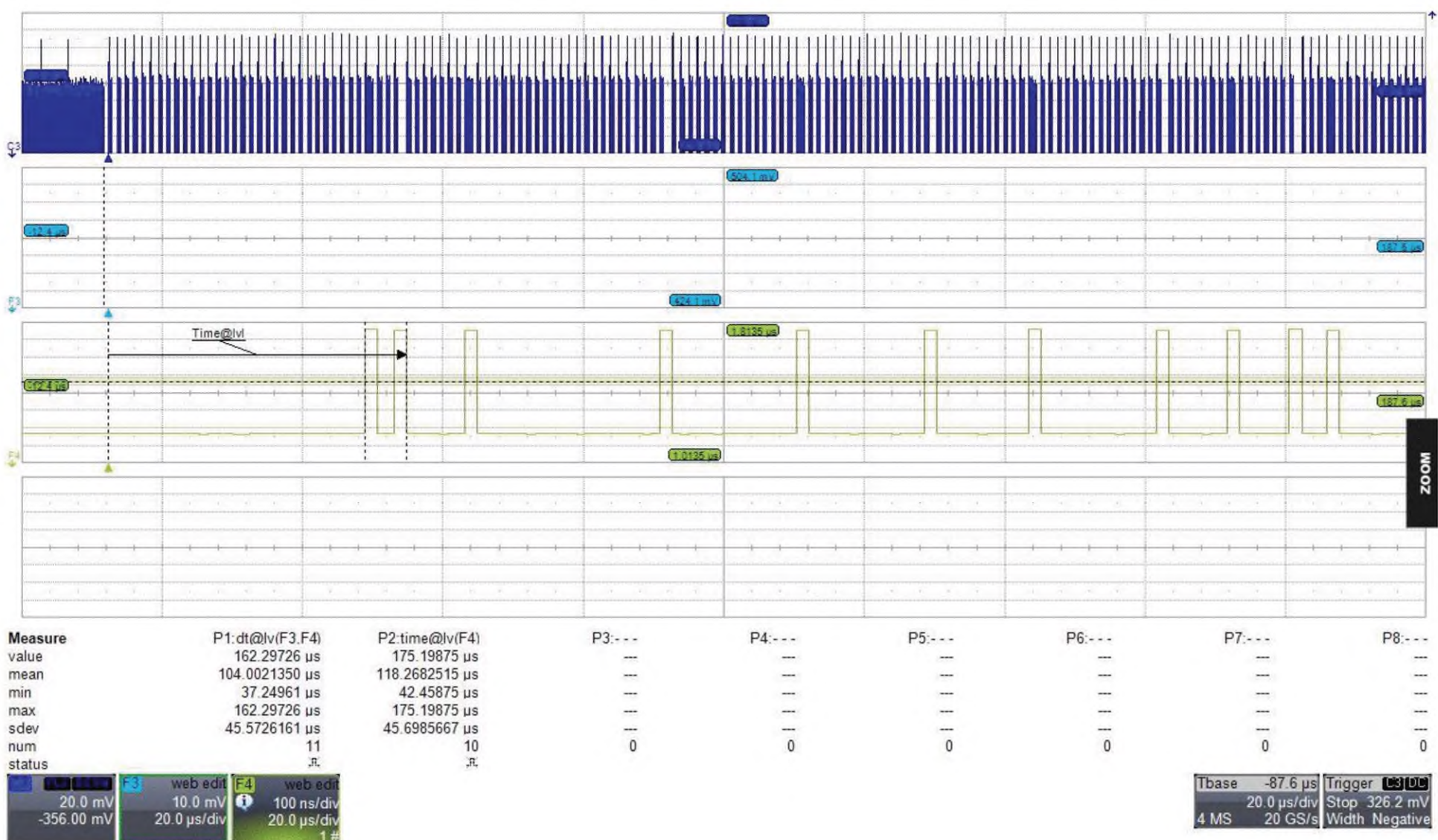
Рисунок ДА.5 — Пример лог-файла с длительностями команд и тестовых последовательностей
