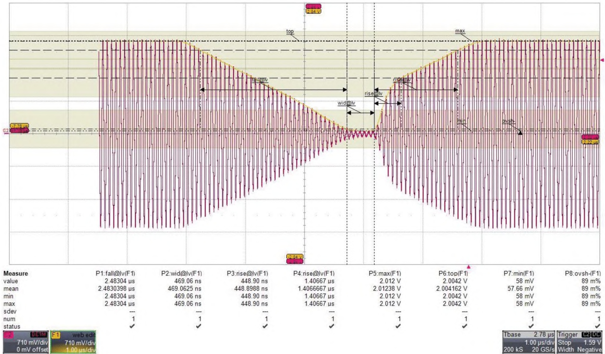
Рисунок ДА.4 — Пример лог-файла с временами спада и нарастания фронтов
