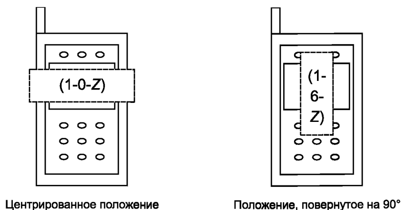
Рисунок 3 — Положения измерения для считывателя eMRTD типа M
