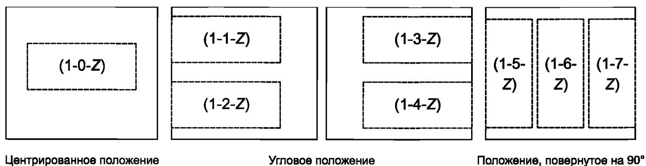
Рисунок 2 — Положения измерения для считывателя eMRTD типа 2 и 3
