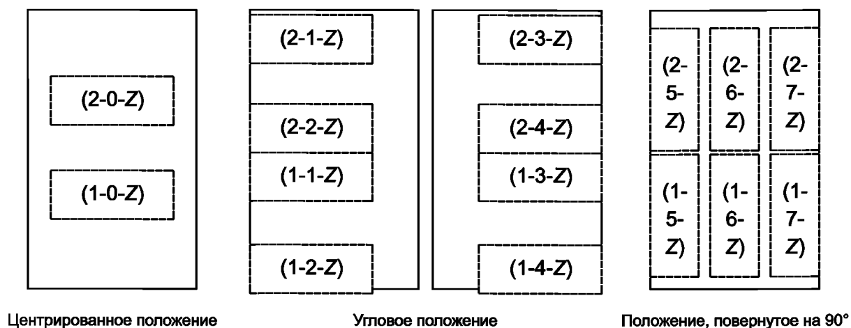
Рисунок 1 — Положения измерения для считывателя eMRTD типа 1
