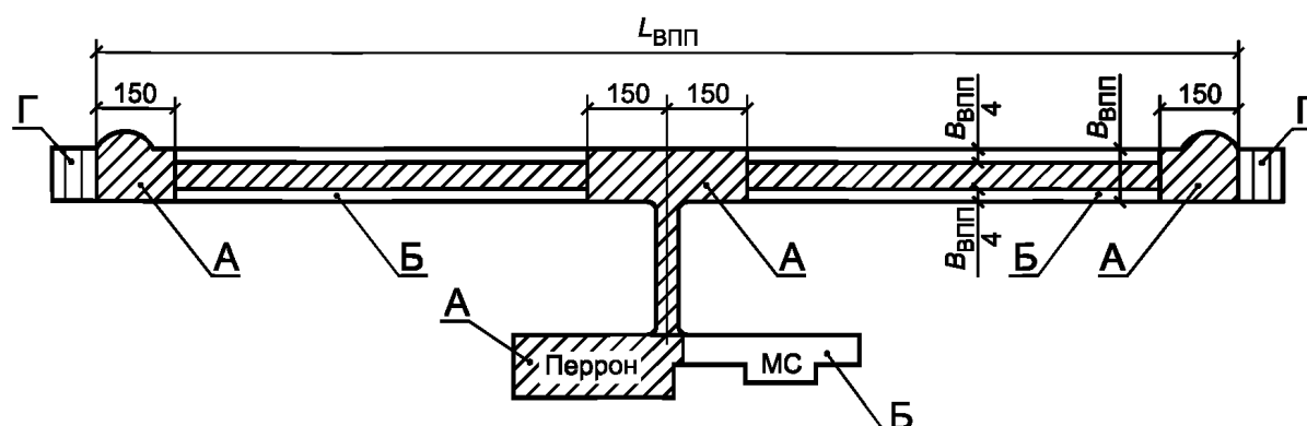
Схема 2
