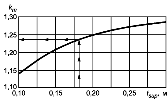
Рисунок К.3 — График для определения поправочного коэффициента k_m при расчете толщины усиления бетонного покрытия t_{sup}
