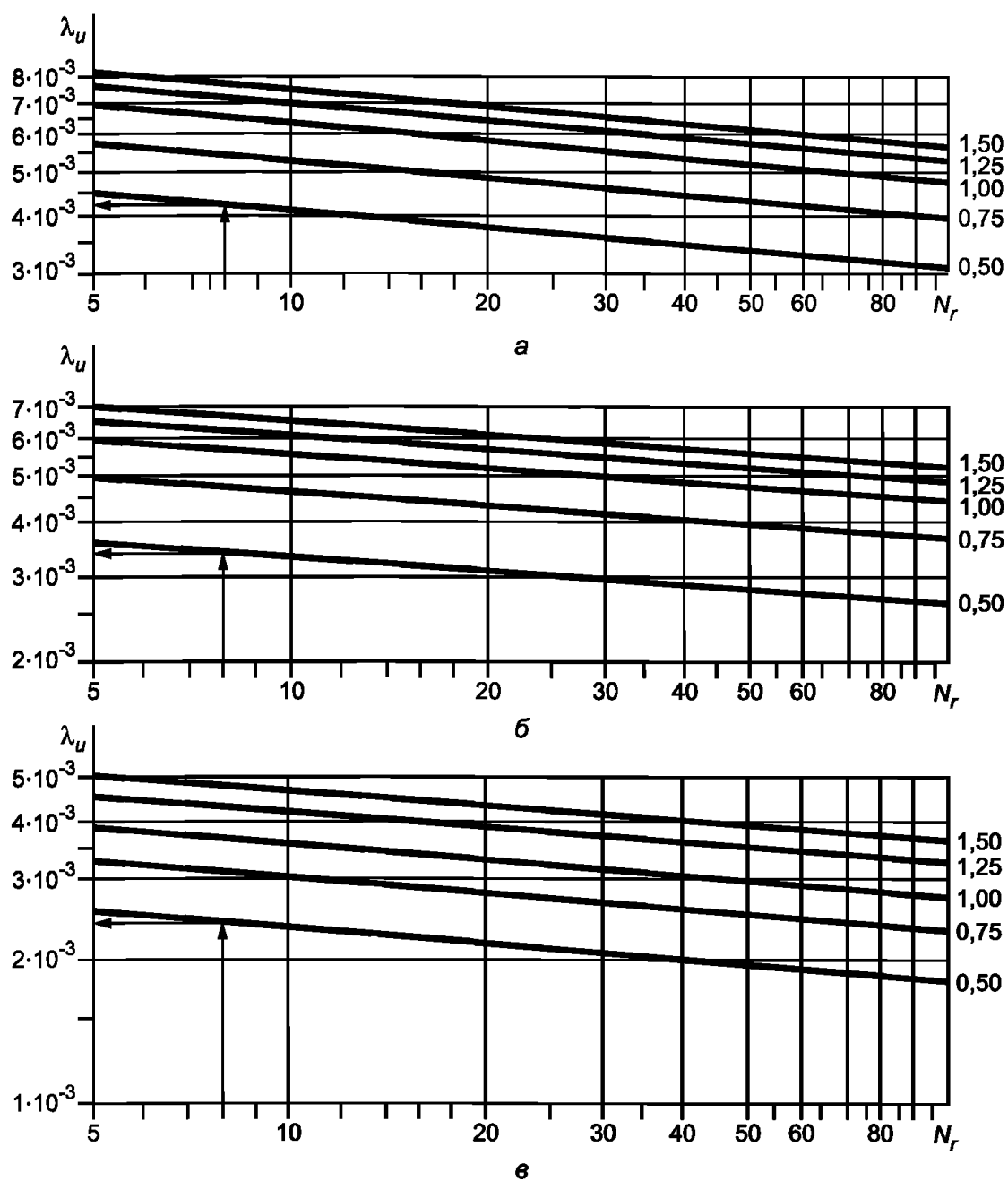
Рисунок К.5 — Графики для определения предельных относительных прогибов \lambda_u нежестких аэродромных покрытий
