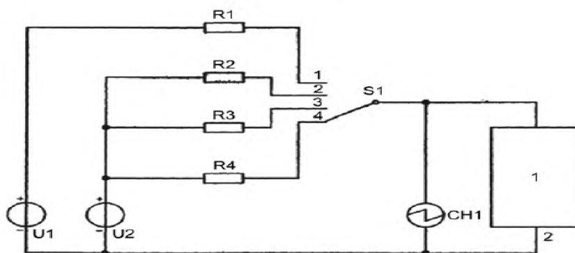
Рисунок А.8 – Электрическая схема испытаний пятипроводного преобразователя
