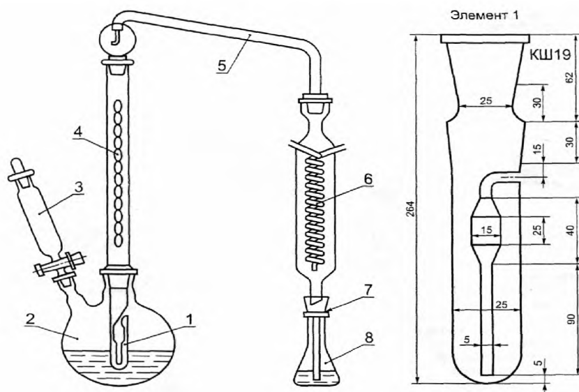
1 – сосуд для перегонки; 2 – колба двугорлая; 3 – делительная воронка с краном; 4 – дефлегматор; 5 – каплеуловитель; 6 – холодильник; 7 – стеклянная воронка; 8 – мерная колба
