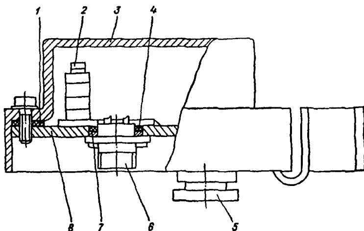
1, 4 — прокладка; 2 — плата; 3 — крышка; 5 — герметизированный вывод кабеля; 6 — вилка разъема; 7 — шайба; 8 — основание
