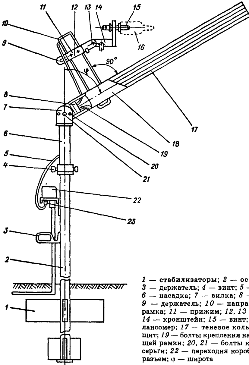
Рисунок Д.2 — Теневая стойка
