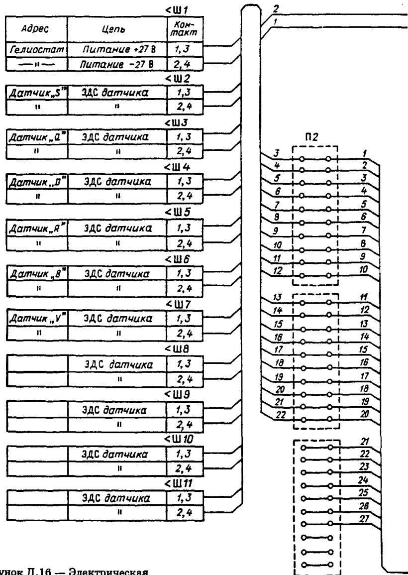
Рисунок Д.16 — Электрическая схема соединительной коробки
