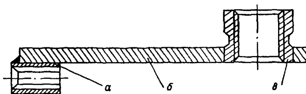
a — гайка; б — кронштейн; в — гнездо для пиранометра
