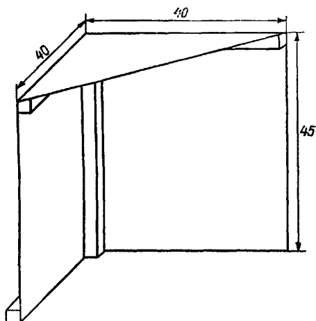
Рисунок Д.13 — Щит для затенения измерительных приборов при выполнении контроля или поверки
