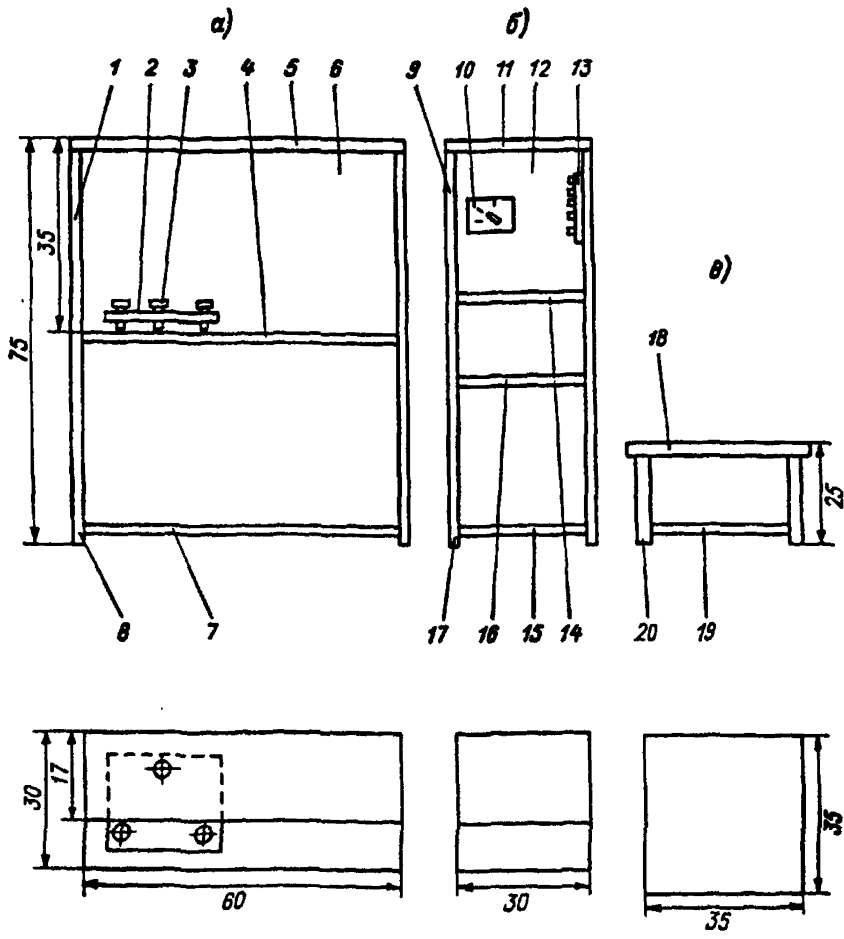
а) поверочный стол: 1 — боковая стенка; 2 — панель; 3 — установочные винты панели; 4 — полка для измерительных приборов; 5 — полка для актинометров; 6 — задняя стенка; 7 — переключатель; 8 — ножка б) тумбочка: 9 — боковая стенка; 10 — переключатель; 11 — козырек; 12 — задняя стенка; 13 — панель с клеммами; 14 — столешница; 15 — переключатель; 16 — полка; 17 — ножка в) подставка для поверочной трубы: 18 — столешница; 19 — переключатель; 20 — ножка
