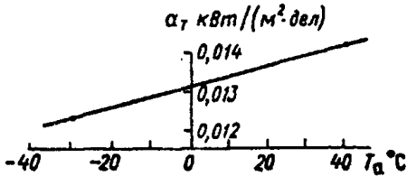
Рисунок В.1 — Зависимость переводного множителя актинометра М-3 № 792 с гальванометром ГСА-1 № 541 от температуры
