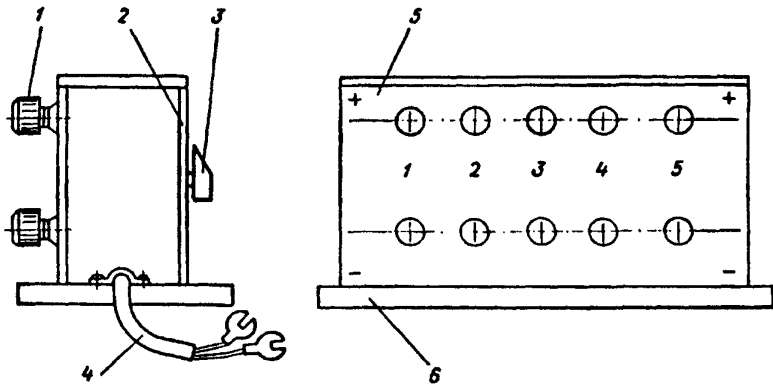
1 — клеммы для подключения датчиков; 2 — передняя панель; 3 — рукоятка; 4 — выводы к измерительному прибору; 5 — задняя панель; 6 — дно
