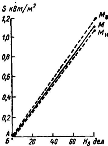
Рисунок 5 — Пример графика зависимости прямой солнечной радиации от ординаты записи сигналов актинометра на диаграммной ленте регистратора
