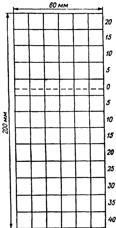
Рисунок 3 — Общий вид палетки Савиковского для обработки диаграммных лент регистратора
