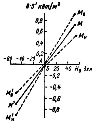
Рисунок 6 — Пример графика зависимости радиационного баланса без прямой солнечной радиации от ординаты записи сигналов балансомера на диаграммной ленте регистратора
