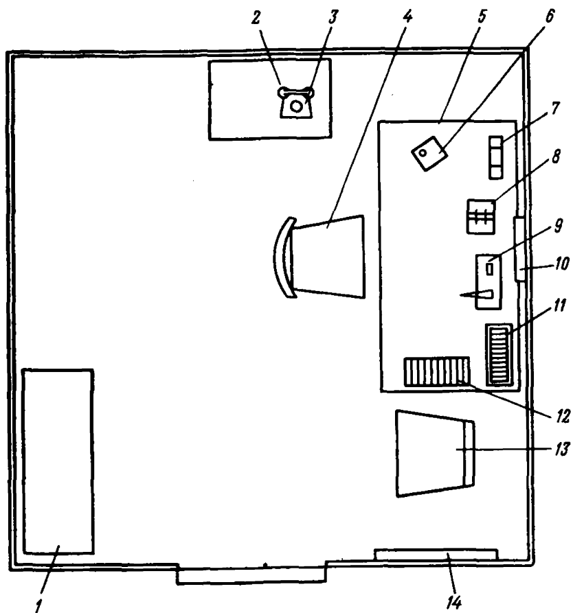
Рис. 12. Схема организации рабочего места мастера производственного участка :
