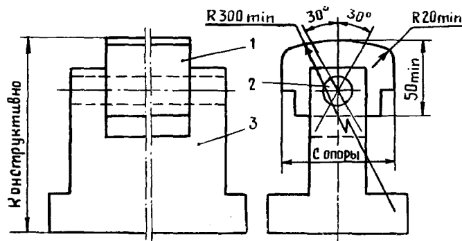
Рис. 5. Типовая конструкция опор для правки панелей к прессам типа ПП-250:
