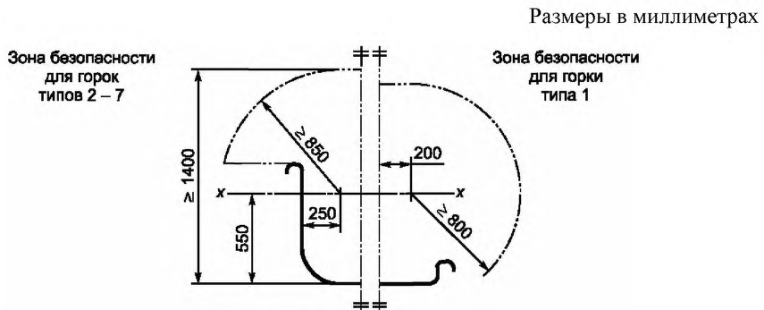
Рисунок 14 — Размеры зон безопасности для горок
