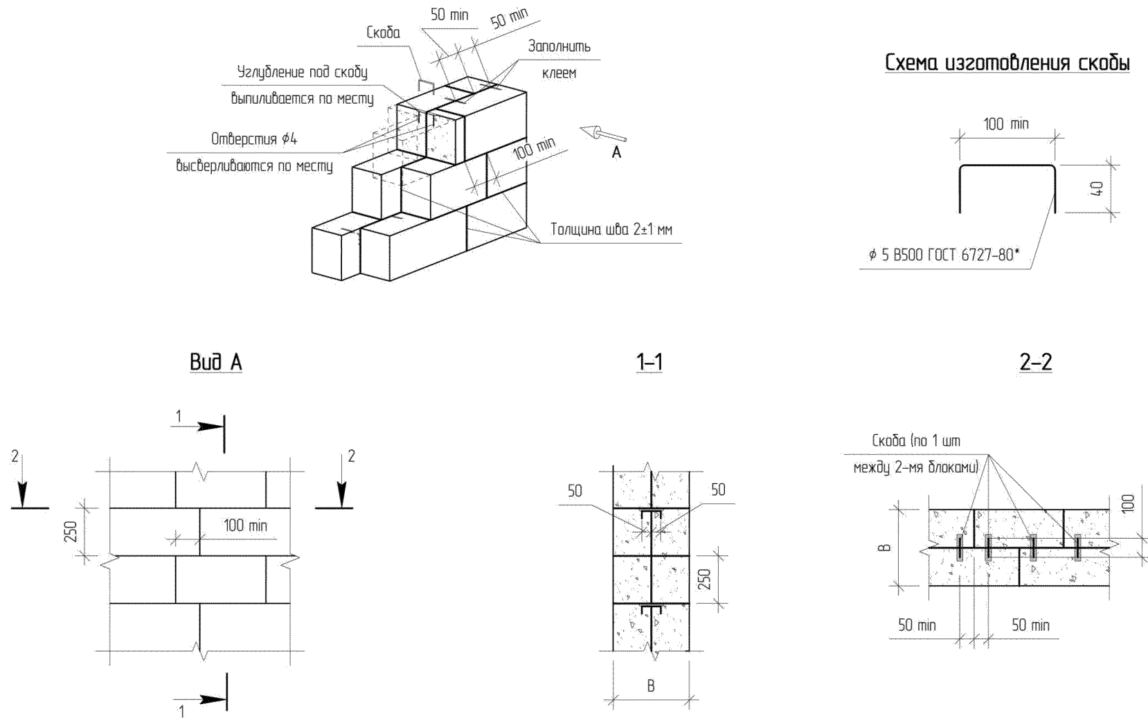
Рис. 3.3. Схема кладки стен толщиной в два одинаковых по толщине блока
