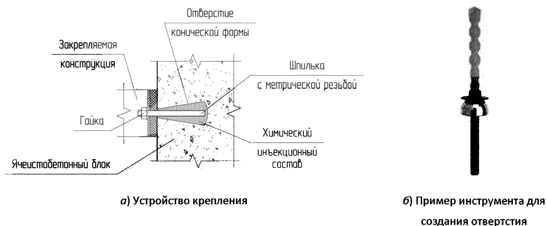
Рис. Б.1. Химический анкер с анкерровкой формой
