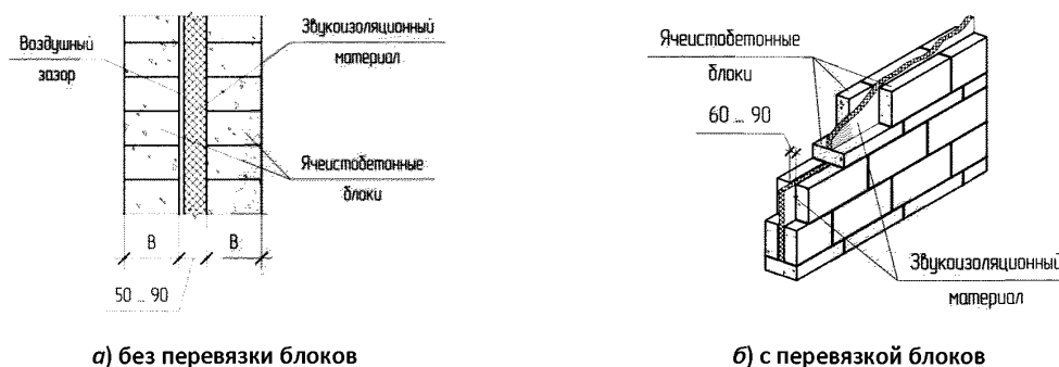
Рис. 3.4. Примеры устройства стен со звукоизоляционной прослойкой
