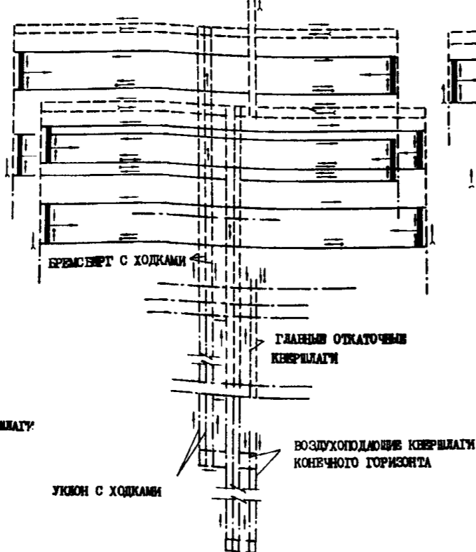
ОДНОВРЕМЕННАЯ ОБРАБОТКА ДВУХ ПЛАСТОВ ДВУМЯ ПАНЕЛЯМИ С НАРЕЗКОЙ ЧЕТЫРЕХ ЛАВ В КАЖДОЙ ПАНЕЛИ
