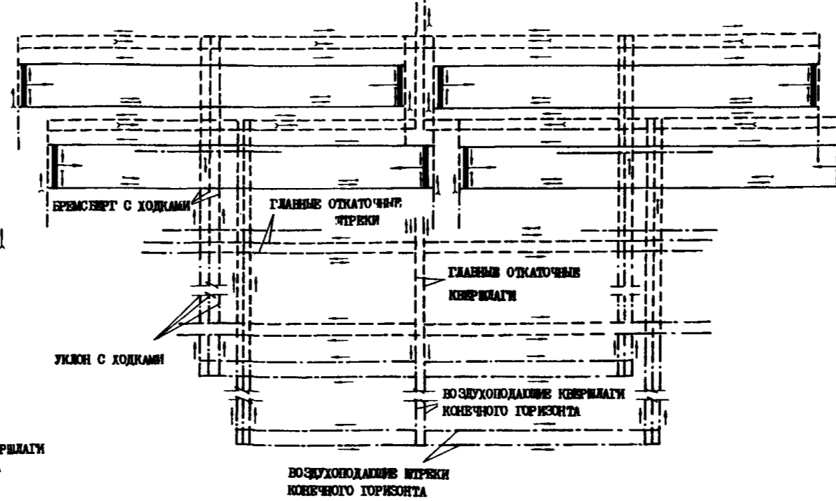
ОДНОВРЕМЕННАЯ ОБРАБОТКА ДВУХ ПЛАСТОВ ЧЕТЫРЬМЯ ПАНЕЛЯМИ С НАРЕЗКОЙ ДВУХ ЛАВ В КАЖДОЙ ПАНЕЛИ
