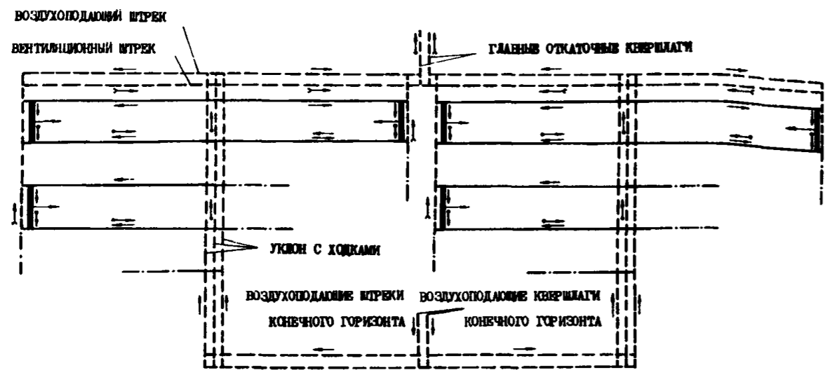
ОДНОВРЕМЕННАЯ ОТРАБОТКА ДВУХ ПЛАСТОВ ДВУМЯ ПАНЕЛЯМИ С НАРЕЗКОЙ ЧЕТЫРЕХ ЛАВ В КАЖДОЙ ПАНЕЛИ
