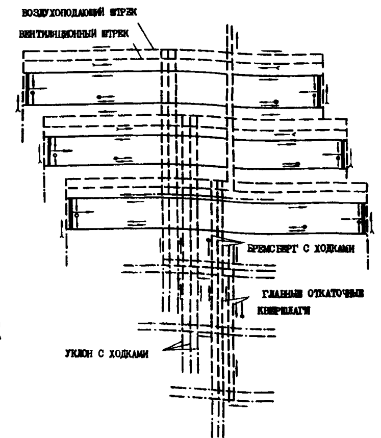
ОДНОВРЕМЕННАЯ ОТРАБОТКА ТРЕХ ПЛАСТОВ ТРЕМИ ПАНЕЛЯМИ С НАРЕЗКОЙ ДВУХ ЛАВ В КАЖДОЙ ПАНЕЛИ
