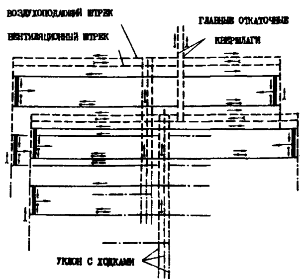
ОДНОВРЕМЕННАЯ ОБРАБОТКА ДВУХ ПЛАСТОВ ДВУМЯ ПАНЕЛЯМИ С НАРЕЗКОЙ ТРЕХ ЛАВ В КАЖДОЙ ПАНЕЛИ
