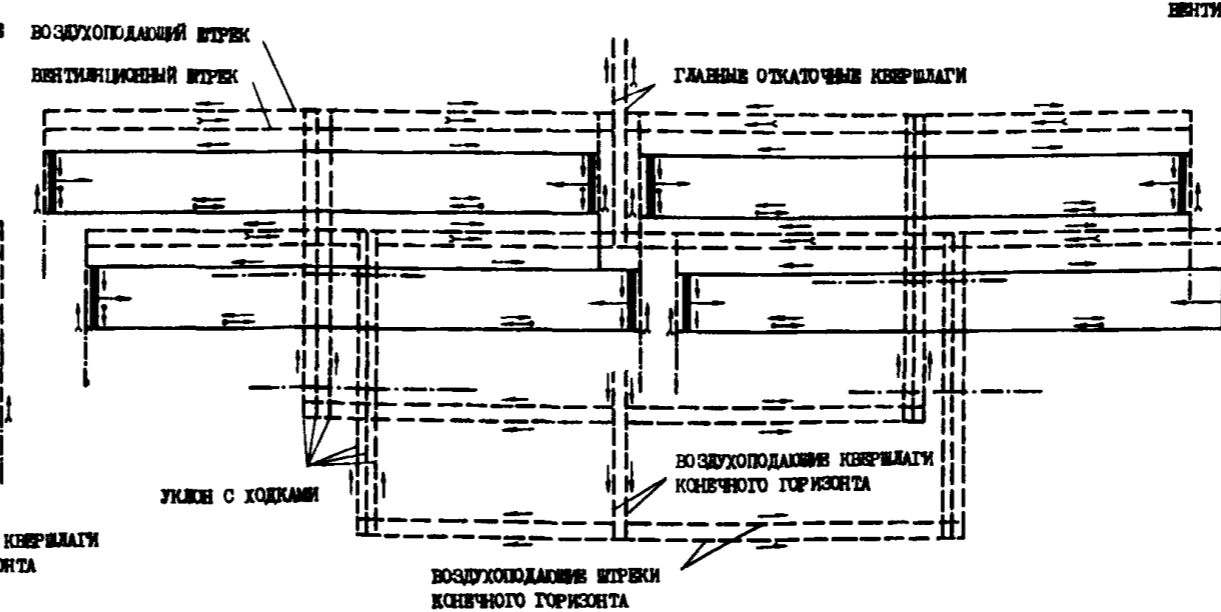
ОДНОВРЕМЕННАЯ ОТРАБОТКА ДВУХ ПЛАСТОВ ЧЕТЫРЬМЯ ПАНЕЛЯМИ С НАРЕЗКОЙ ДВУХ ЛАВ В КАЖДОЙ ПАНЕЛИ
