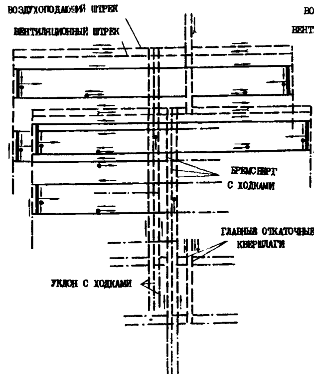
ОДНОВРЕМЕННАЯ ОТРАБОТКА ДВУХ ПЛАСТОВ ДВУМИ ПАНЕЛЯМИ С НАРЕЗКОЙ ТРЕХ ЛАВ В КАЖДОЙ ПАНЕЛИ
