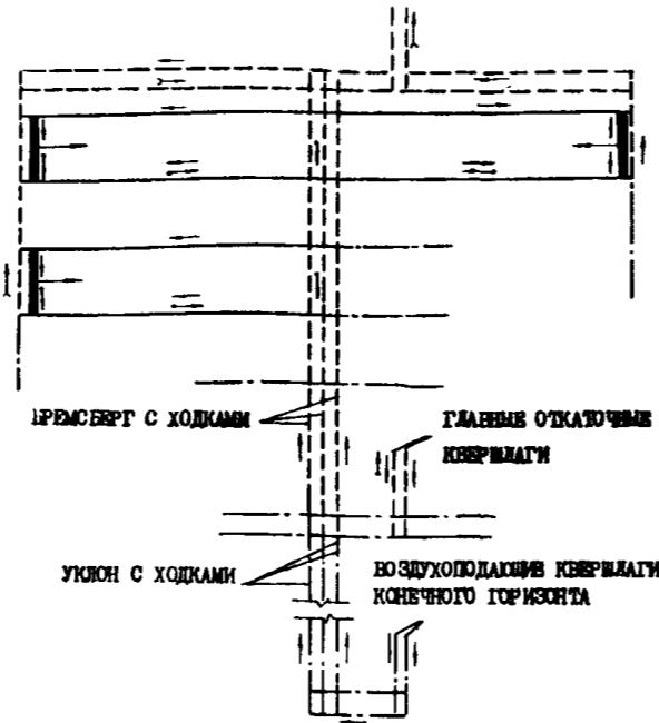
ОБРАБОТКА ОДНОГО ПЛАСТА ДВУМЯ ПАНЕЛЯМИ С НАРЕЗКОЙ ЧЕТЫРЕХ ЛАВ В КАЖДОЙ ПАНЕЛИ
