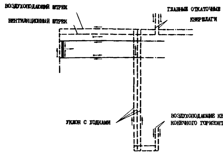
ОТРАБОТКА ОДНОГО ПЛАСТА ДВУМЯ ПАНЕЛЯМИ С НАРЕЗКОЙ ТРЕХ ЛАВ В КАЖДОЙ ПАНЕЛИ
