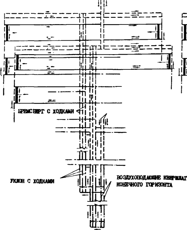
ОДНОВРЕМЕННАЯ ОБРАБОТКА ДВУХ ПЛАСТОВ ДВУМЯ ПАНЕЛЯМИ С НАРЕЗКОЙ ТРЕХ ЛАВ В КАЖДОЙ ПАНЕЛИ
