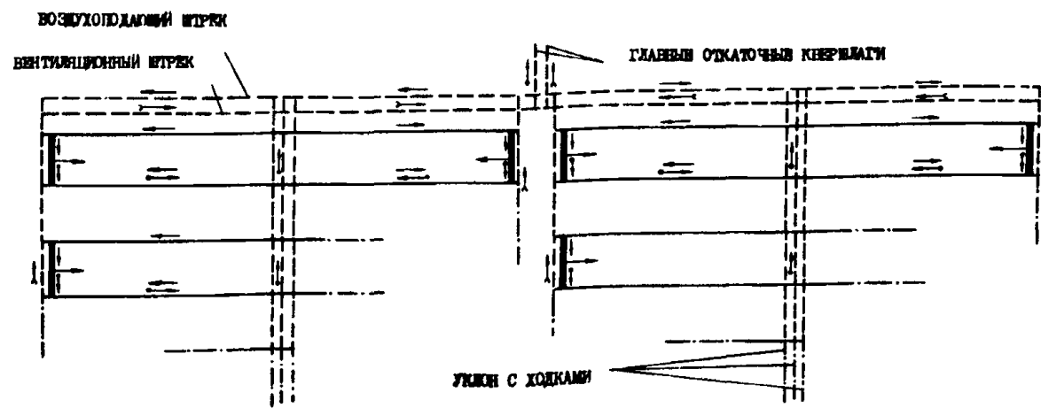
ОДНОВРЕМЕННАЯ ОБРАБОТКА ДВУХ ПЛАСТОВ ДВУМЯ ПАНЕЛЯМИ С НАРЕЗКОЙ ЧЕТЫРЕХ ЛАВ В КАЖДОЙ ПАНЕЛИ
