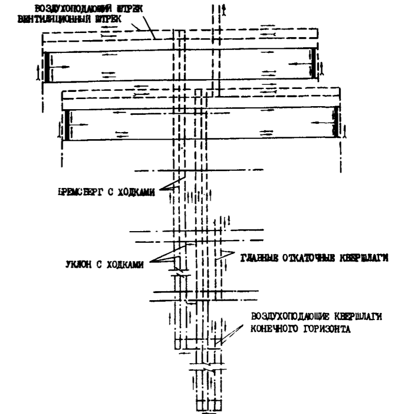
ОДНОВРЕМЕННАЯ ОБРАБОТКА ДВУХ ПЛАСТОВ ДВУМЯ ПАНЕЛЯМИ С НАРЕЗКОЙ ДВУХ ЛАВ В КАЖДОЙ ПАНЕЛИ
