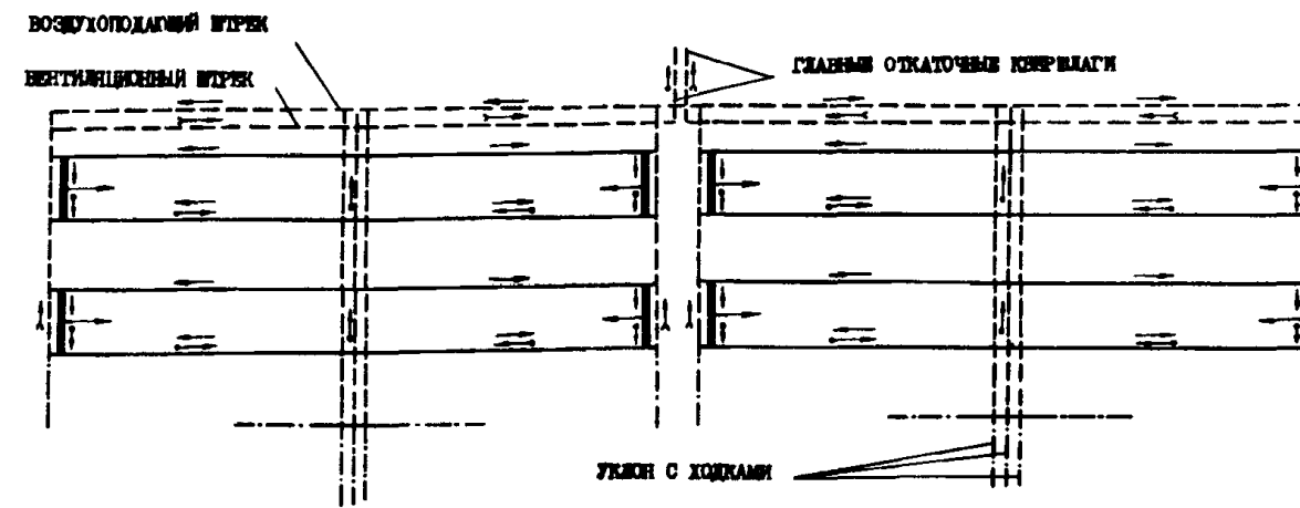
ОДНОВРЕМЕННАЯ ОБРАБОТКА ДВУХ ПЛАСТОВ ЧЕТЫРЬМЯ ПАНЕЛЯМИ С НАРЕЗКОЙ ДВУХ ЛАВ В КАЖДОЙ ПАНЕЛИ
