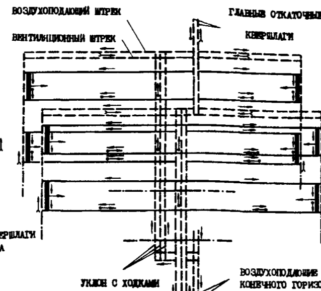
ОДНОВРЕМЕННАЯ ОТРАБОТКА ДВУХ ПЛАСТОВ ДВУМЯ ПАНЕЛЯМИ С НАРЕЗКОЙ ЧЕТЫРЕХ ЛАВ В КАЖДОЙ ПАНЕЛИ
