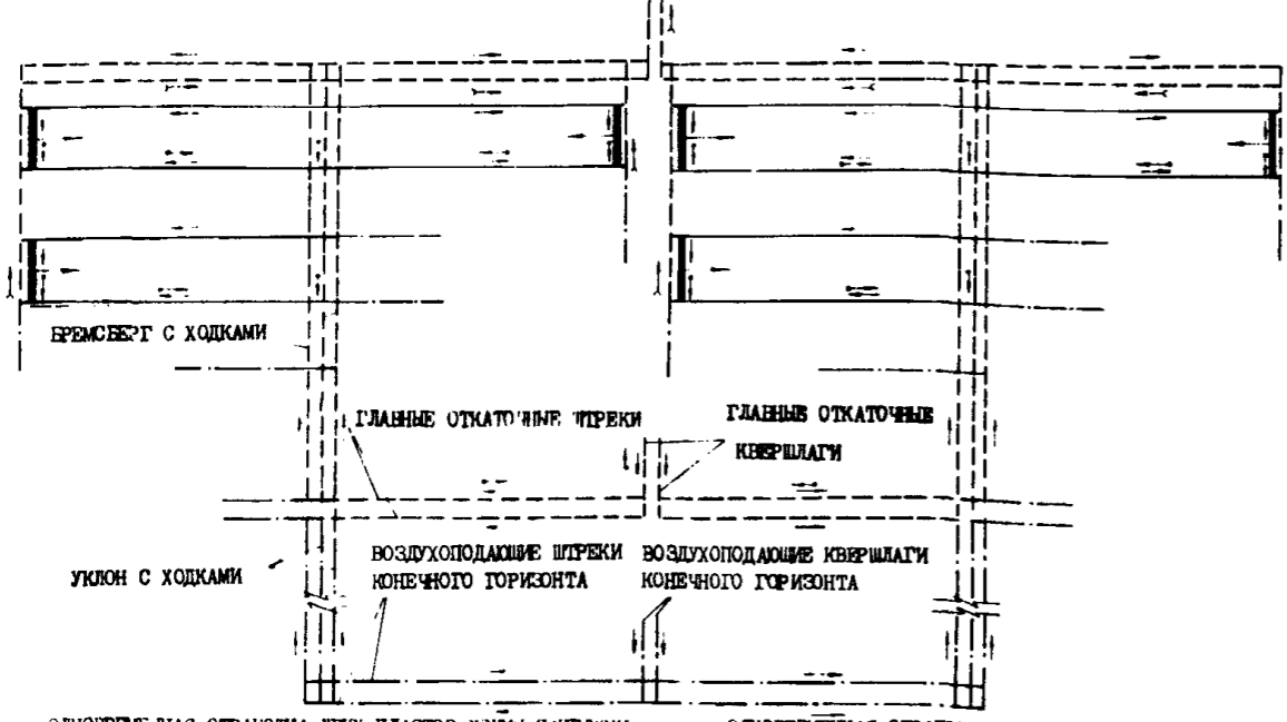
ОДНОВРЕМЕННАЯ ОБРАБОТКА ДВУХ ПЛАСТОВ ДВУМЯ ПАНЕЛЯМИ С НАРЕЗКОЙ ТРЕХ ЛАВ В КАЖДОЙ ПАНЕЛИ
