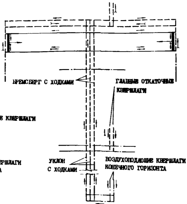
ОБРАБОТКА ОДНОГО ПЛАСТА ДВУМЯ ПАНЕЛЯМИ С НАРЕЗКОЙ ТРЕХ ЛАВ В КАЖДОЙ ПАНЕЛИ
