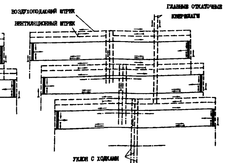
ОДНОВРЕМЕННАЯ ОБРАБОТКА ТРЕХ ПЛАСТОВ ТРЕМЯ ПАНЕЛЯМИ С НАРЕЗКОЙ ДВУХ ЛАВ В КАЖДОЙ ПАНЕЛИ
