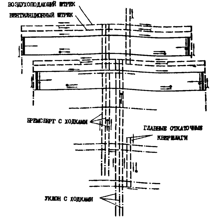
ОДНОВРЕМЕННАЯ ОТРАБОТКА ДВУХ ПЛАСТОВ ДВУМИ ПАНЕЛЯМИ С НАРЕЗКОЙ ДВУХ ЛАВ В КАЖДОЙ ПАНЕЛИ
