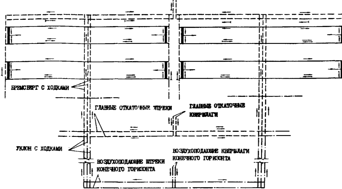
ОДНОВРЕМЕННАЯ ОБРАБОТКА ДВУХ ПЛАСТОВ ЧЕТЫРЬМЯ ПАНЕЛЯМИ С НАРЕЗКОЙ ДВУХ ЛАВ В КАЖДОЙ ПАНЕЛИ
