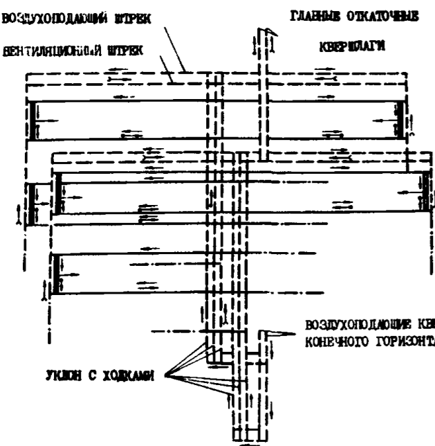
ОДНОВРЕМЕННАЯ ОТРАБОТКА ДВУХ ПЛАСТОВ ДВУМЯ ПАНЕЛЯМИ С НАРЕЗКОЙ ТРЕХ ЛАВ В КАЖДОЙ ПАНЕЛИ
