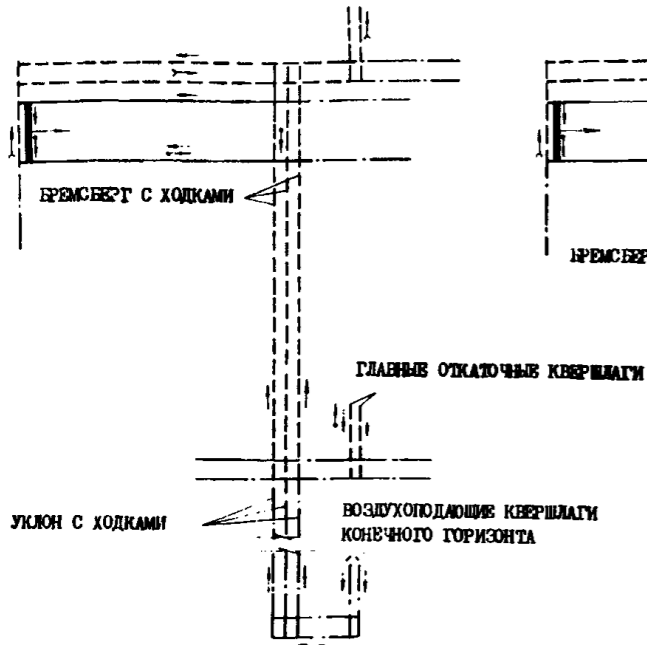
ОБРАБОТКА ОДНОГО ПЛАСТА ДВУМЯ ПАНЕЛЯМИ С НАРЕЗКОЙ ТРЕХ ЛАВ В КАЖДОЙ ПАНЕЛИ
