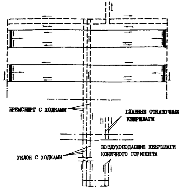
ОБРАБОТКА ОДНОГО ПЛАСТА ДВУМЯ ПАНЕЛЯМИ С НАРЕЗКОЙ ЧЕТЫРЕХ ЛАВ В КАЖДОЙ ПАНЕЛИ
