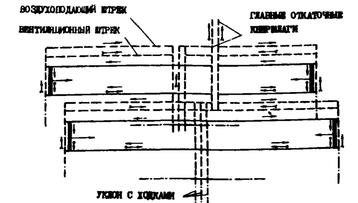
ОДНОВРЕМЕННАЯ ОБРАБОТКА ДВУХ ПЛАСТОВ ДВУМЯ ПАНЕЛЯМИ С НАРЕЗКОЙ ДВУХ ЛАВ В КАЖДОЙ ПАНЕЛИ
