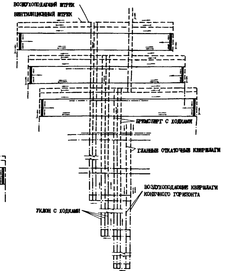
ОДНОВРЕМЕННАЯ ОБРАБОТКА ТРЕХ ПЛАСТОВ ТРЕМЯ ПАНЕЛЯМИ С НАРЕЗКОЙ ДВУХ ЛАВ В КАЖДОЙ ПАНЕЛИ
