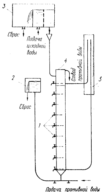
Рис. 15. Установка для определения фильтровальных характеристик воды 1—пробоотборники; 2—стабилизирующий бак; 3—бак для исходной воды; 4—фильтровальная колонка; 5—пьезометры
