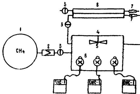
1 - емкость с метаном, 2 - дозирующее устройство, 3 - химпоглотитель (осушитель), 4 - испытательная камера, 5 - вентилятор, 6 - испытуемый СМС-1, 7 - насос, 8 - интерферометр ИТР-1 (ЛИ-4)
