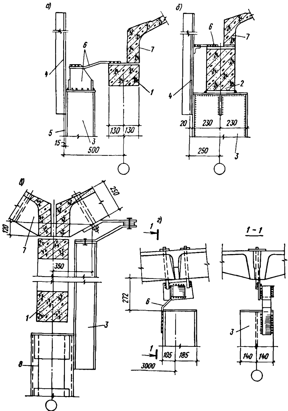
Рис. 34. Крепление фахверковых колонн
