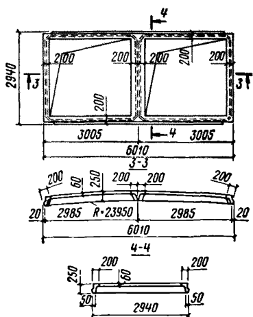
Рис. 10. Плиты с проемами для светоаэрационных фонарей (тип ПБ-7 — с двумя проемами и тип ПБ-8 — с одним проемом)
