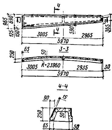
Рис. 8. Доборные крайние плиты (тип ПБ-5 и в зеркальном изображении ПБ-4)
