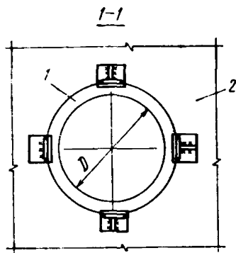
Рис. 45. Деталь крепления стакана к плите оболочки
