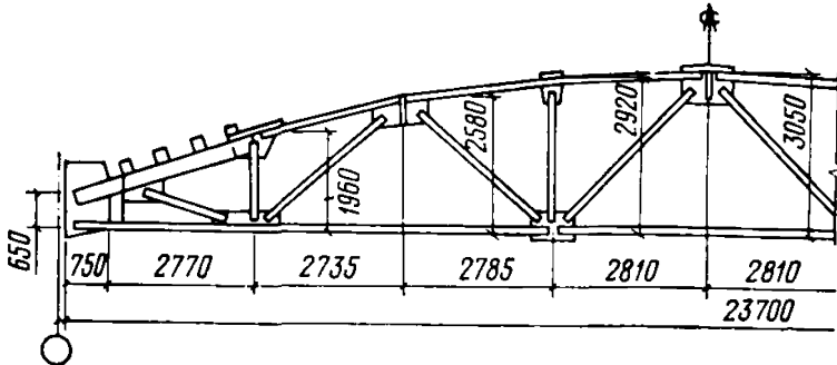
Рис. 16. Стальная контурная ферма пролетом 24 м (тип ФКМ-24)
