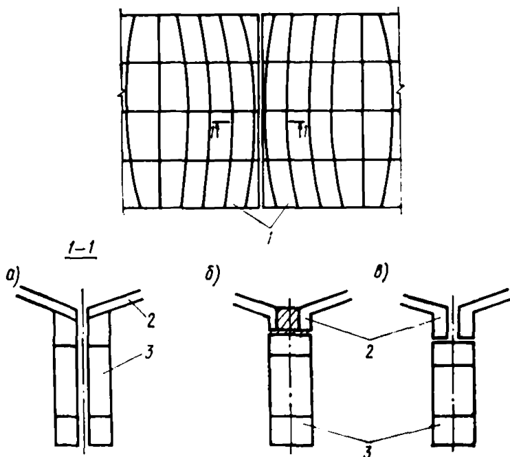
Рис. 3. Типы оболочек по сопряжению в системе покрытия а — отдельно стоящие; б — неразрезные; в — с тангенциально-подвижным сопряжением; 1 — смежные оболочки; 2 — плиты; 3 — контурные элементы
