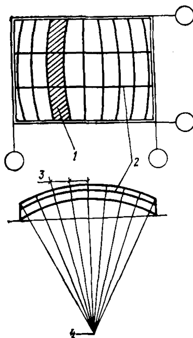
Рис. 2. Схема разрезки исходной поверхности
