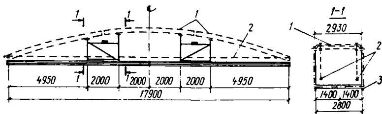
Рис. 51. Монтажная схема стенда укрупнительной сборки плит 1 — плиты оболочки; 2 — стальные затяжки; 3 — стенд
