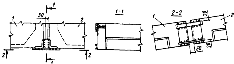
Рис. 22. Соединение плит при укрупнительной сборке 1 — контурные плиты; 2 — средние плиты
