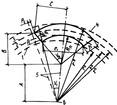
Рис. 54. Определение координат точек реальных поверхностей
