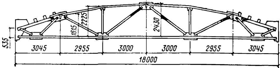
Рис. 15. Стальная контурная ферма пролетом 18 м (тип ФКМ-18)
