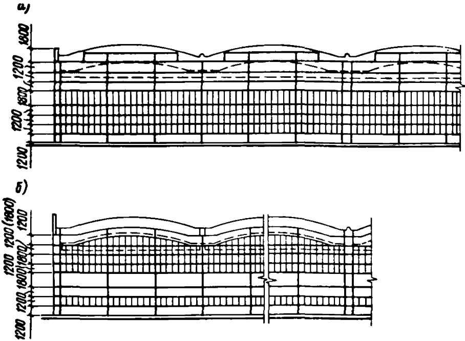
Рис. 35. Примеры решения фасадов а — с парапетными панелями прямолинейного очертания; б — с парапетными панелями криволинейного очертания
