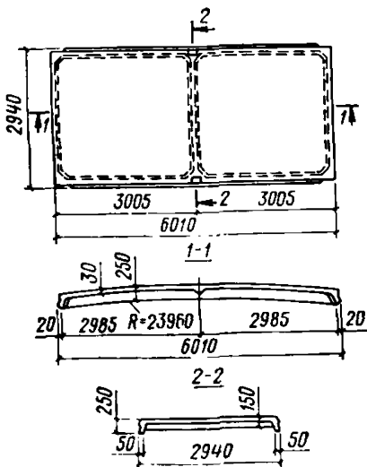
Рис. 5. Средняя плита (тип П6-1)
