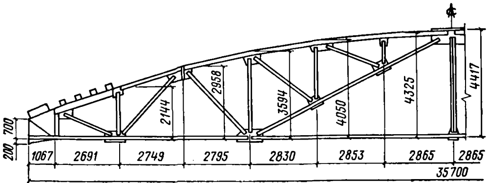
Рис. 18. Стальная контурная ферма пролетом 36 м (тип ФКМ-36)
