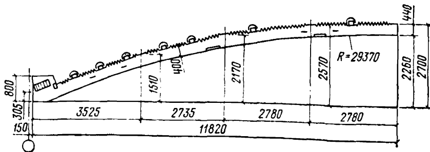
Рис. 14. Железобетонные контурные балки для пролета 24 м (тип БКБ-24)
