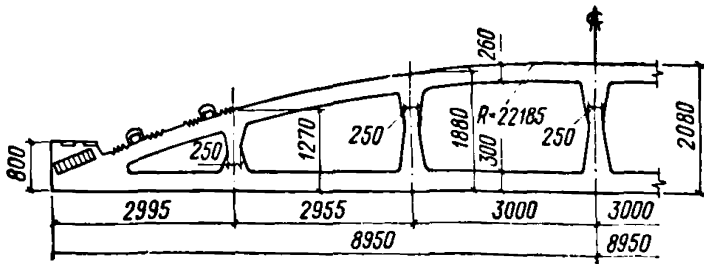
Рис. 11. Железобетонная ферма пролетом 18 м (тип ФКБ-18)
