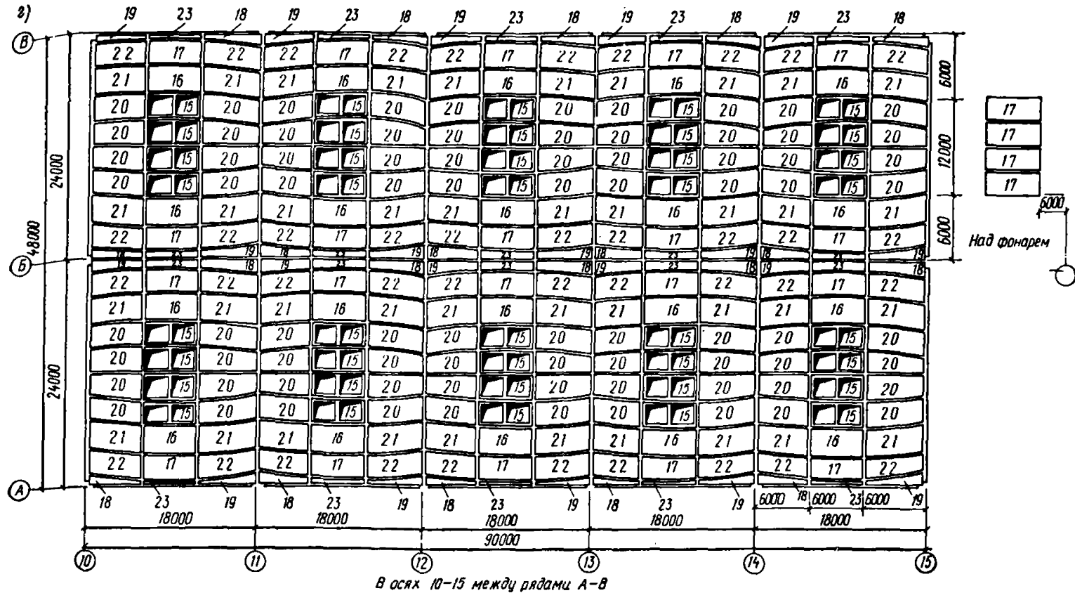
Рис. 29. Пример применения типовых конструкций оболочек
