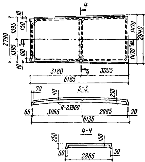
Рис. 6. Контурная плита (тип П6-2)
