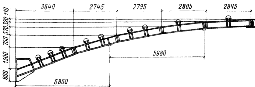
Рис. 21. Стальная контурная балка для пролета 30 м
