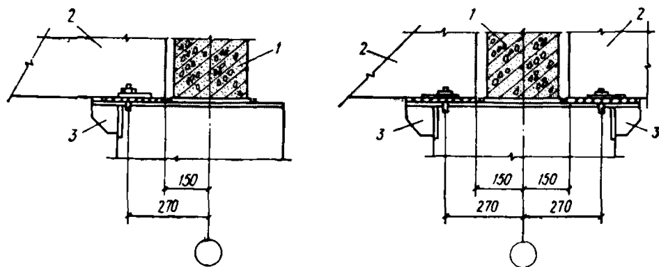
Рис. 33. Устройство опорных столиков для опирания ферм 1 — ферма пролетом 18 м; 2 — ферма пролетом 24 м; 3 — опорный столик
