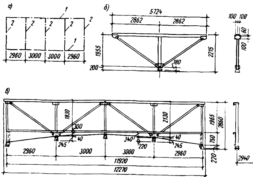
Рис. 42. Стальные несущие конструкции фонаря а — маркировочная схема; б — схема поперечной фермы ФФ-1; в — схема продольной фермы ФП-1; 1 — продольная ферма; 2 — поперечная ферма
