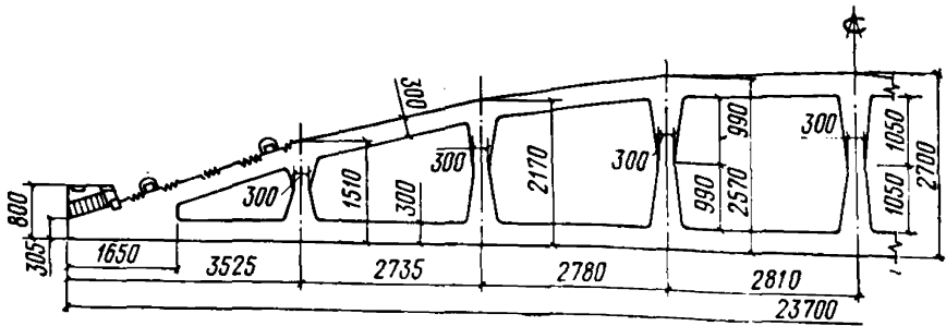
Рис. 12. Железобетонная ферма пролетом 24 м (тип ФКБ-24)
