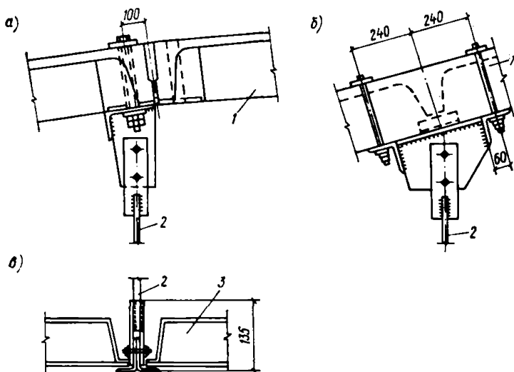
Рис. 48. Детали крепления подвесных потолков
