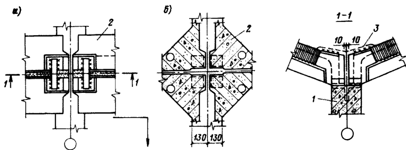
Рис. 25. Соединение плит у примыкания смежных оболочек
