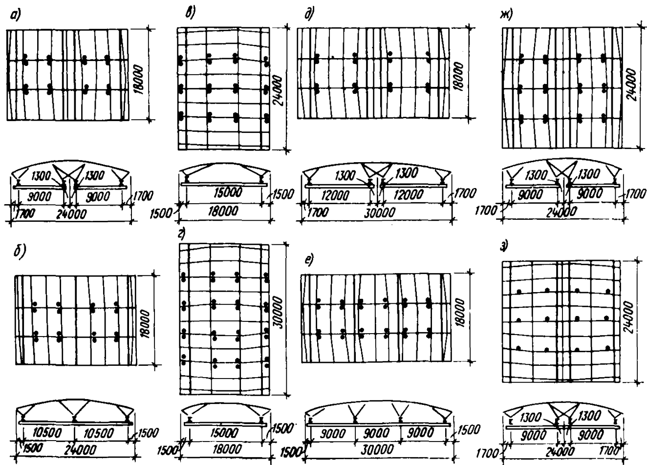
Рис. 46. Схемы размещения путей подвешного транспорта а, б, в — для оболочки 18×24 м соответственно при продольном (по отношению к плитам) движении двух и одного кранов и при поперечном движении одного крана; г, д, е, — для оболочки 18×30 м соответственно при поперечном движении одного крана и при продольном движении двух и одного кранов; ж, з — для оболочки 24×24 м при продольном и поперечном движении двух кранов
