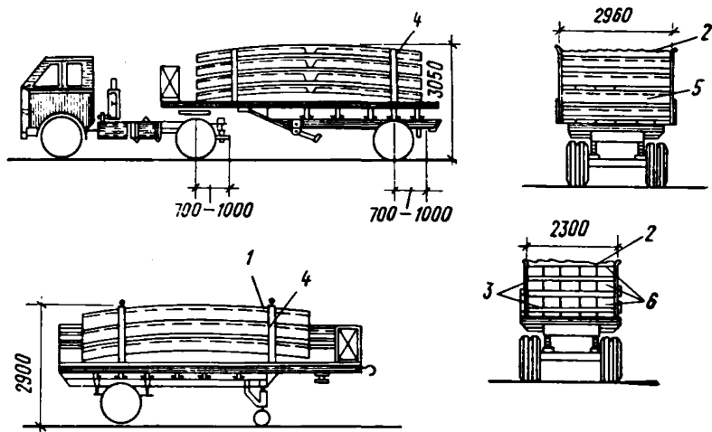
Рис. 49. Схема перевозки плит на полуприцепе МАЗ-5245
