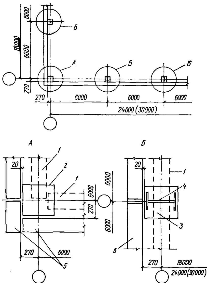
Рис. 32. Схема привязки основных и фахверковых колонн 1 — контурная балка; 2 — основная колонна; 3 — фахверковая колонна; 4 — металлический оголовок колонны; 5 — стеновые панели
