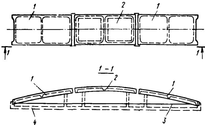
Рис. 52. Схема монтажного блока
