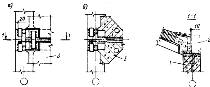
Рис. 24. Соединение плит по периметру здания
