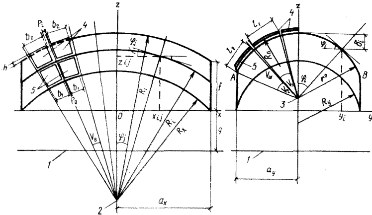
Рис. 53. Определение координат точек исходной поверхности 1 — плоскость отсчета; 2 — ось вращения тора; 3 — центр меридионального сечения тора; 4 — средние плиты; 5 — контурные плиты
