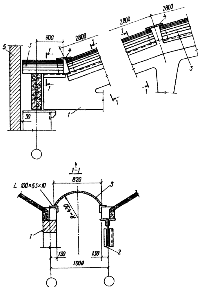
Рис. 31. Перекрытие температурных швов 1 — железобетонная ферма; 2 — стальная ферма; 3 — щит настила; 4 — нащельник из оцинкованной кровельной стали; 5 — стена
