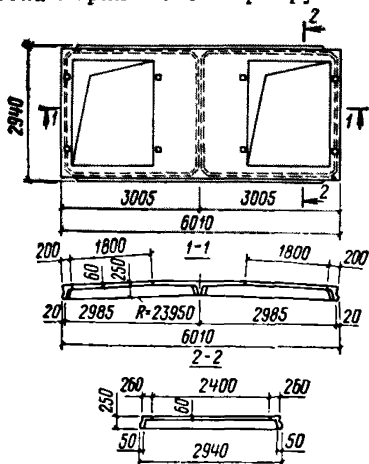
Рис. 9. Плита с проемами для зенитных фонарей (тип ПБ-6)
