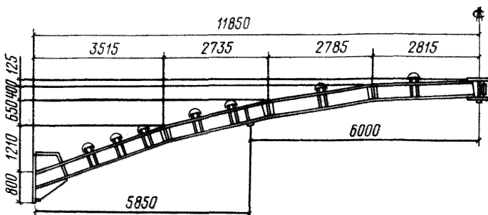
Рис. 20. Стальная контурная балка для пролета 24 м
