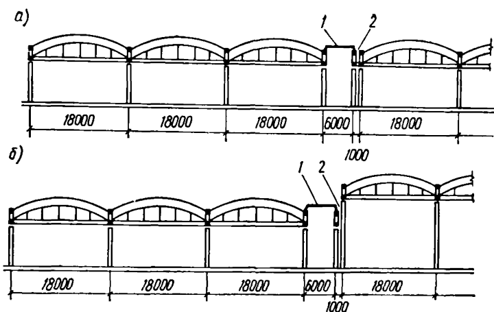
Рис. 30. Устройство плоских вставок в зданиях с оболочками а — в местах температурных швов; б — в местах перепадов высот; 1 — плоская вставка; 2 — деформационный шов
