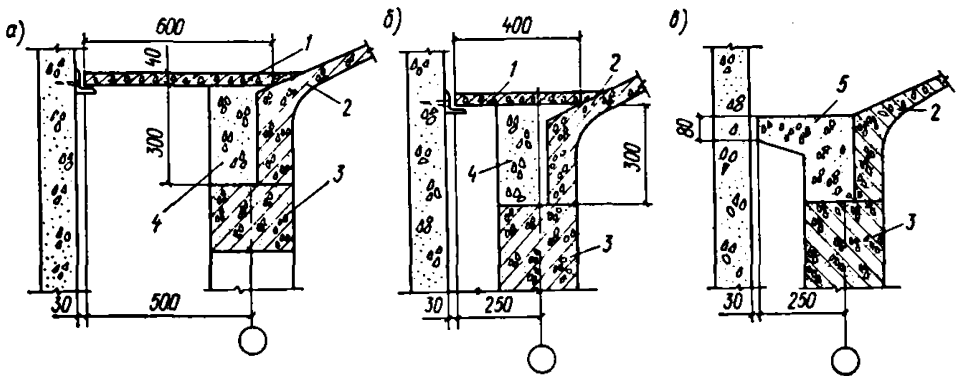
Рис. 36. Заделка зазоров между стеной и контурным элементом а — сборными плитами при привязке 500 мм; б — сборными плитами при привязке 250 мм; в — монолитным контурным швом; 1 — доборная плита по серии ПК-01-88; 2 — плита оболочки; 3 — контурный элемент; 4 — набетонка; 5 — монолитный шов
