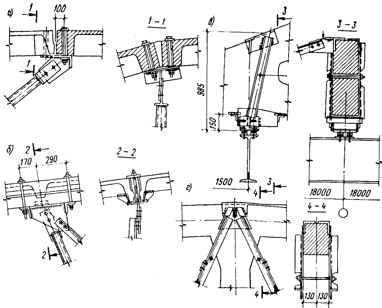
Рис. 47. Узлы крепления подвесных кранов
