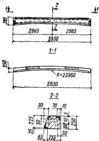
Рис. 7. Доборная средняя плита (тип ПБ-3)
