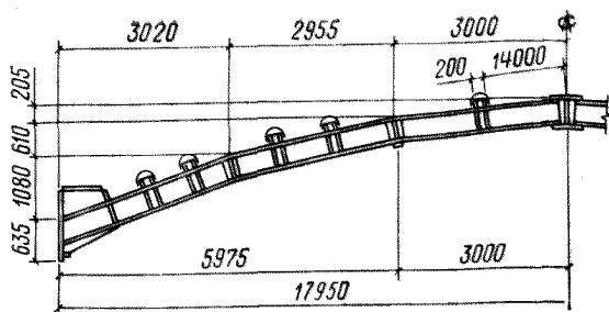
Рис. 19. Стальная контурная балка для пролета 18 м (тип БКМ-18)
