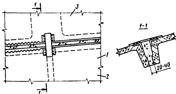
Рис. 23. Примыкание средних поперечных ребер основных и доборных плит 1 — средняя плита; 2 — контурная плита; 3 — доборная плита
