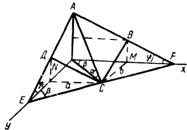
Рис. 55. Определение угла наибольшего ската поверхности
