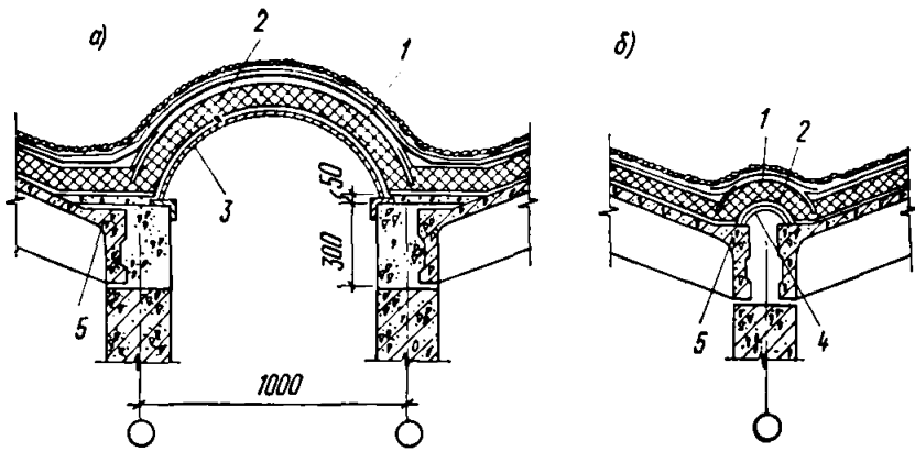
Рис. 38. Детали устройства
