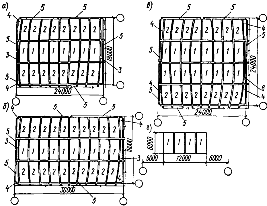
Рис. 4. Маркировочные схемы элементов
