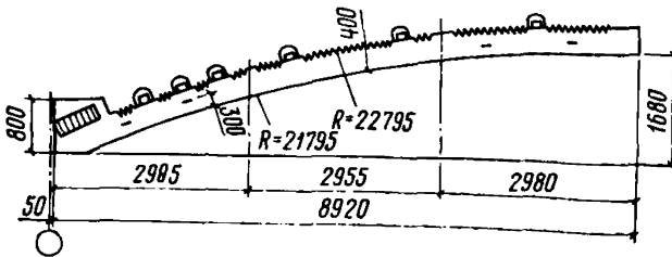
Рис. 13. Железобетонные контурные балки для пролета 18 м (тип БКБ-18)
