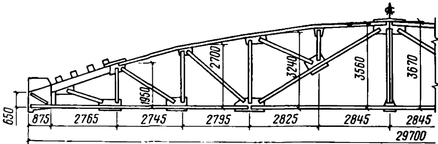
Рис. 17. Стальная контурная ферма пролетом 30 м (тип ФКМ-30)
