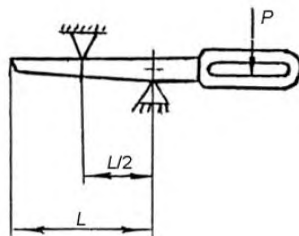
Рисунок 1 – Схема проверки прочности соединения пластмассовых ручек с лезвиями
