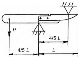
Рисунок 2 – Схема проверки прочности крепления накладных лезвий к корпусу
