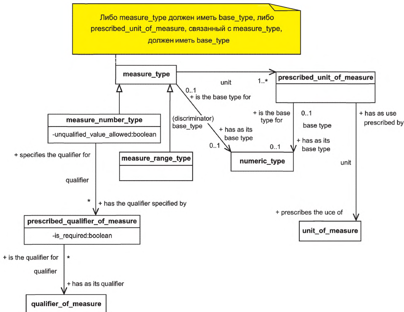
Рисунок 9 — Диаграмма класса UML для типов показателей
