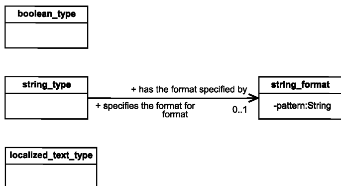
Рисунок 6 — Диаграмма класса UML для Булева и строковых типов данных
