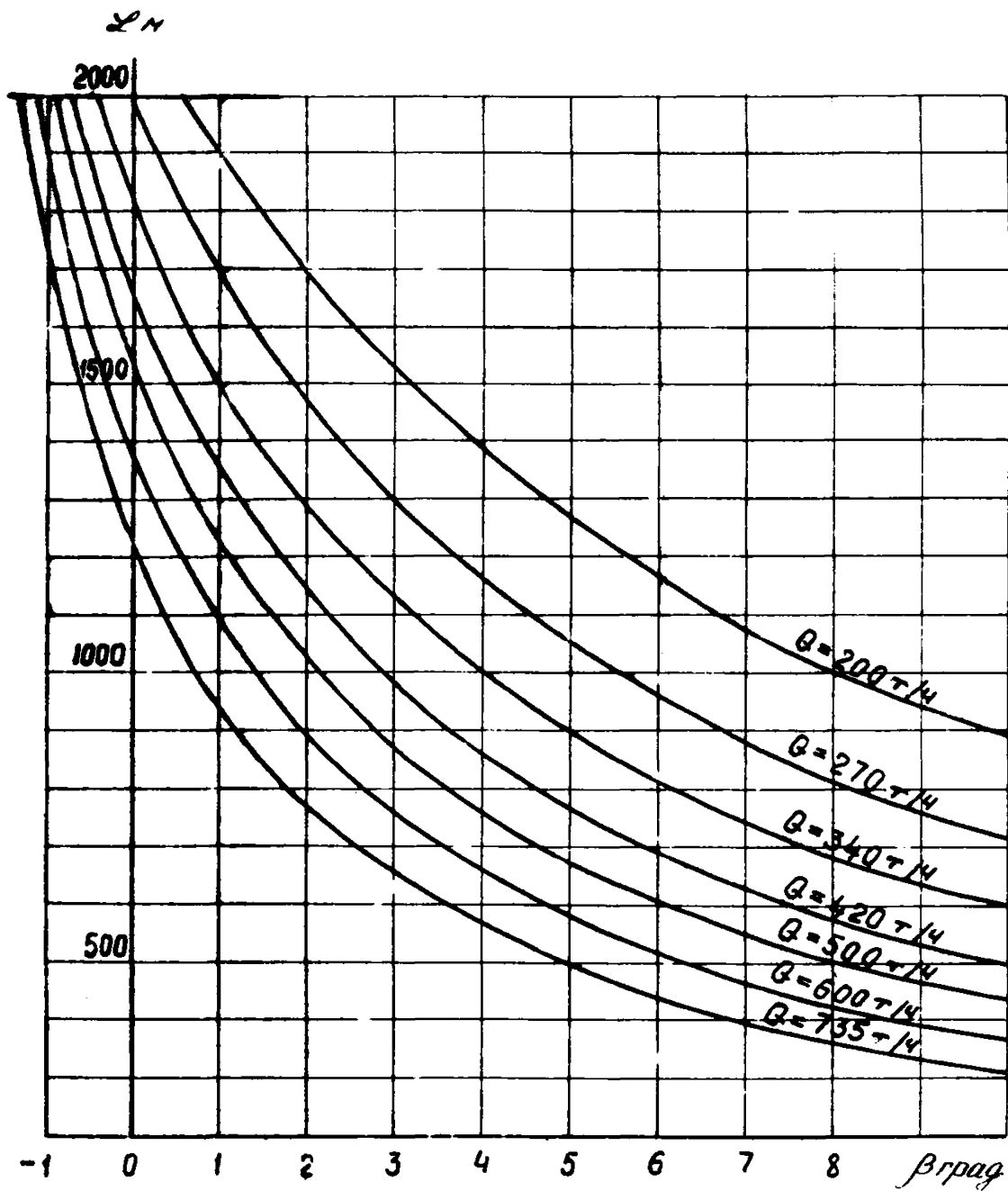
Рис. 19. Зависимость длины конвейера ДТ100 от угла наклона и производительности при V = 2,5 м/с и \rho = 200 кВт
