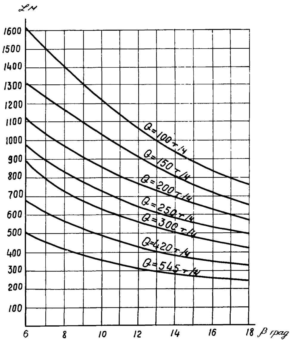
Рис. 13. Зависимость длины конвейера ШВ100 от угла наклона и производительности (резинотросовая лента)
