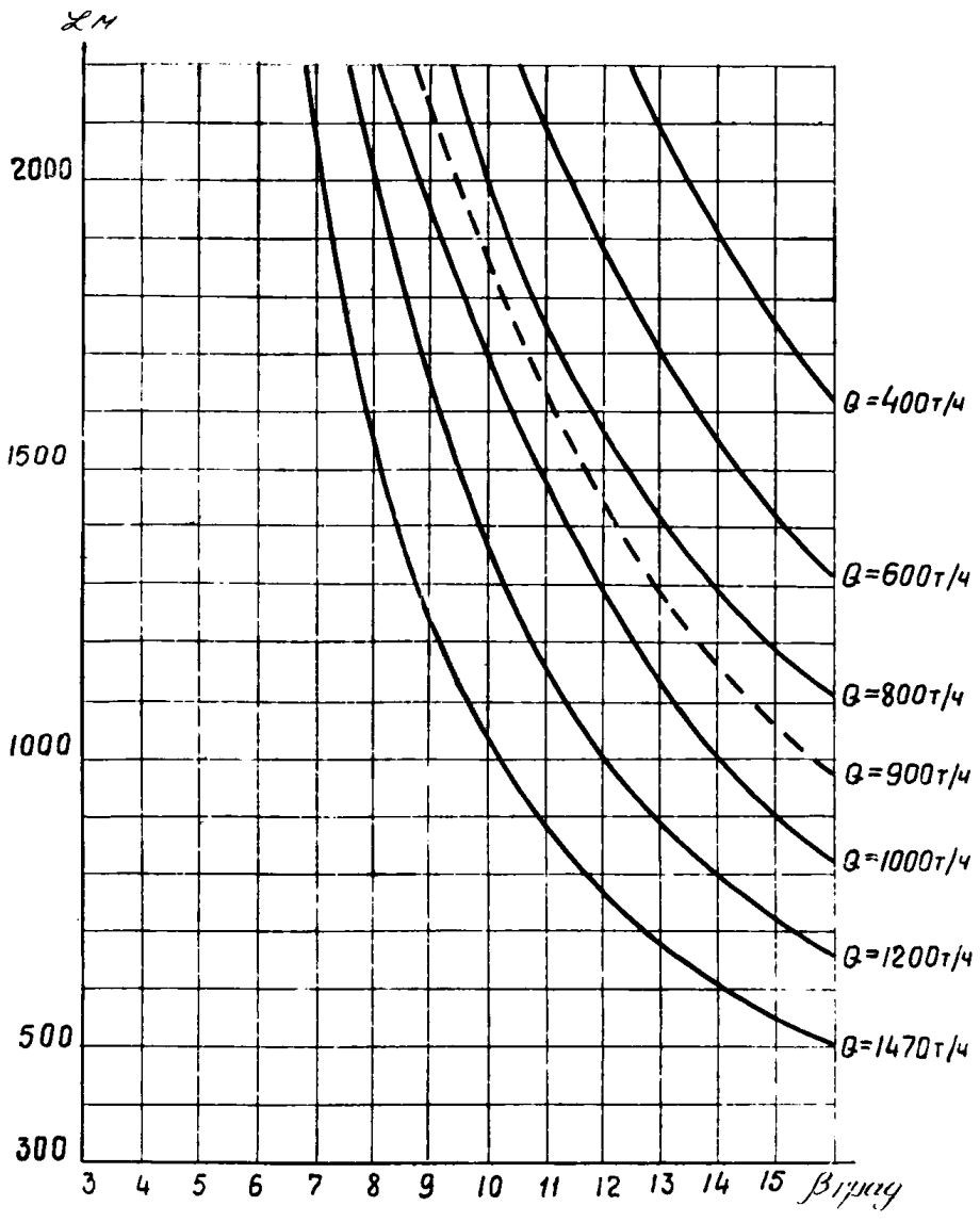
Рис. 28. Зависимость длины конвейера 2ЛБ120 от угла наклона и производительности
