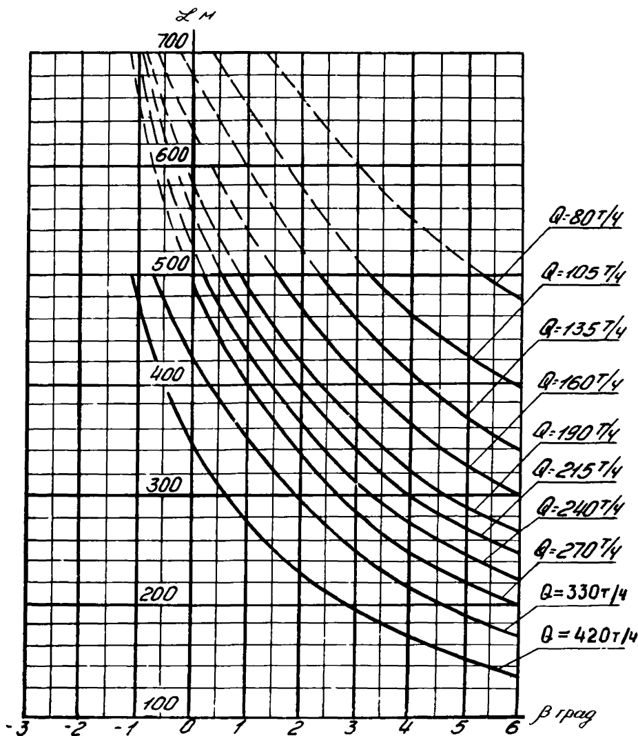
Рис. I. Зависимость длины конвейеров ЛЭ80 и ЛЛ80 от угла наклона и производительности:
