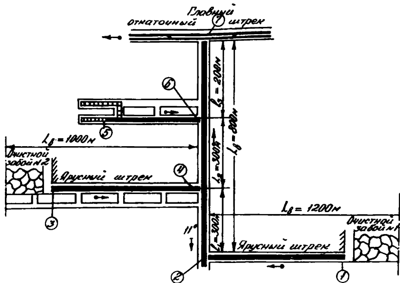
Рис. 3.3. Схемы участкового конвейерного транспорта угля от двух очистных и подготовительных забоев, расположенных на разных уровнях, при отработке длинных столов по простиранию:
