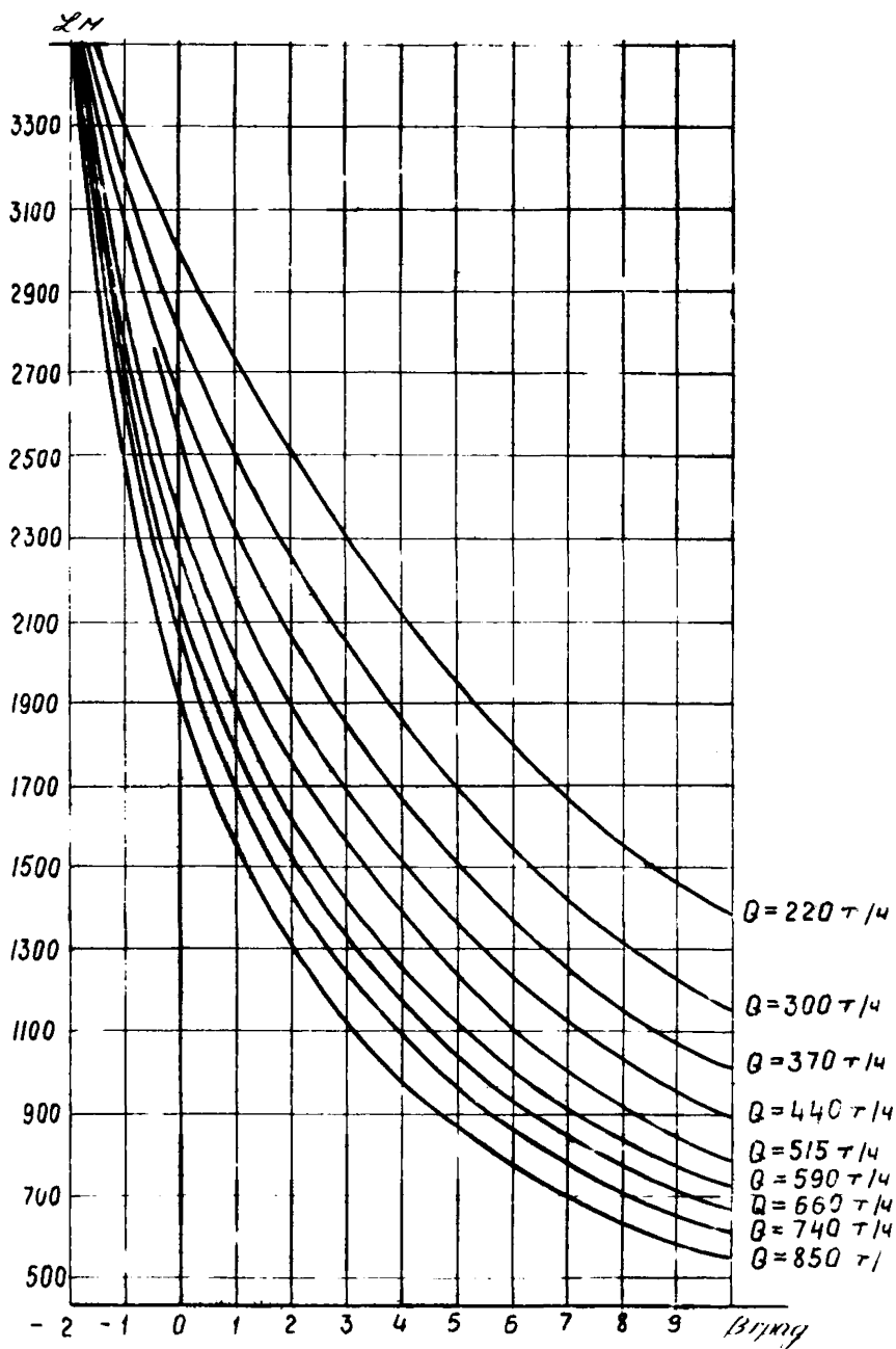
Рис. 22. Зависимость длины конвейера 2ЛТ100 от угла наклона в производительности
