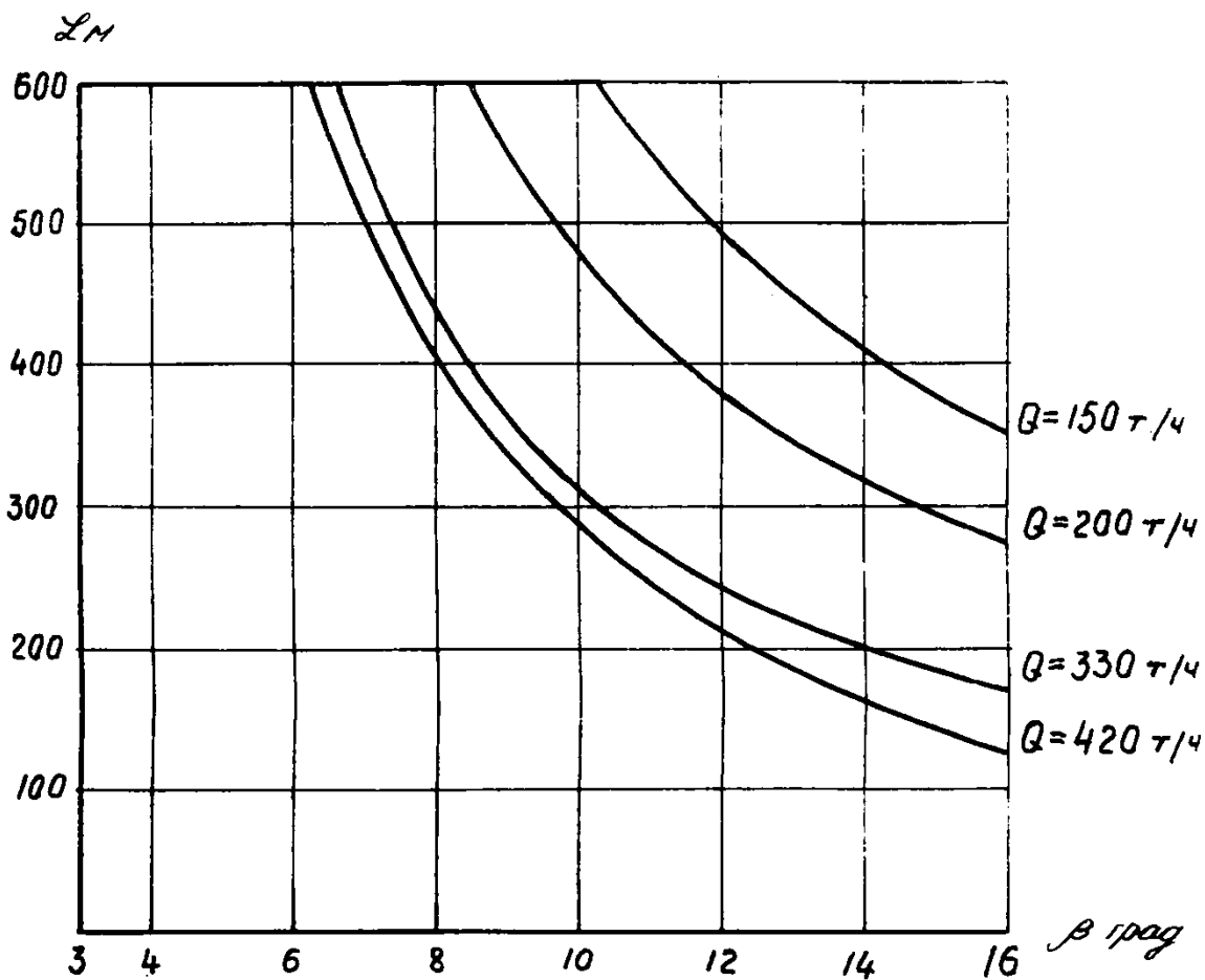
Рис. 3. Зависимость длины конвейера ЛБ80 от угла наклона и производительности:
