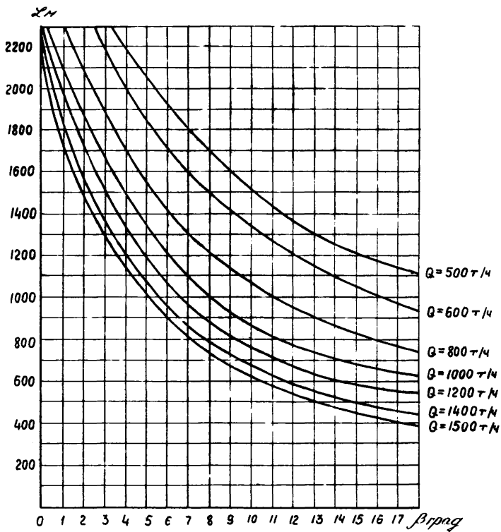
Рис. 26. Зависимость длины конвейеров 2ЛУ120А и 2ЛУ120В от угла наклона и производительности
