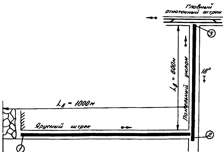
Рис. 2.3. Схемы участкового конвейерного транспорта угля от одного очистного забоя при отработке длинных столбов по пространству:
