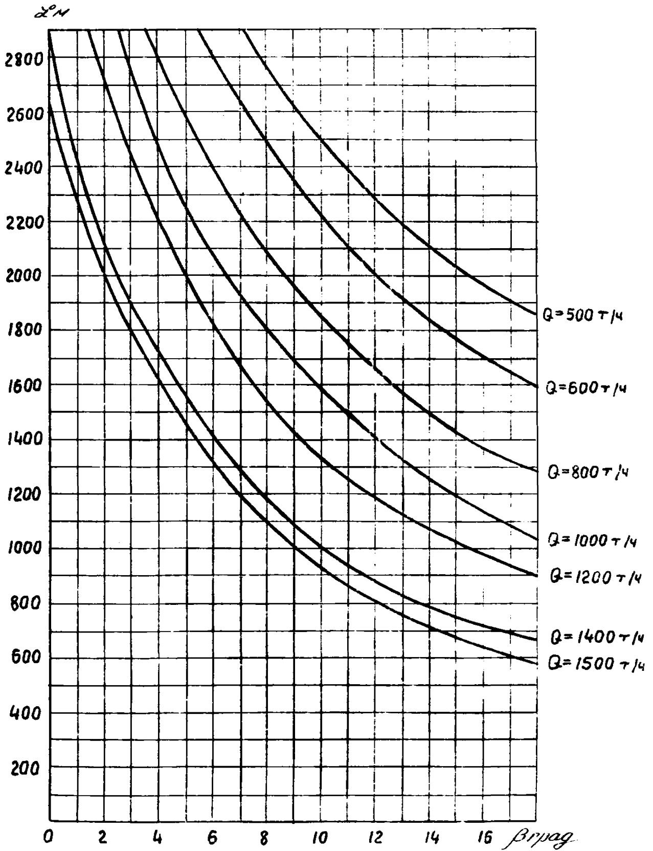
Рис. 27. Зависимость длины конвейера 2ЛУ1205 от угла наклона и производительности
