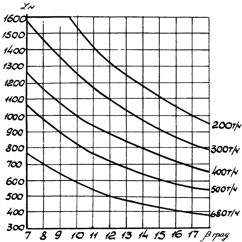
Рис. 24. Зависимость длины конвейера 2ЛУ100 от угла наклона и производительности
