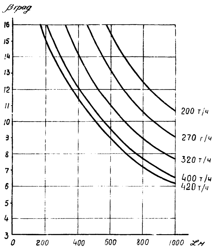
Рис. 9. Зависимость длины конвейера 21680 от угла наклона и производительности при V = 2,0 м/с и P = 80 кВт
