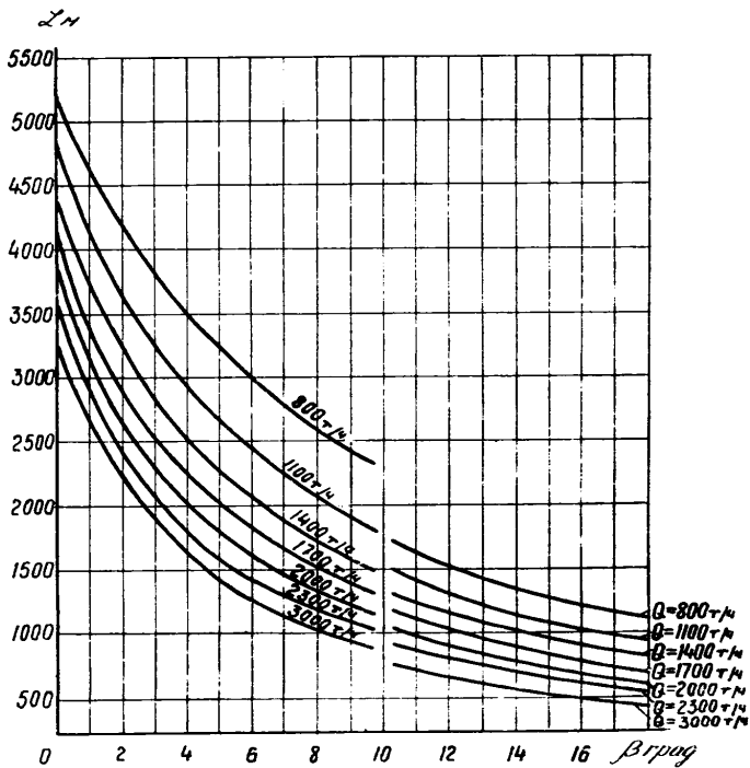
Рис. 31. Зависимость длины конвейера 2ДУ160 от угла наклона и производительности при \rho = 2000 кг/л
