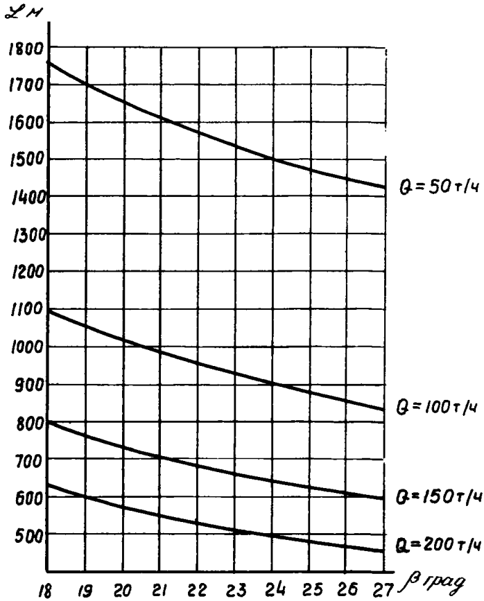
Рис. 10. Зависимость длины конвейера ЗЛН80 от угла наклона и производительности
