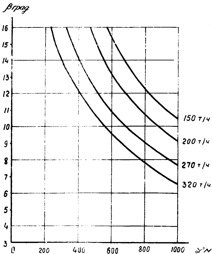
Рис. 8. Зависимость длины конвейера 2ЛБ80 от угла наклона и производительности при V = 1,6 м/с и D = 80 кВт
