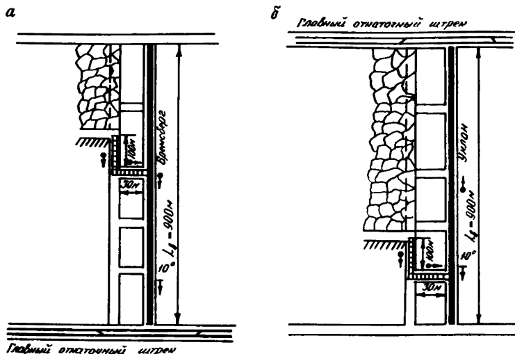
Рис. 2.2. Схемы участкового конвейерного транспорта угля от одного очистного забоя при отработке длинных столбов (с оставлением целиков) по падению (а) и восставию (б)
