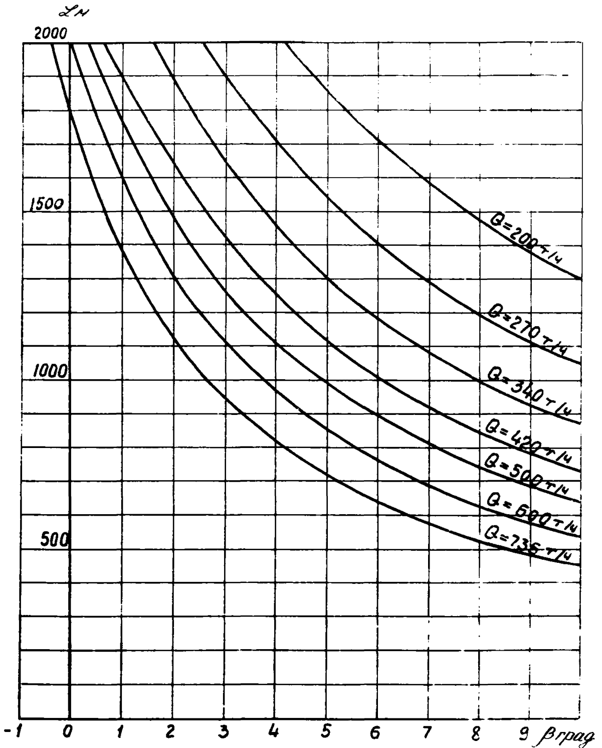
Рис. 22. Зависимость длины конвейера ЛТ100 от угла наклона и производительности при V = 2,5 \text{ м/с} и \rho = 300 \text{ кг}
