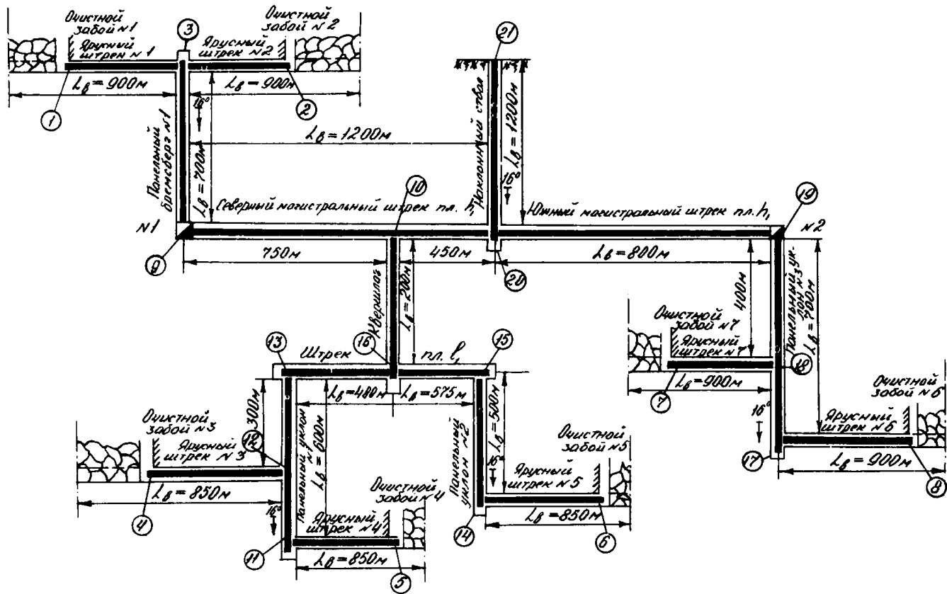
Рис. 4.2. Схема конвейерного транспорта угля шахты с семью очистными забоями
