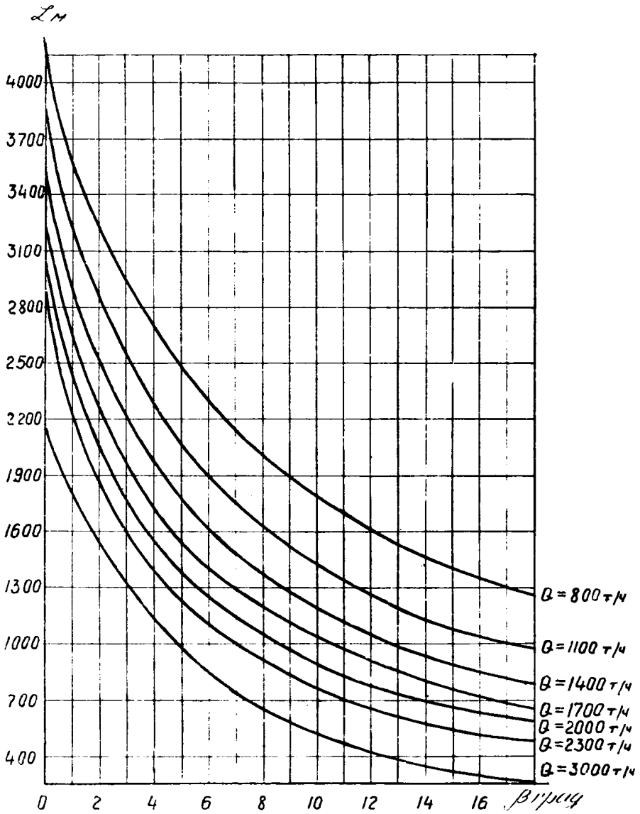
Рис. 30. Зависимость длины конвейера 2ЛУ160 от угла наклона и производительности при D = 1500 кВт
