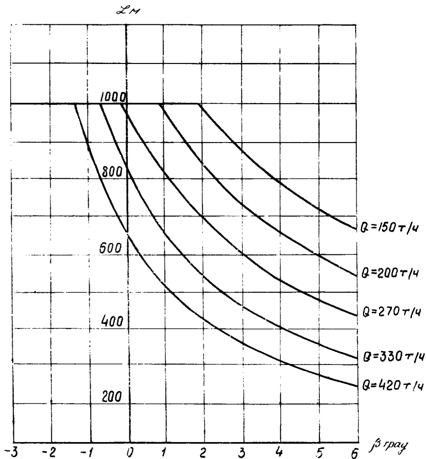
Рис. 4. Зависимость длины конвейеров 2ЛВ0 и 2ЛТ80 от угла наклона и производительности:
