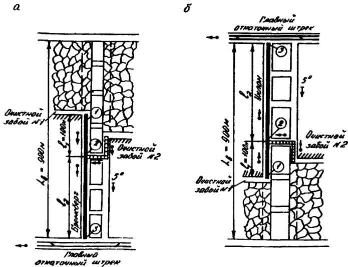
Рис. 3.1. Схемы участкового конвейерного транспорта угля от двоясных очистных забоев при отрастке длинных столбов по падению (а) и восставию (б)
