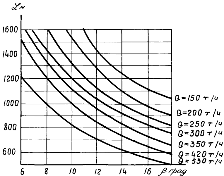
Рис. 16. Зависимость длины конвейера 2ЛЛ100 от угла наклона и производительности
