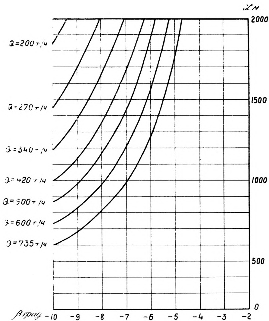
Рис. 2С. Зависимость длины конвейера ИЛТ100 от угла наклона и производительности при V = 2,5 \text{ м/с} и P = 200 \text{ кВт}
