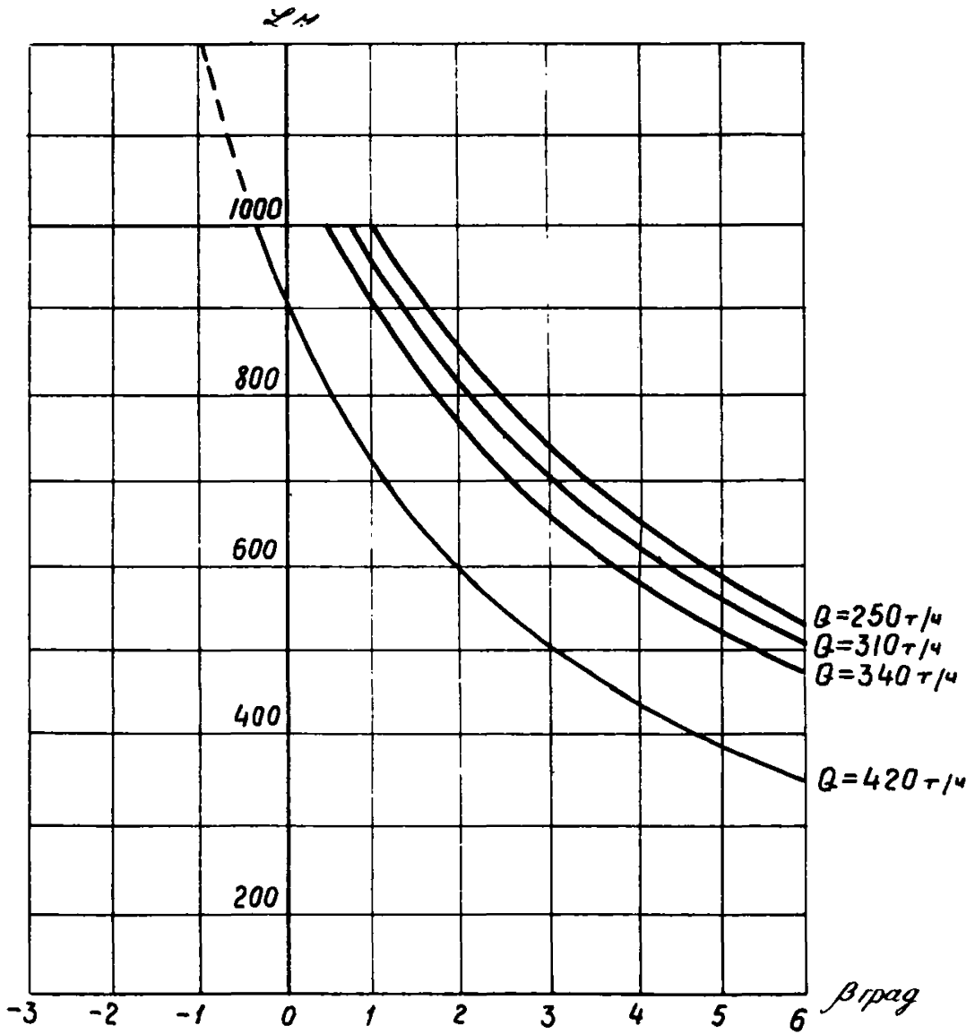
Рис. 7. Зависимость длины конвейеров 2Л80 и 2ЛТ80 от угла наклона и производительности при V = 2,0 м/с и P = 110 кВт
