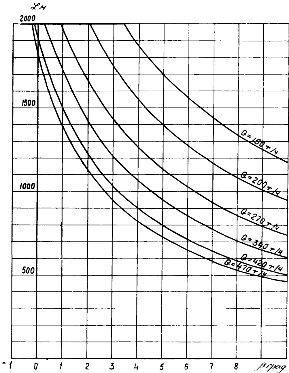
Рис. 17. Зависимость длины конвейера ЛТ100 от угла наклона и производительности при V = 1,6 м/с и \rho = 200 кВт
