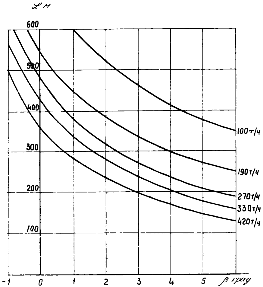
Рис. 2. Зависимость длины конвейеров ЛЛ80 и ЛЛТ80 от угла наклона и производительности при V = 2 м/с и P = 40 кВт
