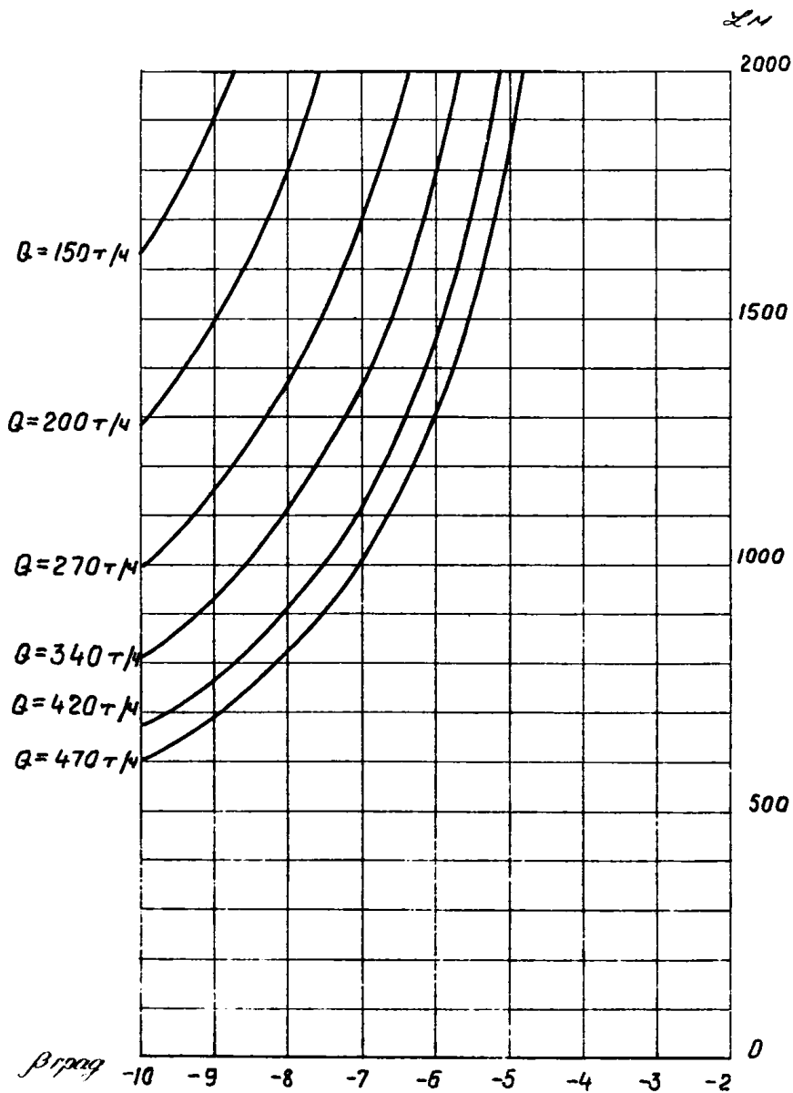
Рис. 18. Зависимость длины конвейера ЛТ100 от угла наклона и производительности при V = 1,6 \text{ м/с} и \rho = 200 \text{ кВт}
