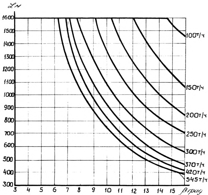
Рис. 15. Зависимость длины конвейера ЛБ100 от угла наклона и производительности
