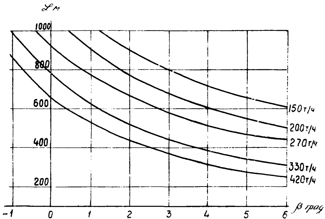
Рис. 5. Зависимость длины конвейеров 2Л80 и 2ЛТ80 от угла наклона и производительности при v = 2,0 м/с и \rho = 80 кВт
