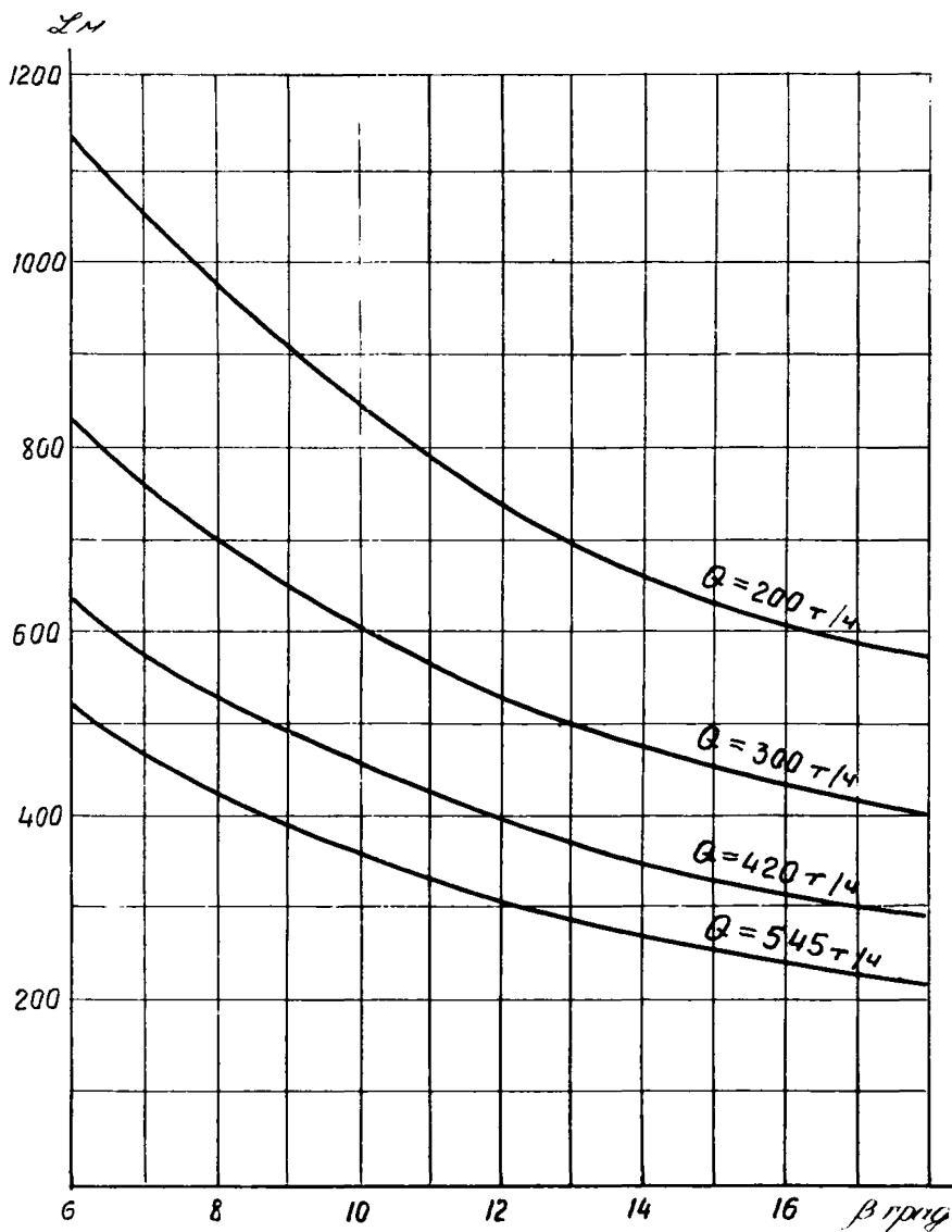
Рис. 14. Зависимость длины конвейера ЛЛУ100 от угла наклона и производительности (резинотканевая лента)
