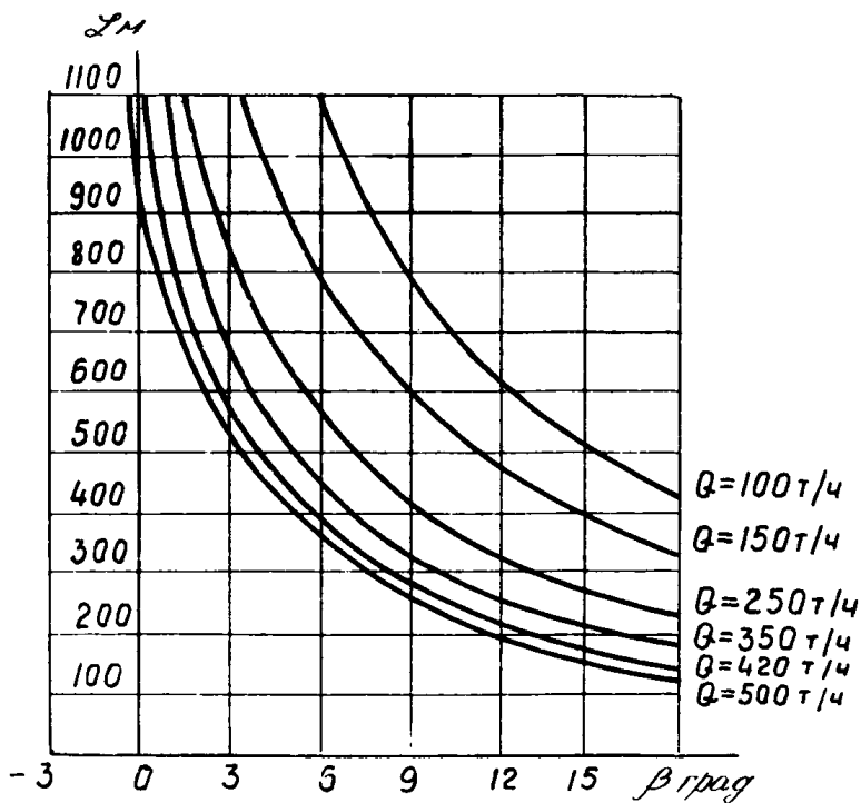
Рис. 12. Зависимость длины конвейера ЛЛЮОК от угла наклона и производительности
