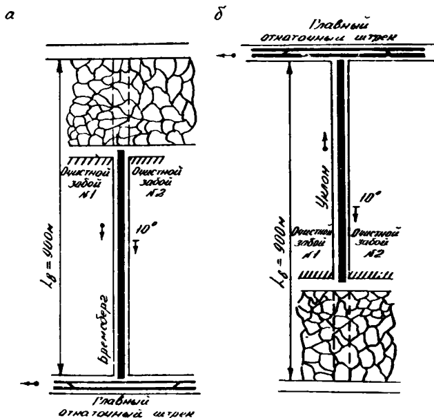
Рис. 2.5. Схемы участкового конвейерного транспорта угля от сперенных очистных забоев при отработке длинных столбов по падению (а) и восстанию (б)
