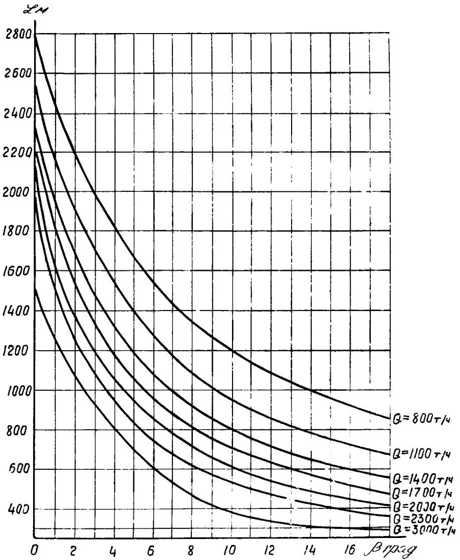
Рис. 29. Зависимость длины конвейера 2ЛУ160 от угла наклона и производительности при \rho = 1000 кг/м
