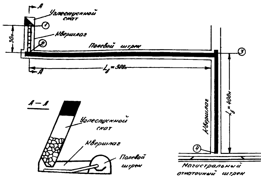
Рис. 2.4. Схема участкового транспорта угля от двух очистных забоев при разработке крутых пластов
