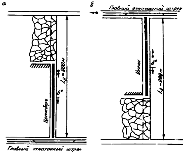
Рис. 2.1. Схемы участка конвейерного транспорта угля от одного очистного забоя при отработке длинных столбов (без оставления целиков) по падению (а) и восстанию (б)
