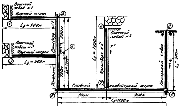
Рис. 4.1. Схема конвейерного транспорта угля шахты с тремя очистными забоями
