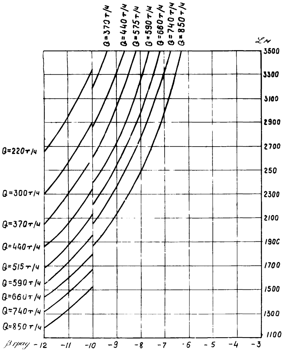
Рис. 23. Зависимость длины конвейера 2ЛТ100 от угла наклона и производительности
