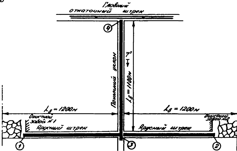
Рис. 3.2. Схемы участкового конвейерного транспорта угля от двух очистных забоев, расположенных на одном уровне, при отработке длинных столбов по простиранию:
