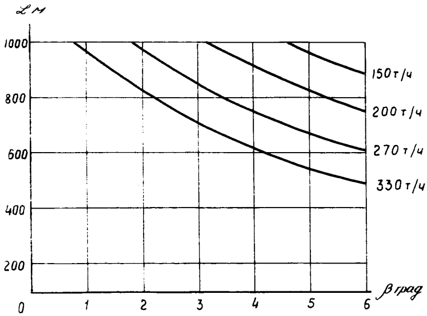
Рис. 6. Зависимость длины конвейеров 2Л80 и 2ЛТ80 от угла наклона и производительности при v = 1,6 м/с и P = 110 кВт
