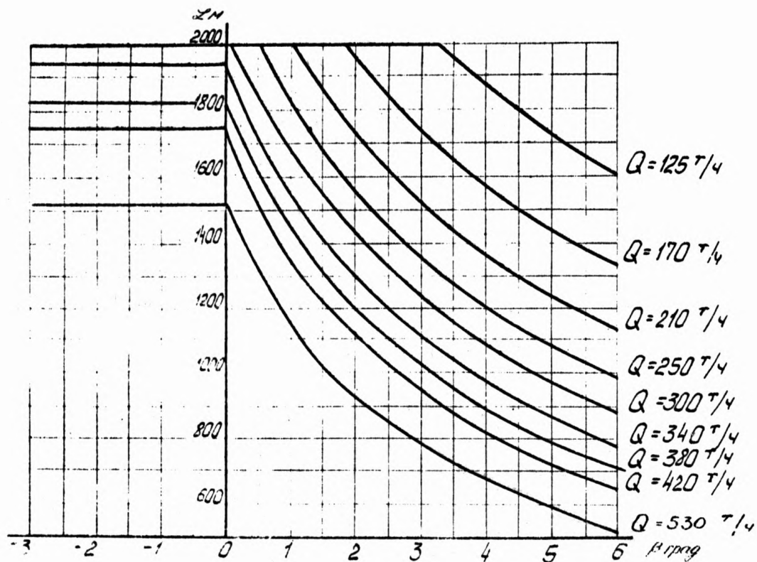
Рис. 11. Зависимость длины конвейера ИЛ100 от угла наклона и производительности
