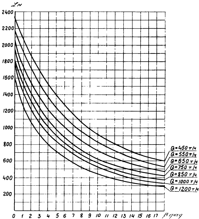
Рис. 25. Зависимость длины конвейера ЛЛУ120 от угла наклона и производительности
