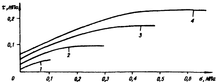
Рис. 3. Графики сопротивления сдвигу намынных пород при различных уплотняющих нагрузках ( \sigma_{упл} )
