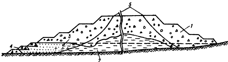
Рис. 19. Отвалообразование на гидротвалах с частичным и полным выдавливанием намывных пород из-под отвала:
