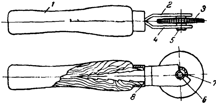
Рис. 49. Накаточный ролик:
