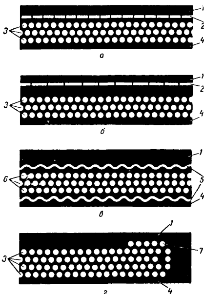
Рис. 1. Конструкции конвейерных лент:
