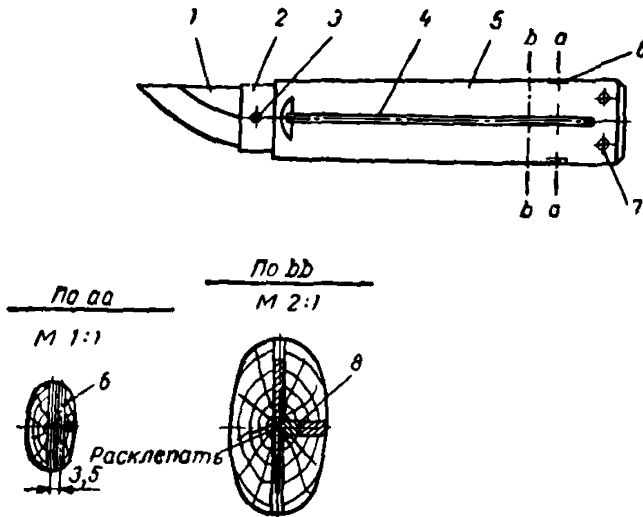
Рис. 50. Выдвижной нож:
