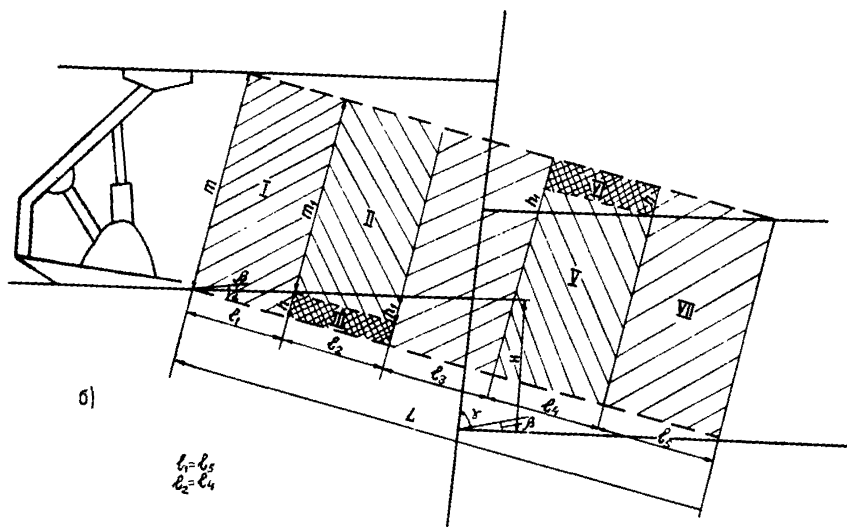
Рис. 8. Схемы для подсчета объема породы при переходе нарушения: а - при односторонней подрывке породы комбайном; б - при двухсторонней подрывке породы комбайном.
