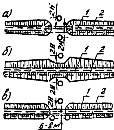
Рис. 1. Схемы расположения скважин в плане: а - при замене существующего моста трубой при проектировании второго пути; б - при удлинении трубы, лотка; в - в случае пристройки второго моста под второй путь; 1, 2 - оси первого (существующего) и второго (пристраиваемого) пути; H - высота насыпи; О - скважины
