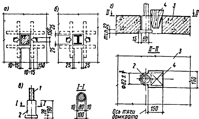
Рис. 7. Величины зазоров между воротниками и колоннами и размеры отверстий в плитах перекрытий для крепления грузовых тег подъемников
