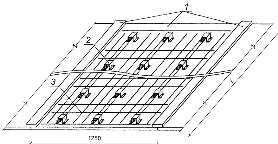
1 — блок несъемной опалубки из ЦПО; 2 — скоба; 3 — арматура; L — пролет перекрытия Рисунок 5.4 — Объемно-щитовой блок несъемной опалубки плиты перекрытия из ЦСП
