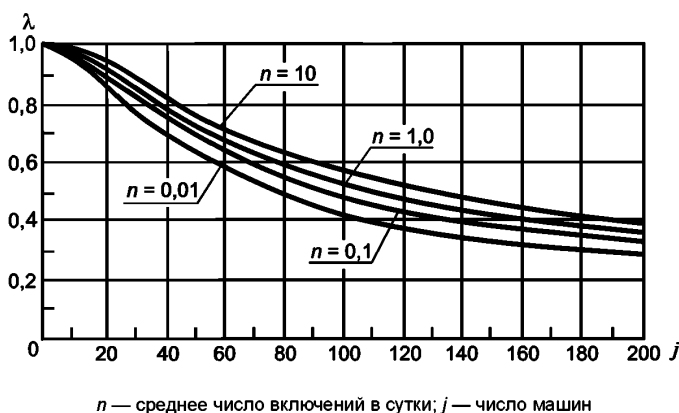
Рисунок 4.2 — График для определения коэффициента синфазности \lambda для машин и установок с синхронными двигателями
