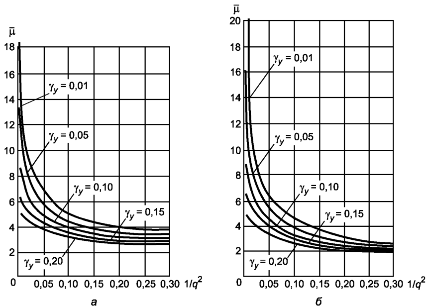
Рисунок 4.3 — Графики для определения коэффициента передачи \bar{\mu} при переходе через резонанс
