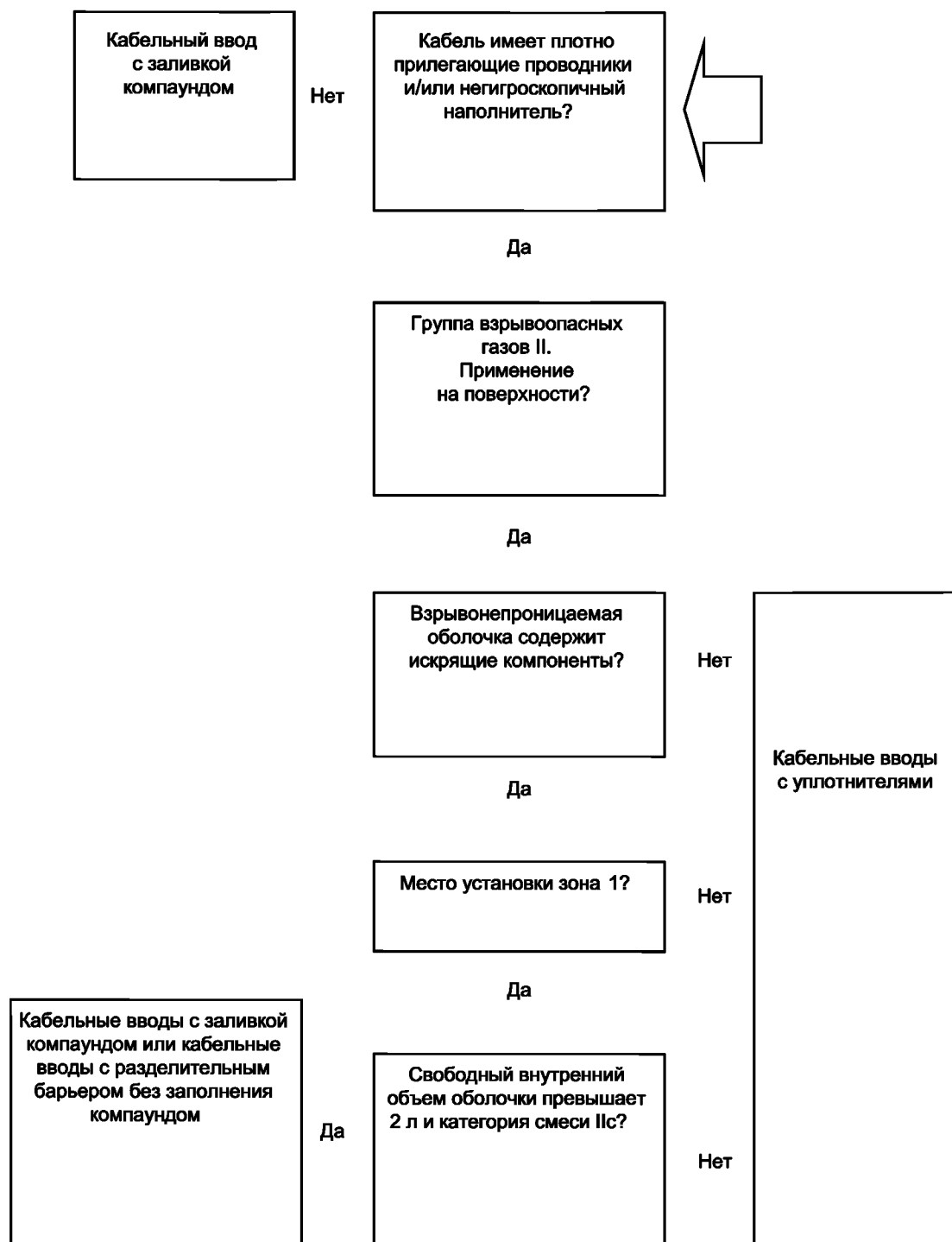
Рисунок 10.1 — Схема выбора кабельного ввода для оболочки Ex d
