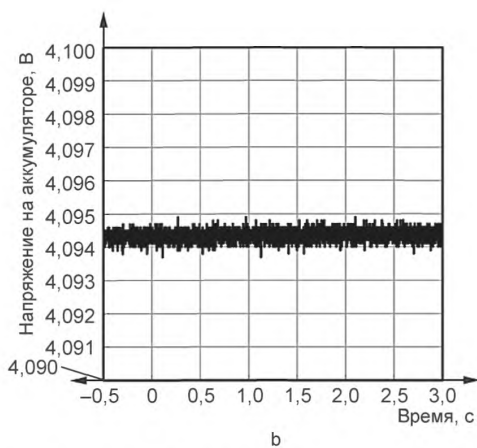
Рисунок А.32 — Напряжение в ходе испытания 14-4
