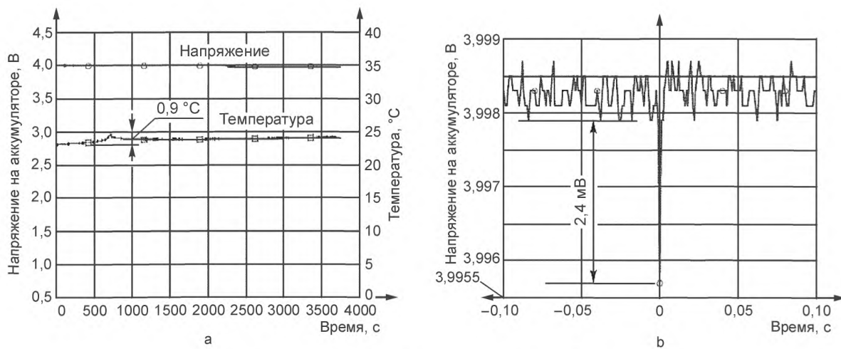
Рисунок А.10 — Напряжение и температура в ходе испытания 4
