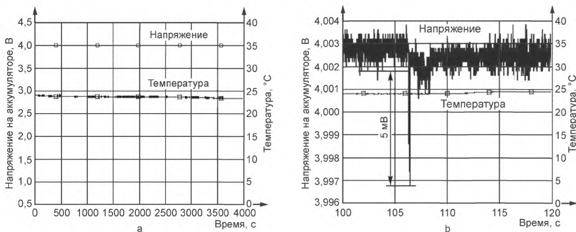
Рисунок А.1 — Напряжение и температура в ходе испытания 1-1 1)
