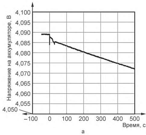
Рисунок А.26 — Напряжение в ходе испытания 12-6
