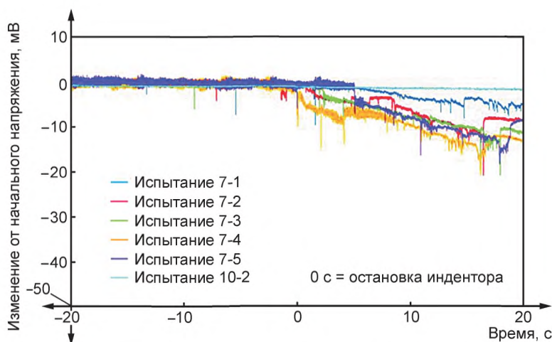
Рисунок А.14 — Напряжение в ходе испытания 7
