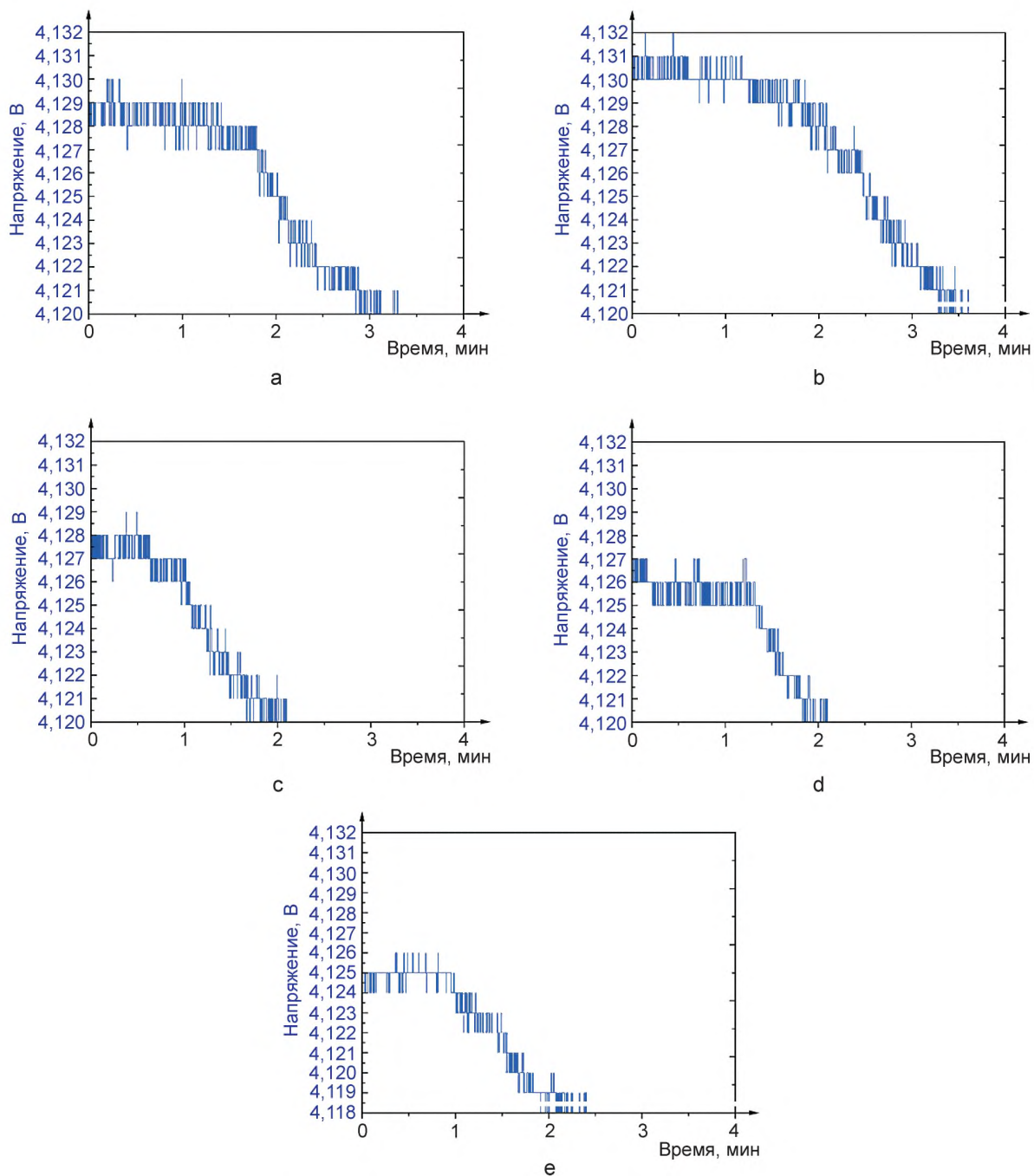
Рисунок А.35 — Напряжение в ходе испытания 16
