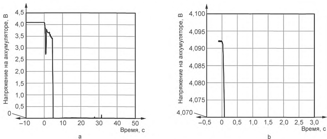
Рисунок А.29 — Напряжение в ходе испытания 14-1
