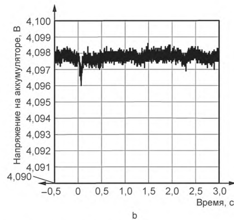
Рисунок А.33 — Напряжение в ходе испытания 14-5
