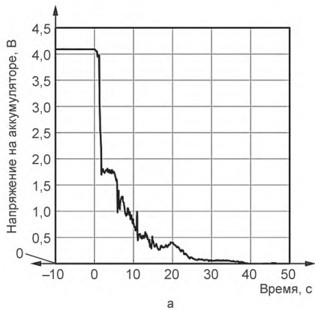
Рисунок А.27 — Напряжение в ходе испытания 12-7
