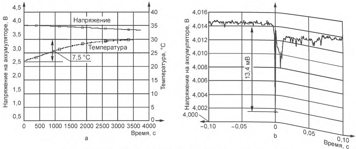
Рисунок А.11 — Напряжение и температура в ходе испытания 5-1
