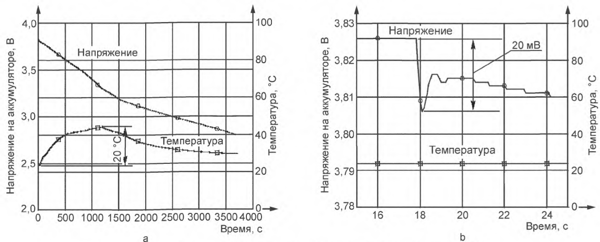
Рисунок А.7 — Напряжение и температура в ходе испытания 3-1
