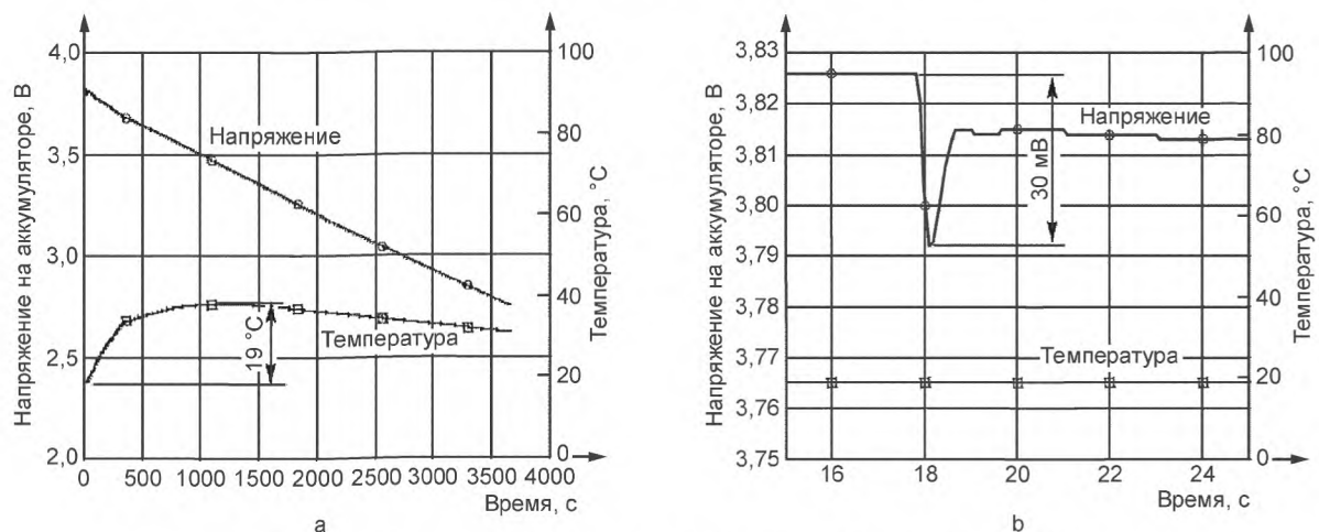
Рисунок А.8 — Напряжение и температура в ходе испытания 3-2
