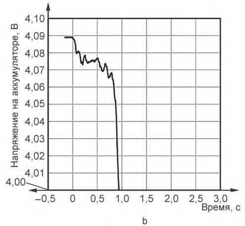
Рисунок А.25 — Напряжение в ходе испытания 12-5
