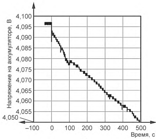
Рисунок А.23 — Напряжение в ходе испытания 12-3
