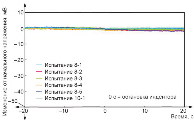
Рисунок А.15 — Напряжение в ходе испытания 8
