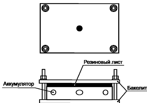
Рисунок 2 — Пример испытательной установки 2
