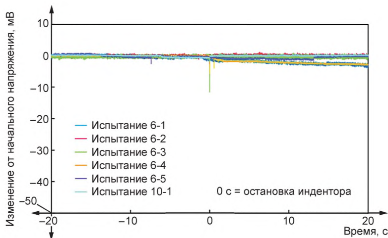
Рисунок А.13 — Напряжение в ходе испытания 6
