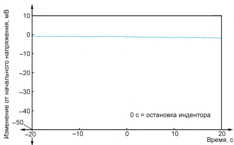
Рисунок А.18 — Напряжение в ходе испытания 10-2
