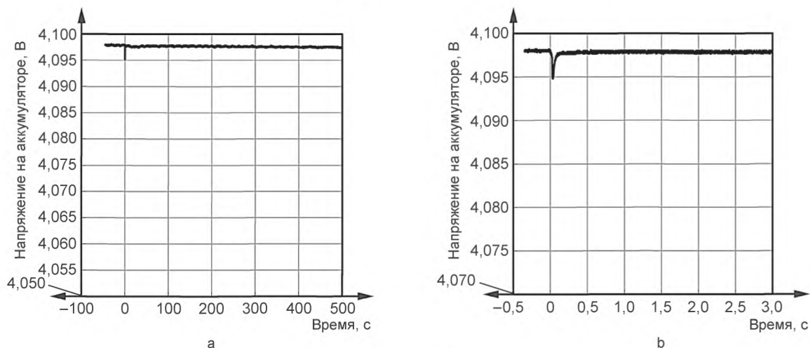
Рисунок А.19 — Напряжение в ходе испытания 11-1
