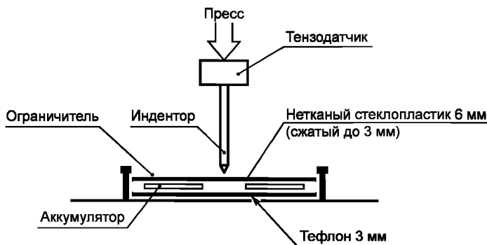
Рисунок 1 — Пример испытательной установки 1
