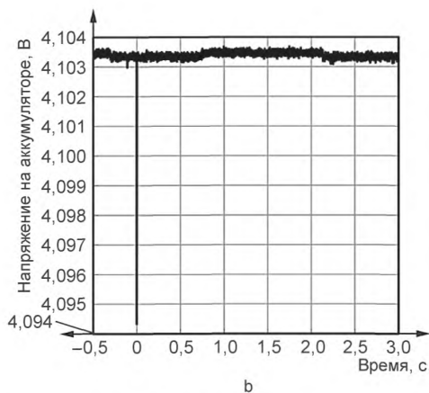
Рисунок А.31 — Напряжение в ходе испытания 14-3
