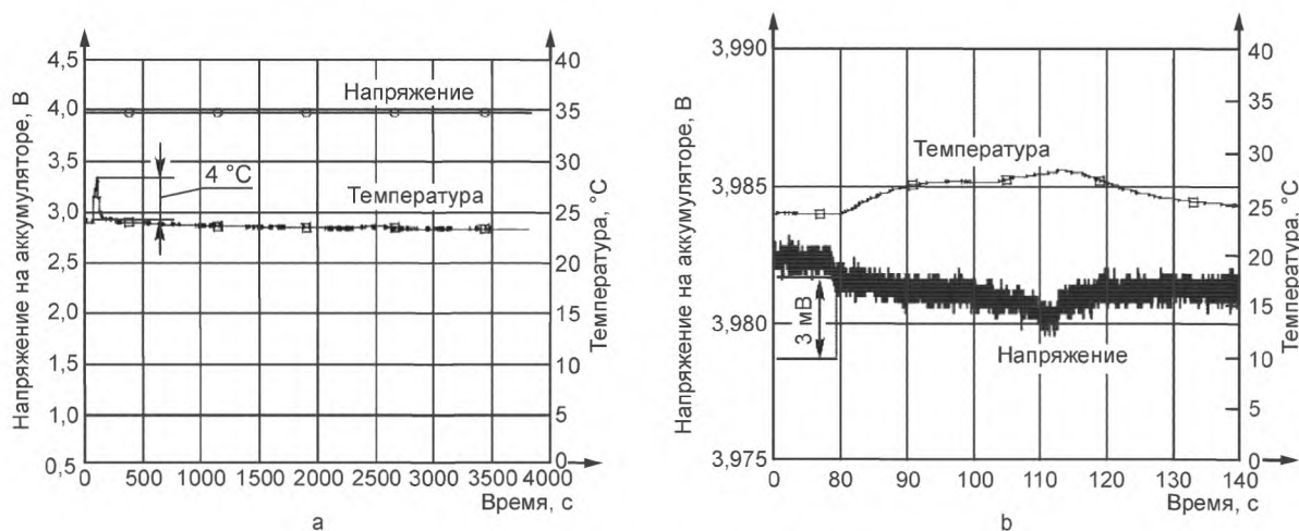
Рисунок А.2 — Напряжение и температура в ходе испытания 1-2
