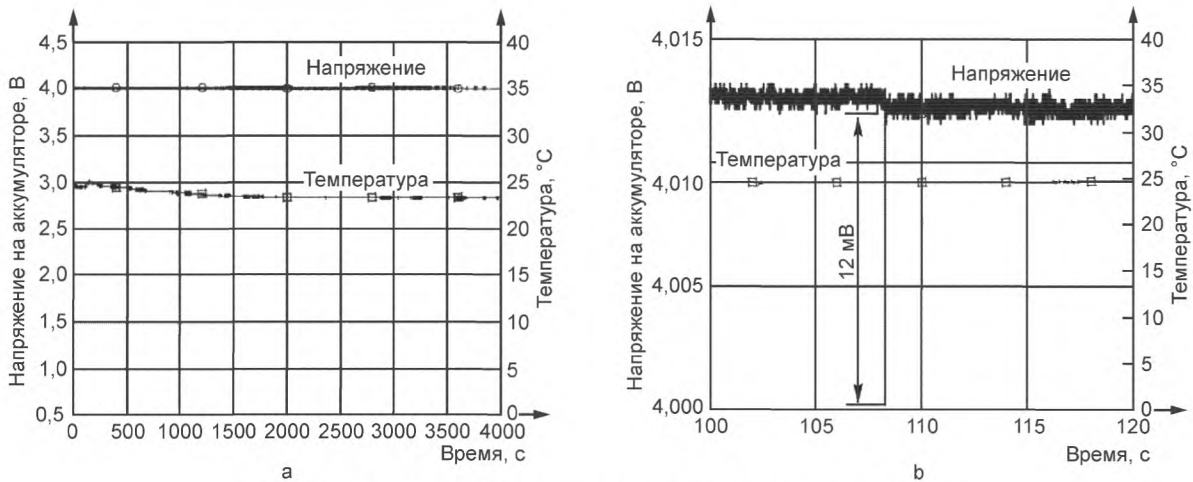
Рисунок А.3 — Напряжение и температура в ходе испытания 1-3
