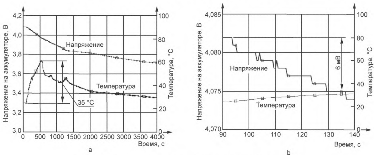
Рисунок А.5 — Напряжение и температура в ходе испытания 2-2
