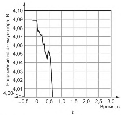
Рисунок А.27 — Напряжение в ходе испытания 12-7
