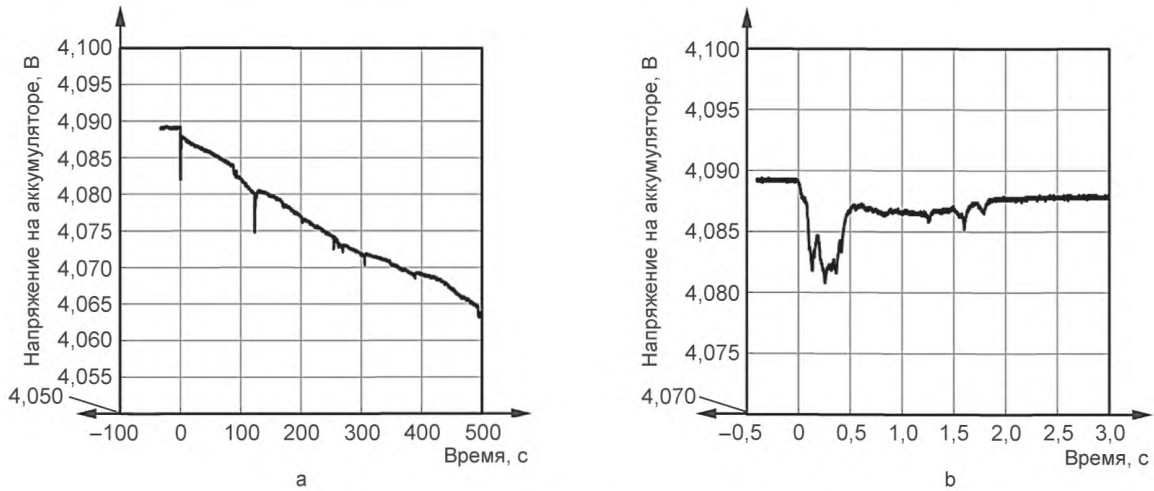
Рисунок А.21 — Напряжение в ходе испытания 12-1
