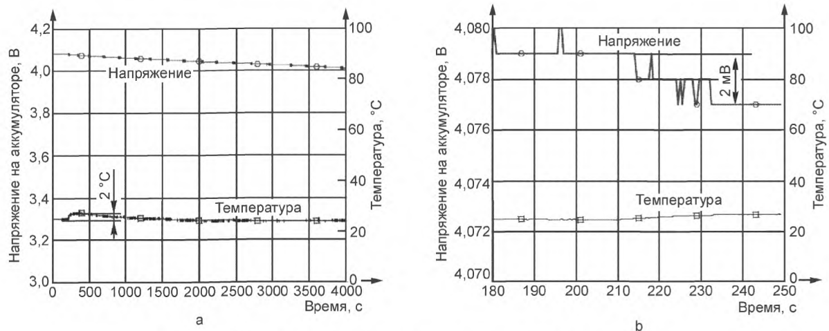
Рисунок А.6 — Напряжение и температура в ходе испытания 2-3
