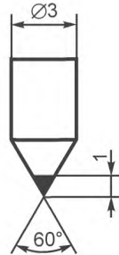
Рисунок А.9 — Керамический гвоздь диаметром 3 мм с наконечником из Ni
