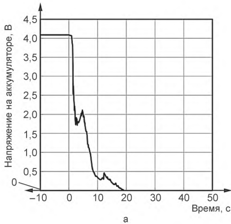
Рисунок А.25 — Напряжение в ходе испытания 12-5
