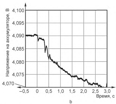
Рисунок А.28 — Напряжение в ходе испытания 13
