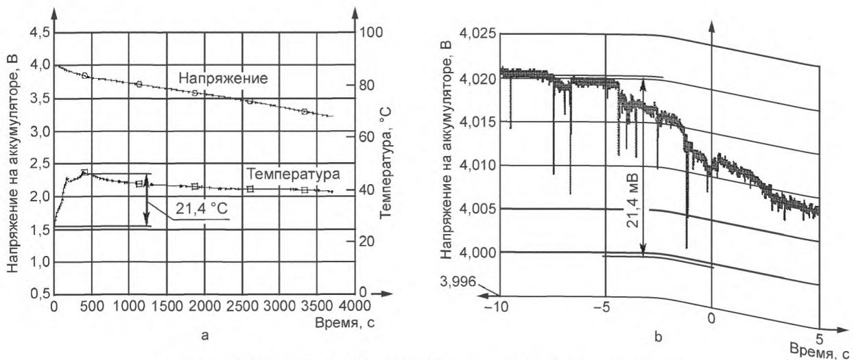
Рисунок А.12 — Напряжение и температура в ходе испытания 5-2
