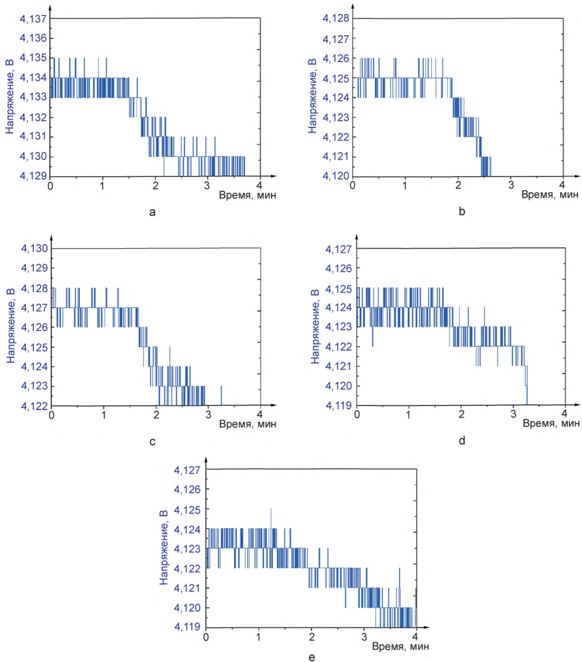
Рисунок А.34 — Напряжение в ходе испытания 15
