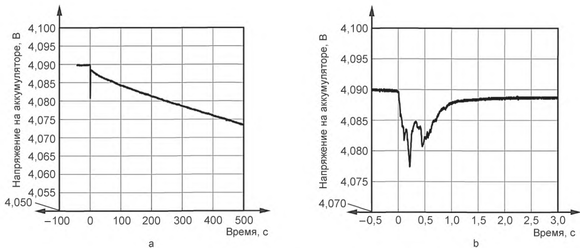
Рисунок А.22 — Напряжение в ходе испытания 12-2
