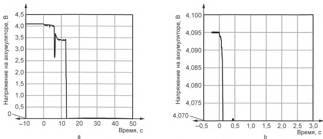
Рисунок А.30 — Напряжение в ходе испытания 14-2
