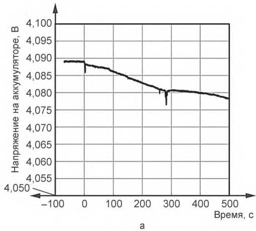
Рисунок А.24 — Напряжение в ходе испытания 12-4
