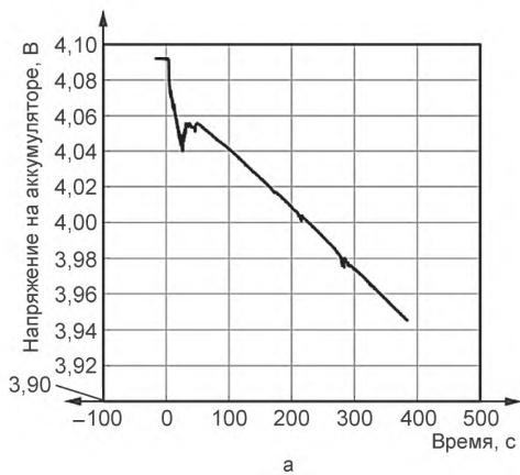
Рисунок А.28 — Напряжение в ходе испытания 13
