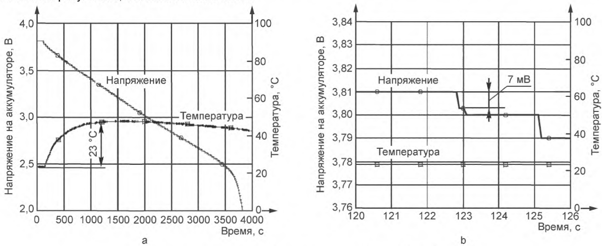
Рисунок А.4 — Напряжение и температура в ходе испытания 2-1
