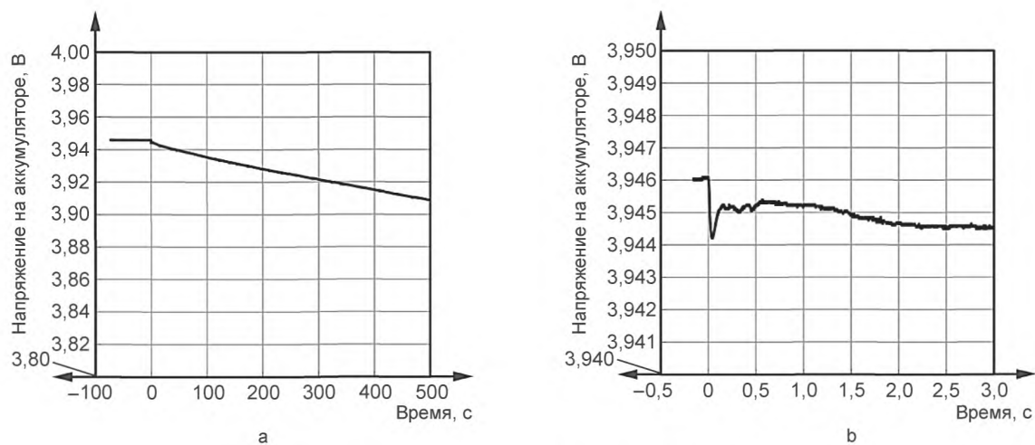
Рисунок А.20 — Напряжение в ходе испытания 11-2
