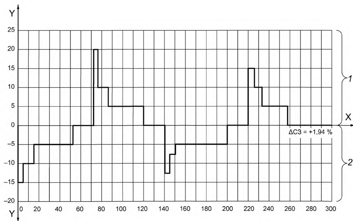
Рисунок 7 — Профиль величины тока испытаний по определению долговечности при циклировании — профиль с преобладанием заряда
